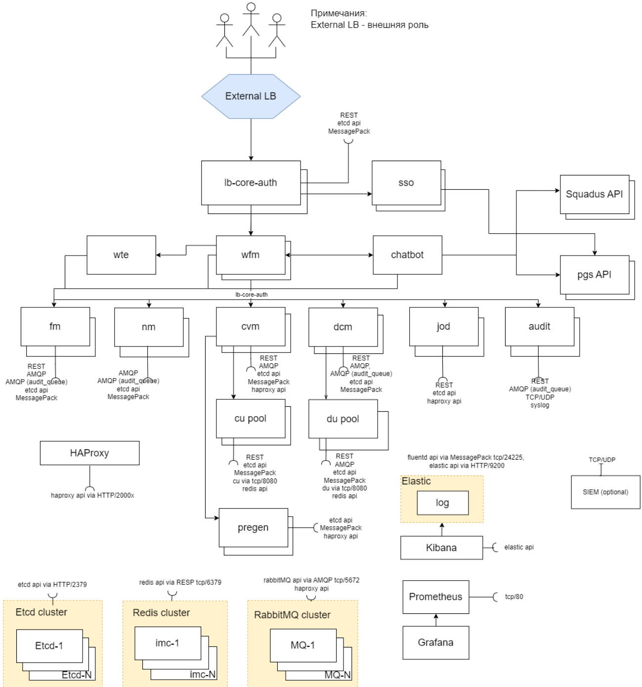
Рисунок 2 — Архитектурная схема Сервера совместного редактирования (СО)
