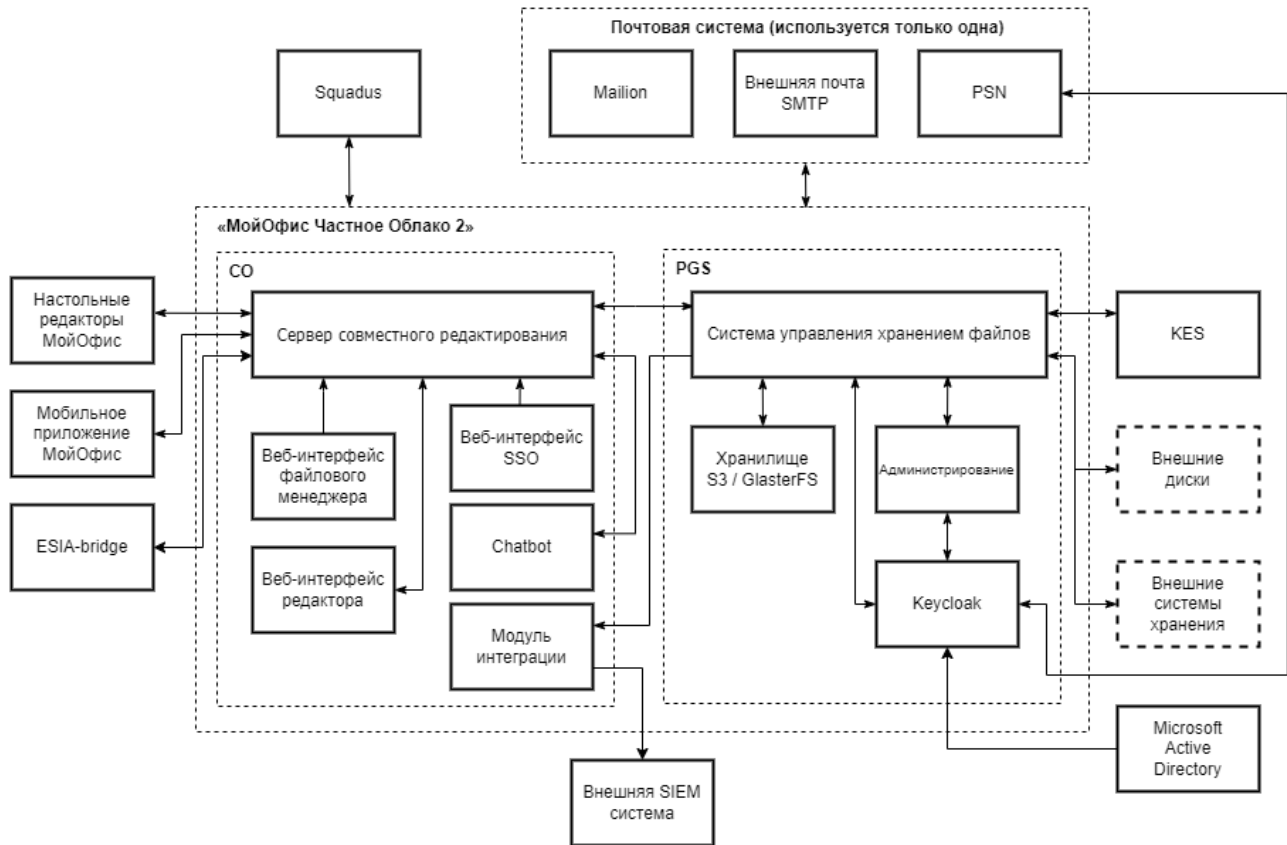
Рисунок 1 — Общая компонентная схема «МойОфис Частное Облако 2»
