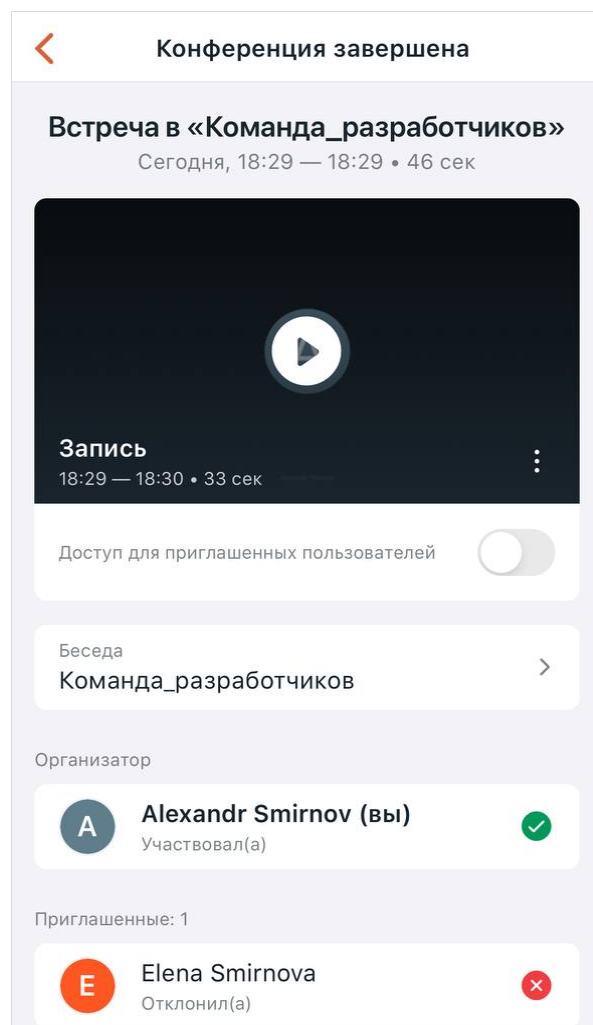
Рисунок 149 — Элементы управления записью у организатора и модераторов
