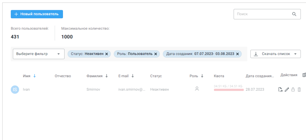
Рисунок 22 – Фильтрация пользователей
