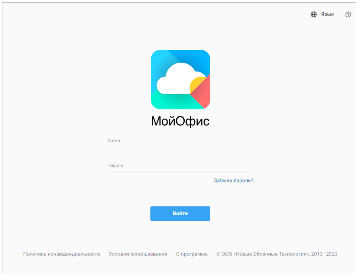
Рисунок 2 — Стартовая страница
