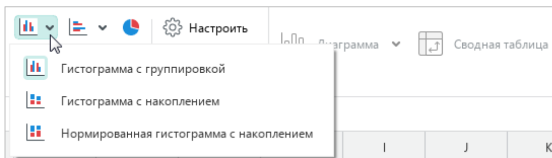
Рисунок 66 – Гистограмма
