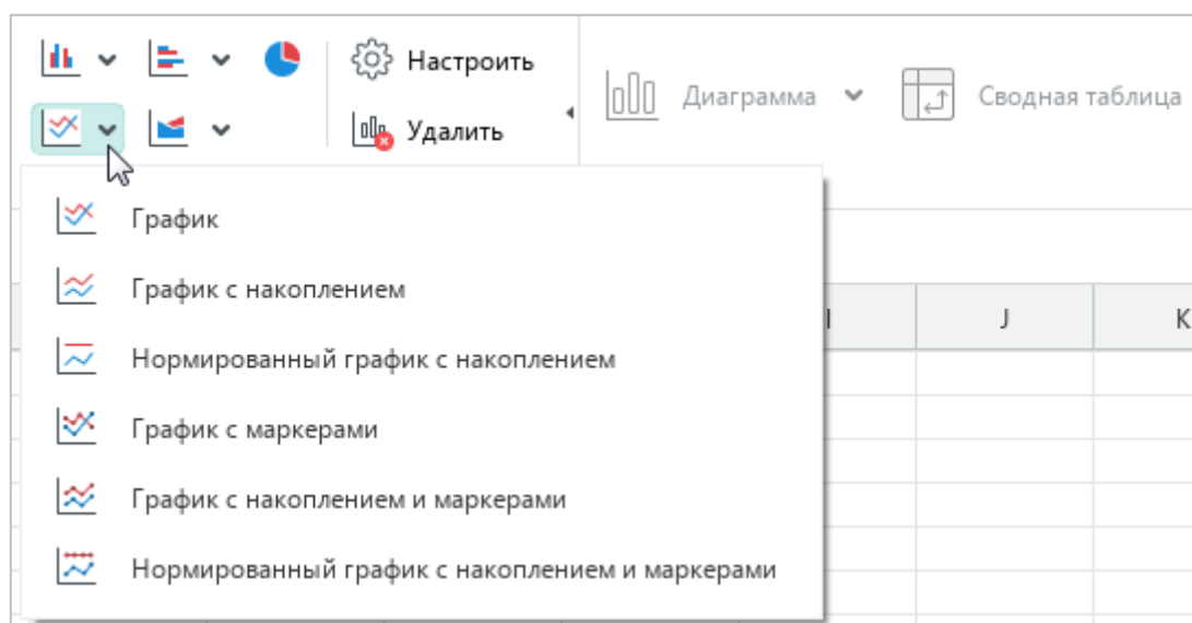
Рисунок 68 – График
