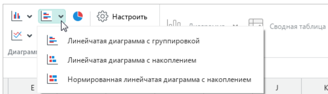
Рисунок 67 – Линейчатая диаграмма
