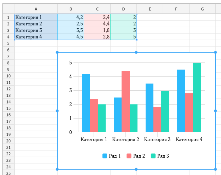
Рисунок 284 – Диаграмма
