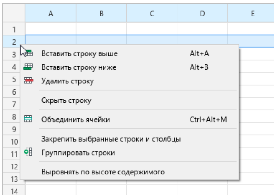
Рисунок 123 – Контекстное меню строки
