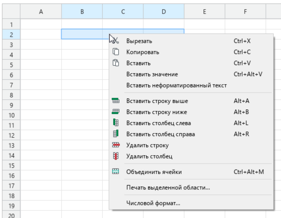
Рисунок 119 – Контекстное меню ячейки
