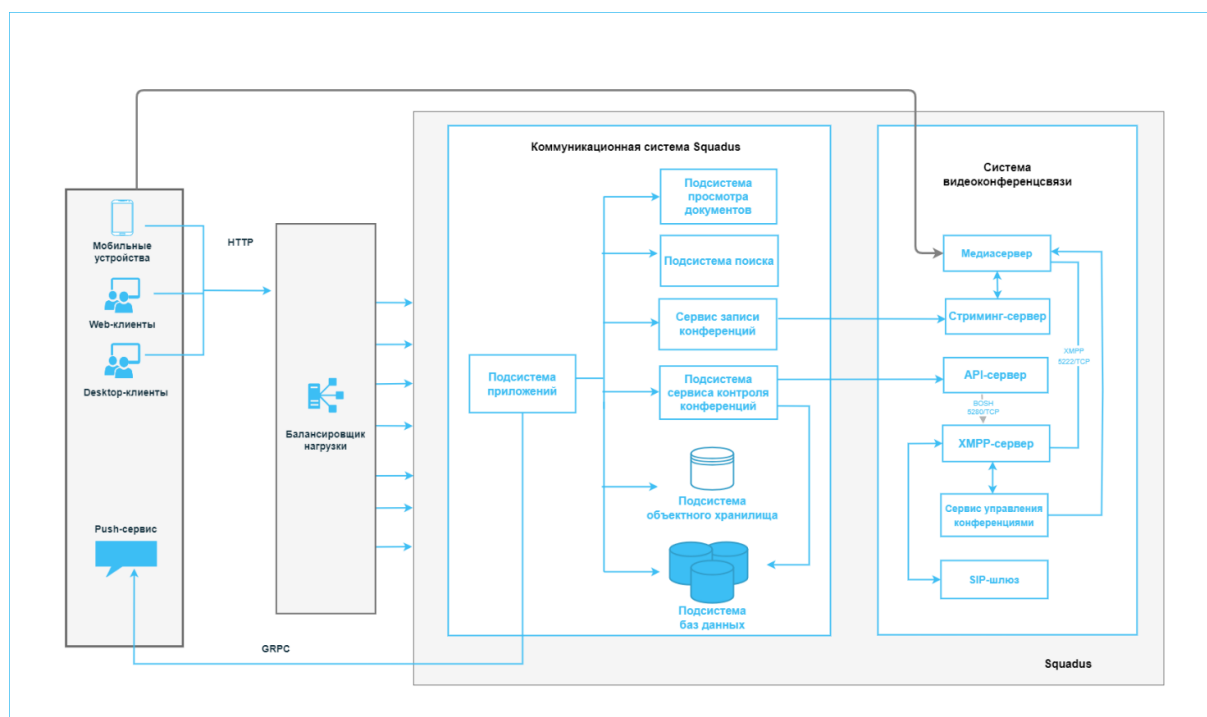
Рисунок 1 — Общая архитектурная схема ПО Squadus
