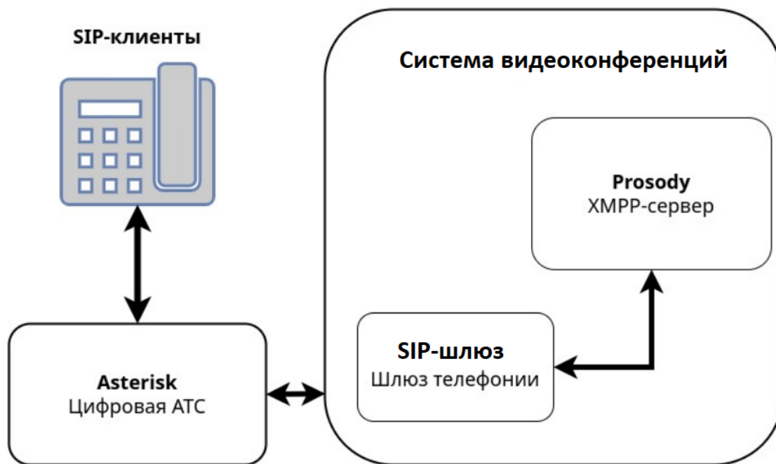
Рисунок 9 — Схема взаимодействия компонентов ПО Squadus и АТС Asterisk
