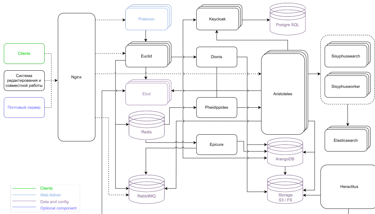
Рисунок 1 — Архитектурная схема Системы хранения данных
