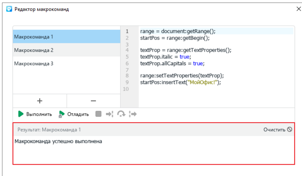
Рисунок 360 – Результат выполнения макроккоманды
