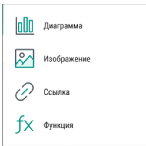
Рисунок 243 — Меню вставки
