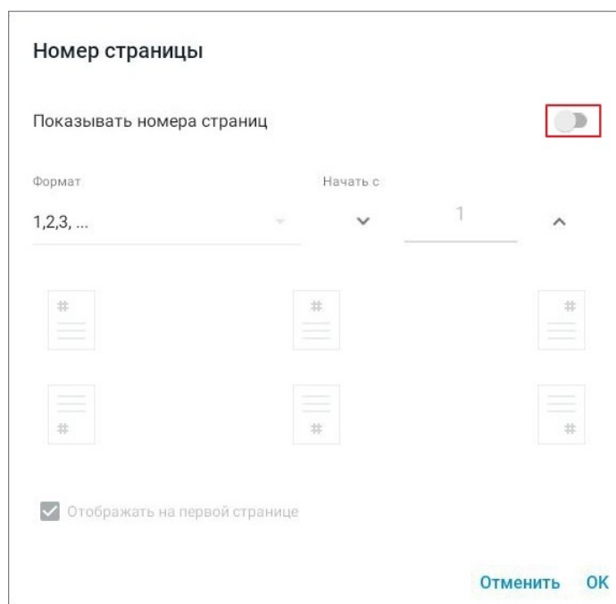
Рисунок 112 — Удаление нумерации
