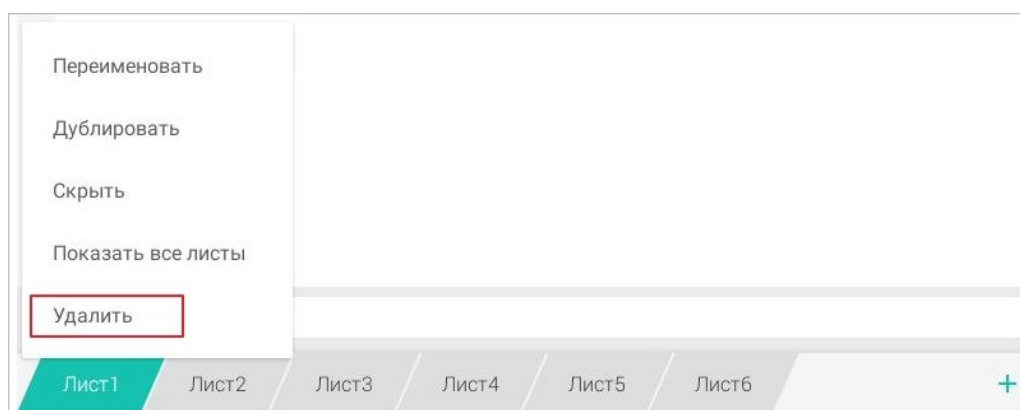
Рисунок 258 — Команда Удалить
