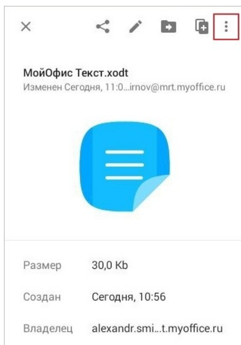
Рисунок 45 — Кнопка Еще
