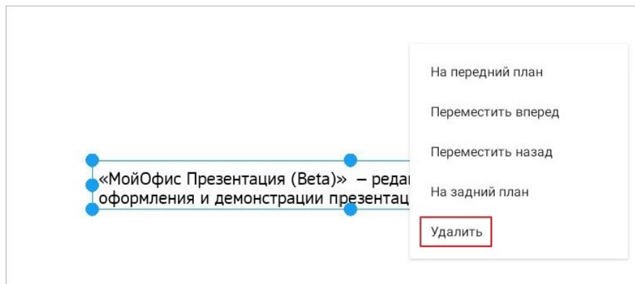
Рисунок 395 — Команда Удалить
