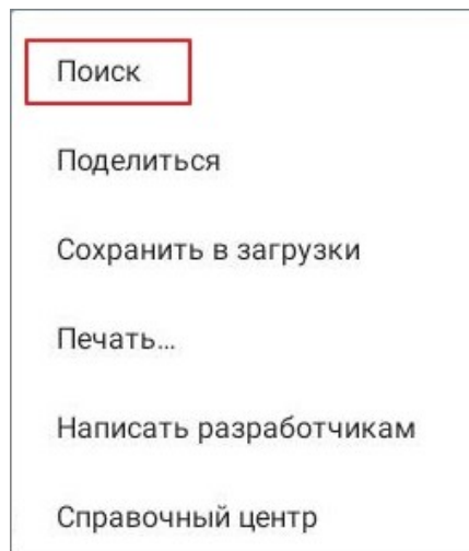
Рисунок 81 — Команда Поиск
