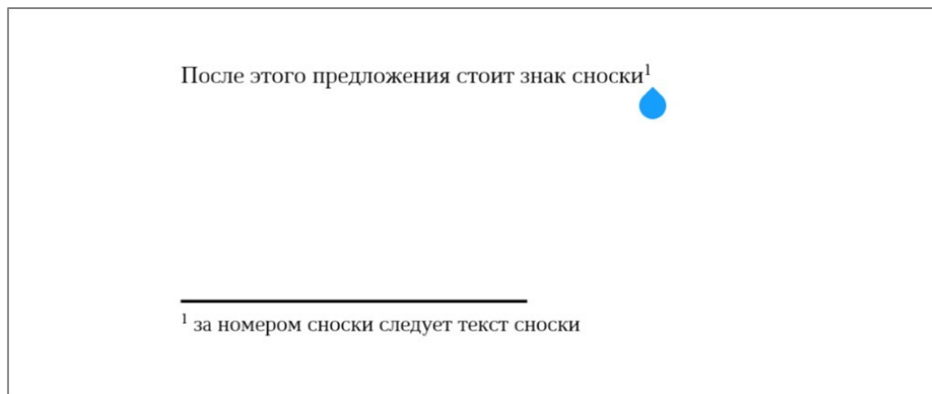
Рисунок 160 — Сноска
