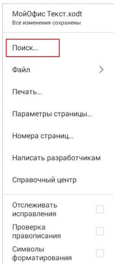
Рисунок 163 — Команда Поиск...
