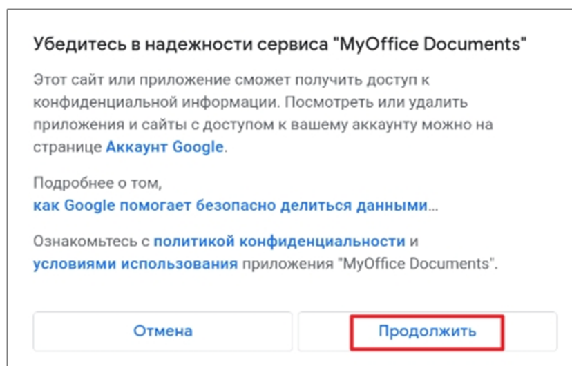
Рисунок 485 — Кнопка Продолжить
