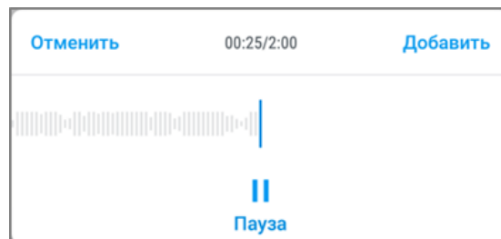
Рисунок 224 — Запись аудиокomentария
