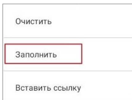
Рисунок 283 — Команда Заполнить
