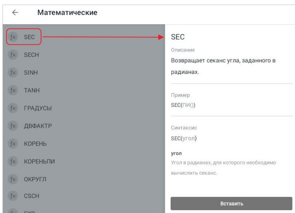
Рисунок 333 — Описание функции
