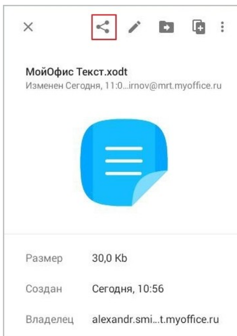
Рисунок 51 — Кнопка Поделиться
