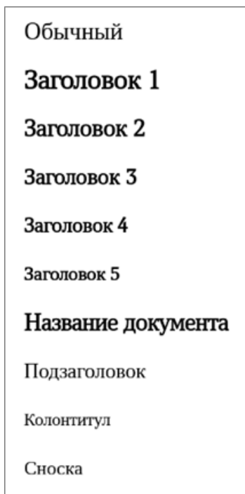
Рисунок 123 — Список стилей
