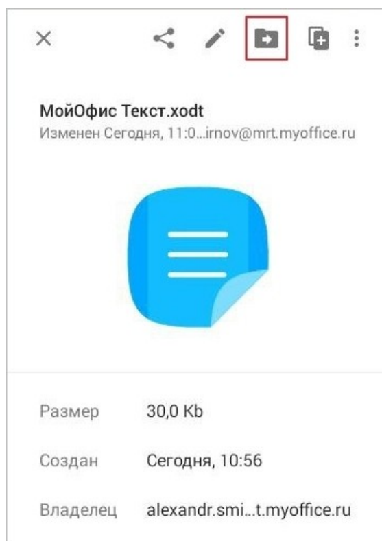
Рисунок 36 — Кнопка Переместить
