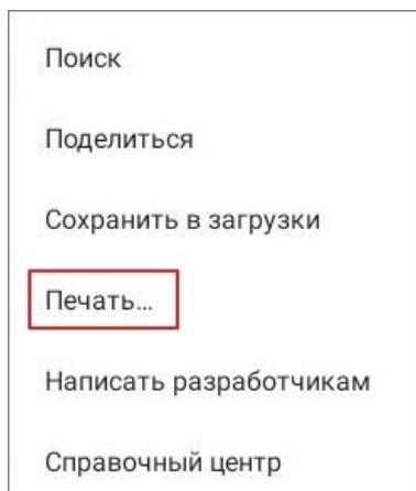
Рисунок 80 — Команда Печать
