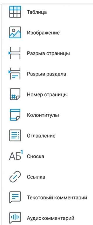
Рисунок 92 — Меню вставки
