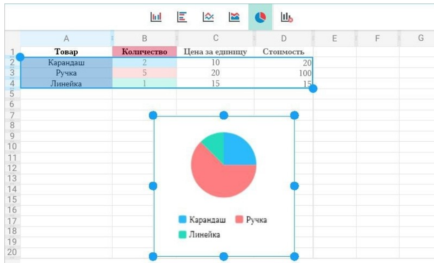
Рисунок 339 — Диаграмма
