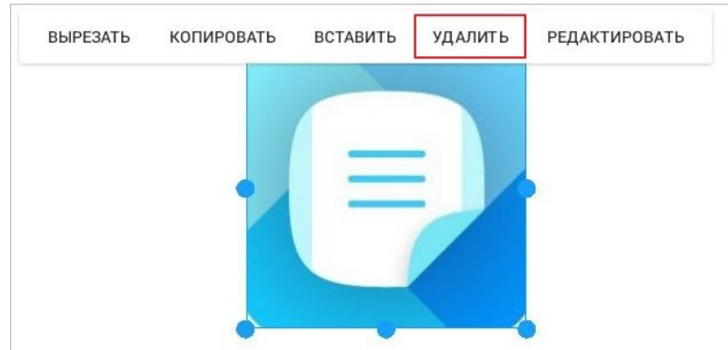
Рисунок 200 — Команда Удалить
