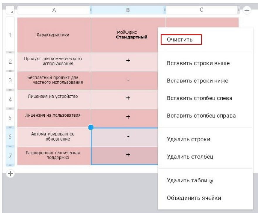
Рисунок 437 — Команда Очистить
