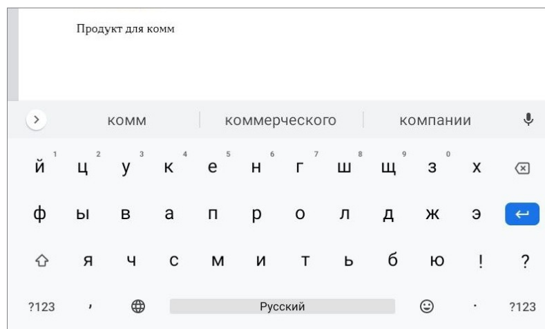
Рисунок 116 — Ввод текста
