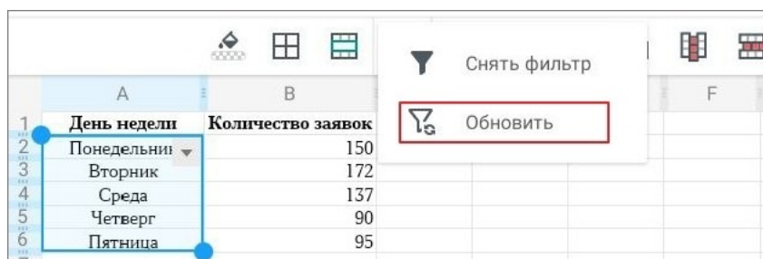
Рисунок 307 — Пункт Обновить
