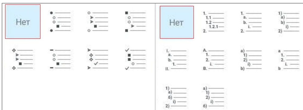
Рисунок 151 — Кнопка Нет
