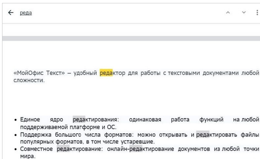
Рисунок 164 — Результаты поиска
