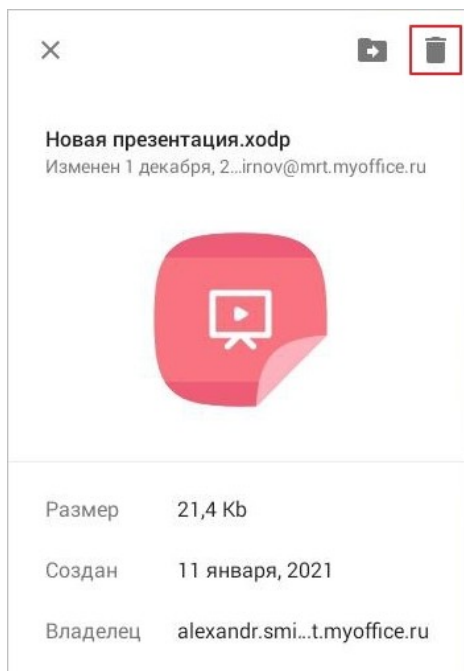
Рисунок 49 — Кнопка Удалить
