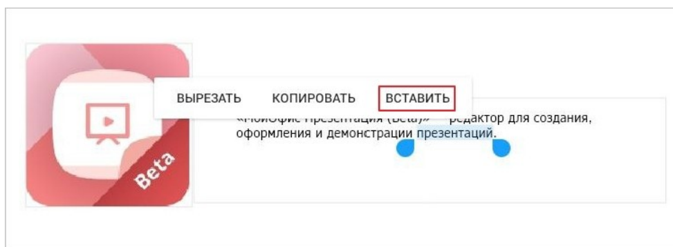
Рисунок 400 — Команда Вставить
