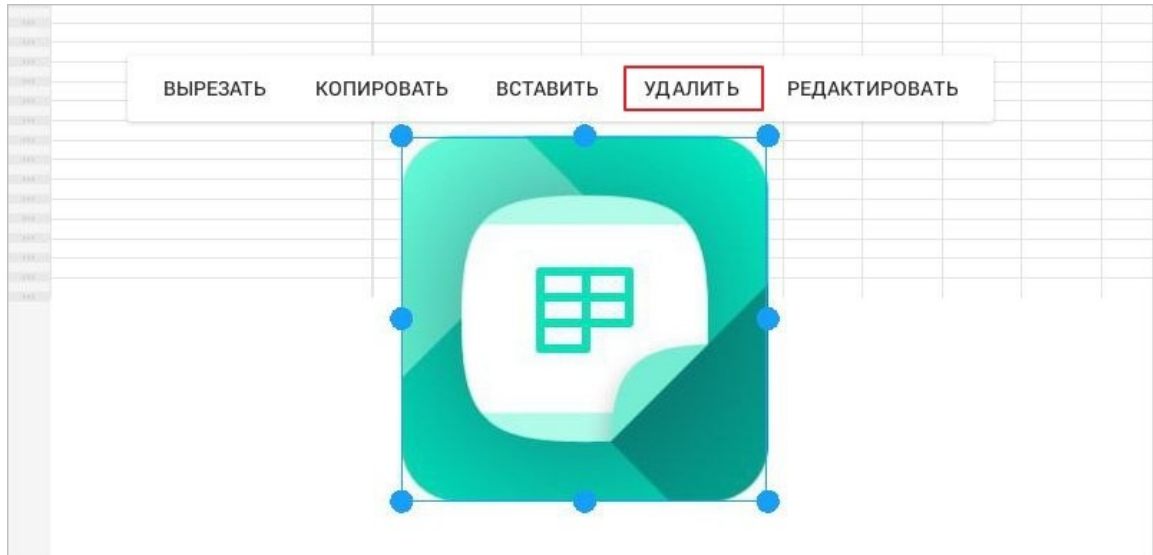
Рисунок 354 — Команда Удалить
