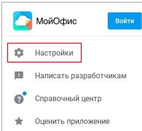
Рисунок 9 — Вкладка Настройки
