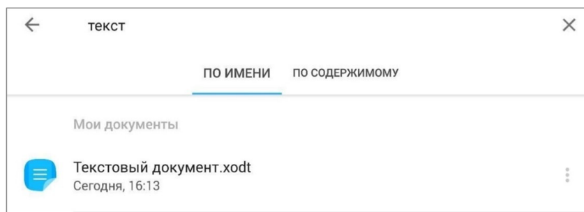
Рисунок 60 — Поиск объекта
