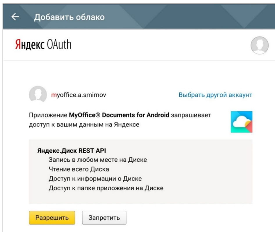
Рисунок 486 — Предоставление доступа
