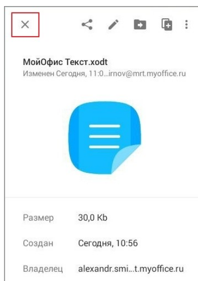
Рисунок 30 — Кнопка Закреть
