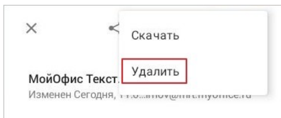
Рисунок 46 — Команда Удалить
