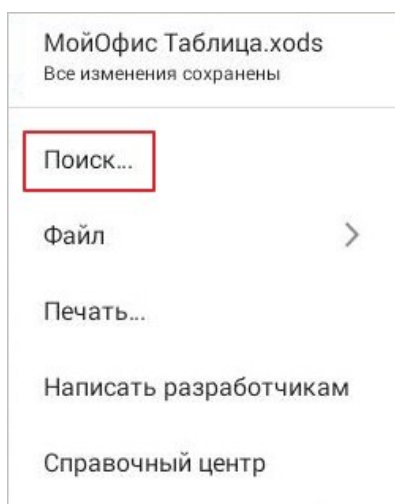
Рисунок 297 — Команда Поиск...
