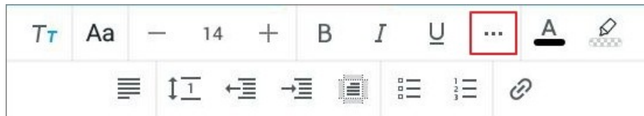
Рисунок 130 — Кнопка Больше
