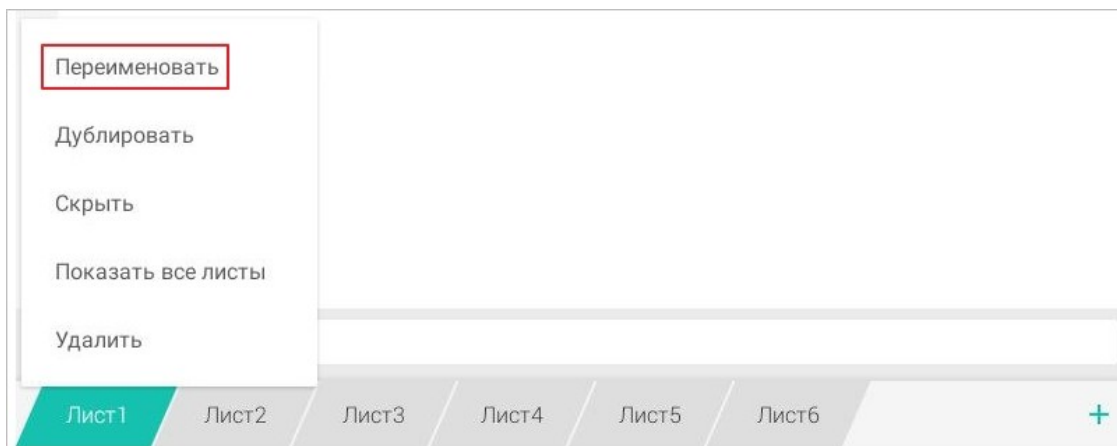
Рисунок 254 — Команда Переименовать
