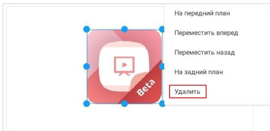
Рисунок 458 — Команда Удалить
