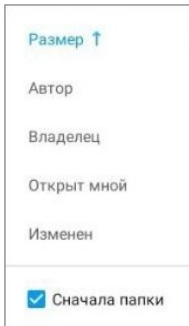
Рисунок 61 — Меню сортировки
