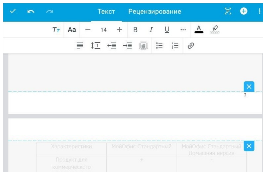
Рисунок 108 — Колонтитулы
