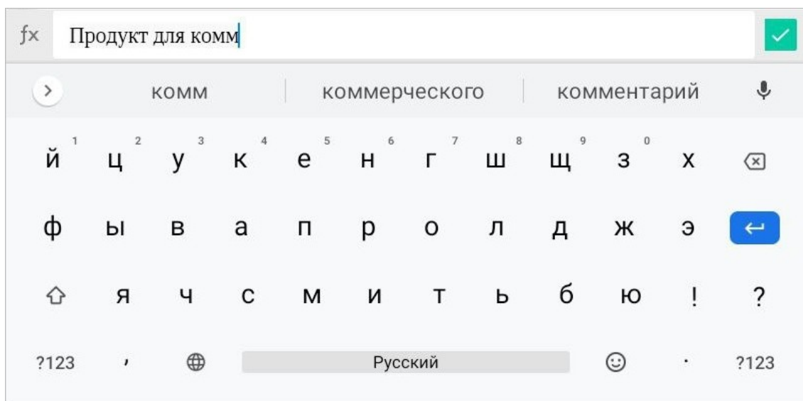
Рисунок 259 — Ввод текста
