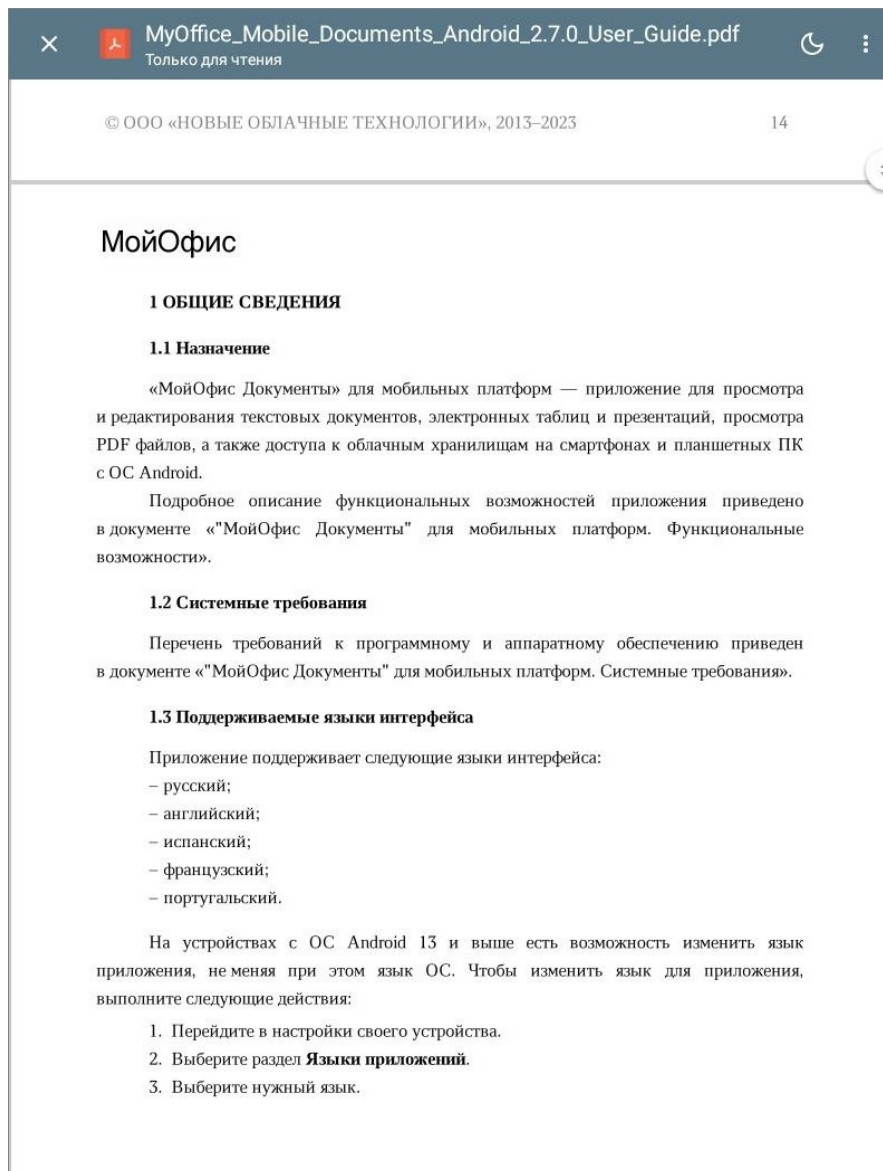
Рисунок 69 — Просмотр PDF
