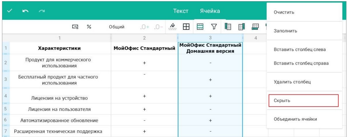
Рисунок 322 — Команда Скрыть
