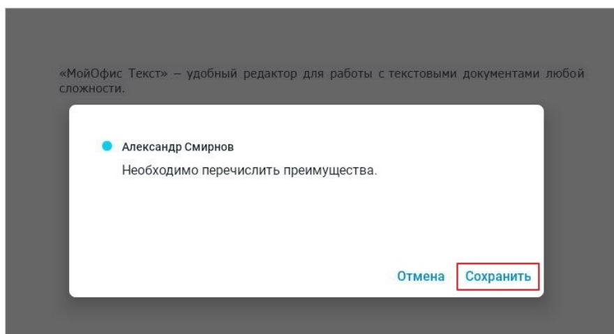
Рисунок 221 — Кнопка Сохранить
