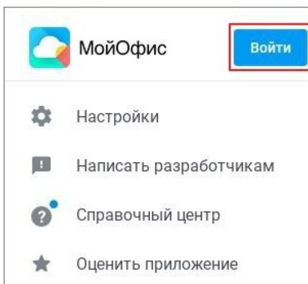
Рисунок 8 — Кнопка Войти
