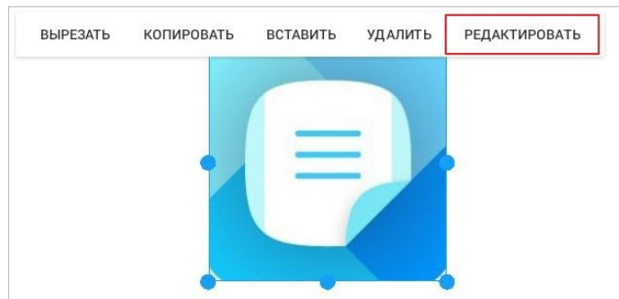
Рисунок 194 — Команда Редактировать
