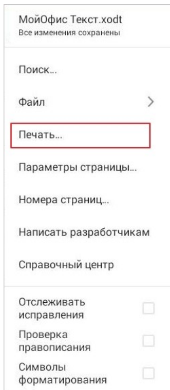
Рисунок 476 — Команда Печать
