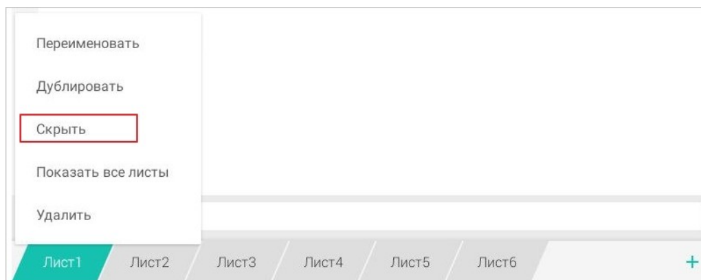
Рисунок 255 — Команда Скрыть
