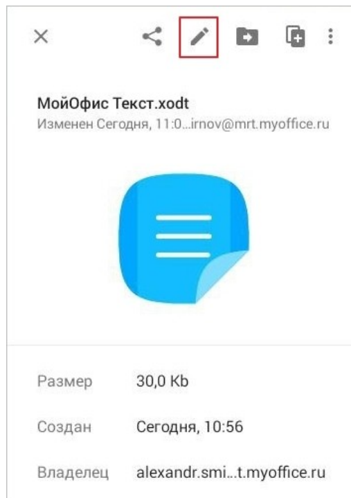
Рисунок 40 — Кнопка Переименовать
