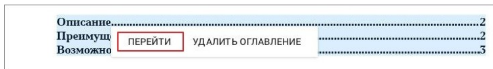
Рисунок 114 — Команда Перейти
