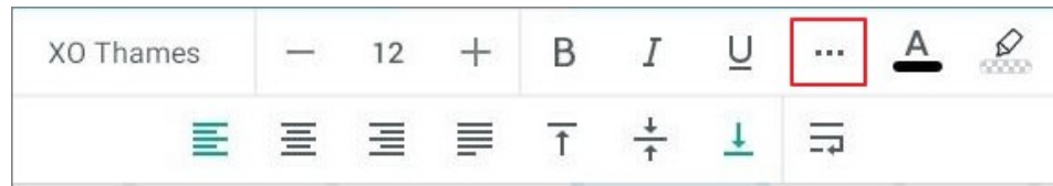
Рисунок 269 — Кнопка Больше
