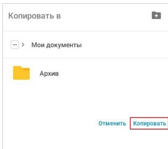
Рисунок 34 — Кнопка Копировать
