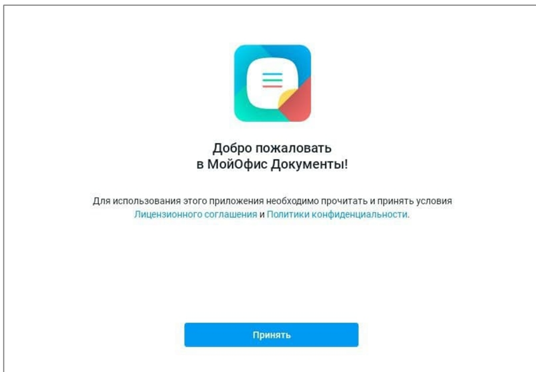
Рисунок 5 — Приветственный экран
