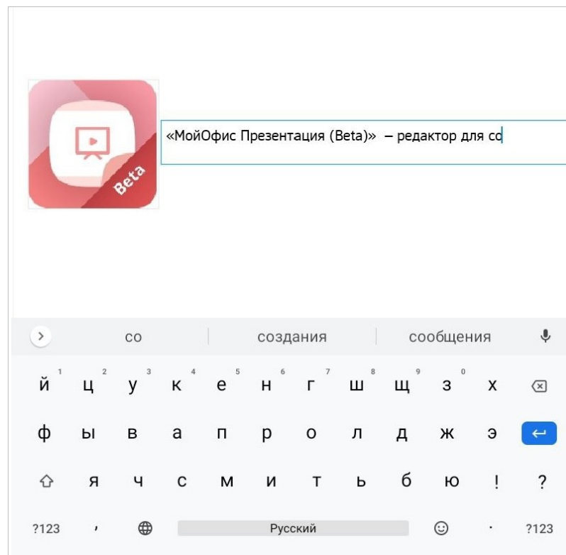
Рисунок 396 — Ввод текста
