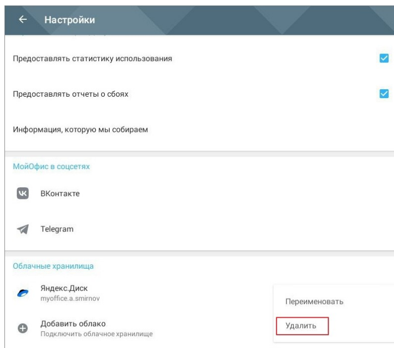
Рисунок 490 — Команда Удалить
