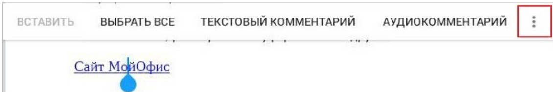
Рисунок 156 — Кнопка Больше
