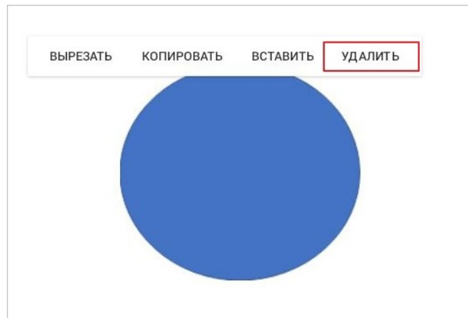
Рисунок 202 — Команда Удалить
