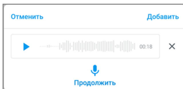
Рисунок 225 — Кнопка Продолжить
