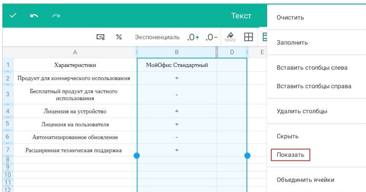
Рисунок 324 — Команда Показать
