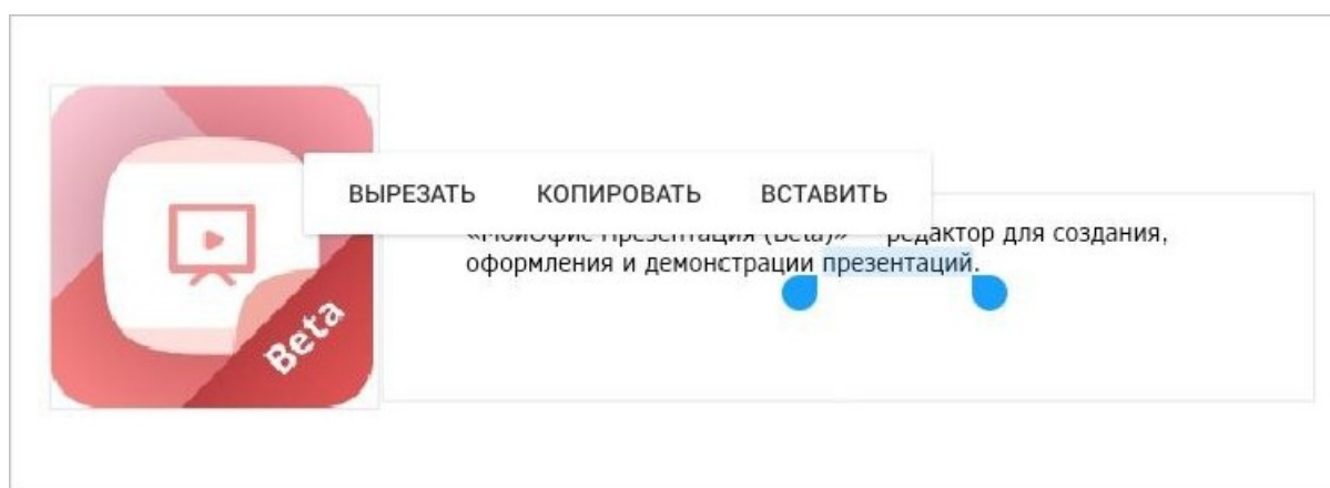
Рисунок 397 — Выделение текста
