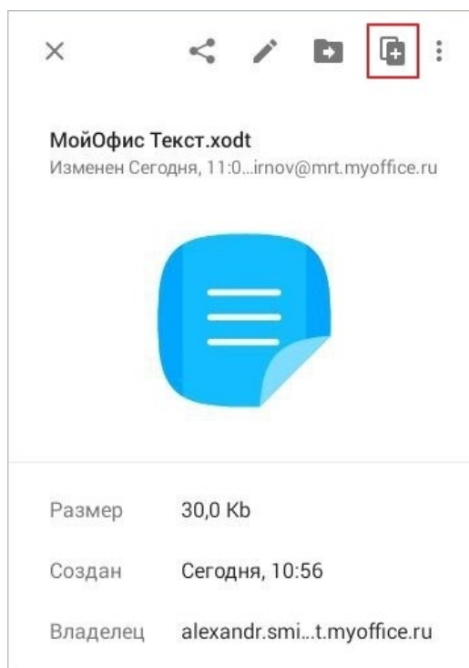
Рисунок 31 — Кнопка Копировать
