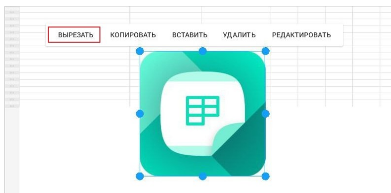
Рисунок 343 — Команда Вырезать
