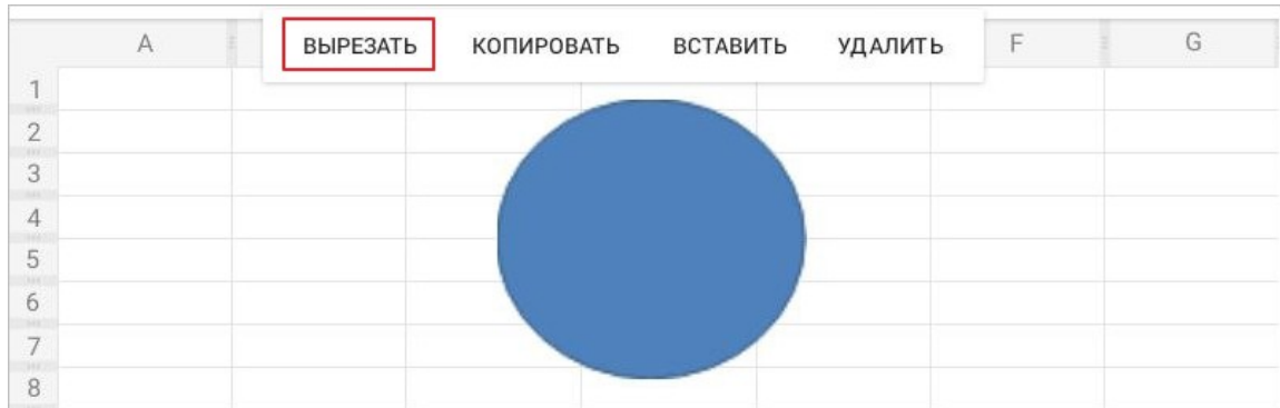
Рисунок 355 — Команда Вырезать
