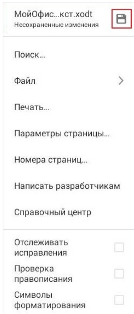
Рисунок 478 — Кнопка сохранения
