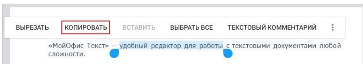
Рисунок 120 — Команда Копировать
