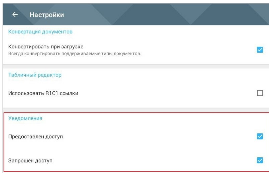
Рисунок 492 — Настройка уведомлений
