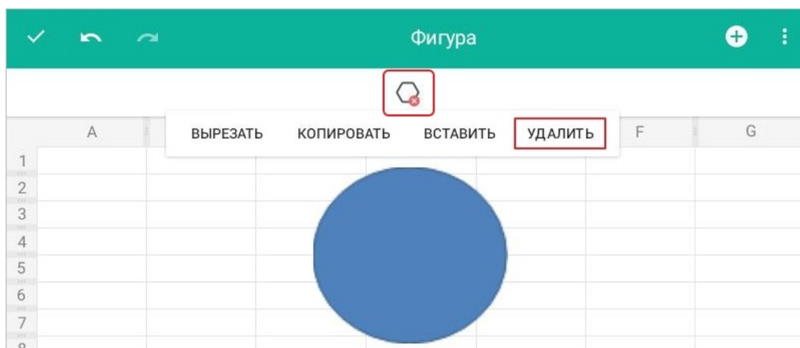
Рисунок 358 — Удаление фигуры
