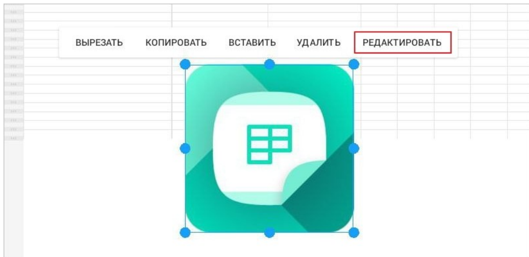
Рисунок 348 — Команда Редактировать
