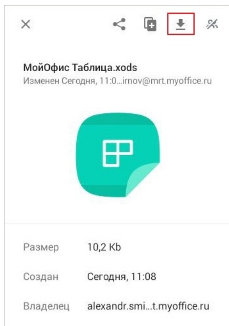
Рисунок 57 — Кнопка Скачать
