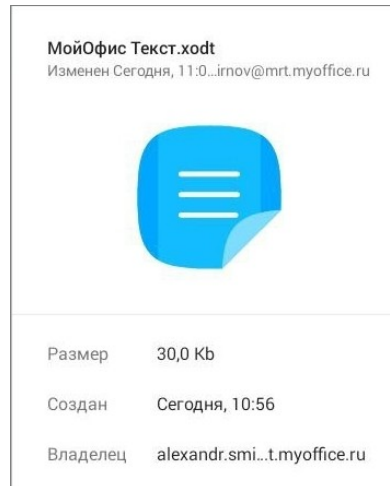
Рисунок 28 — Панель сведений
