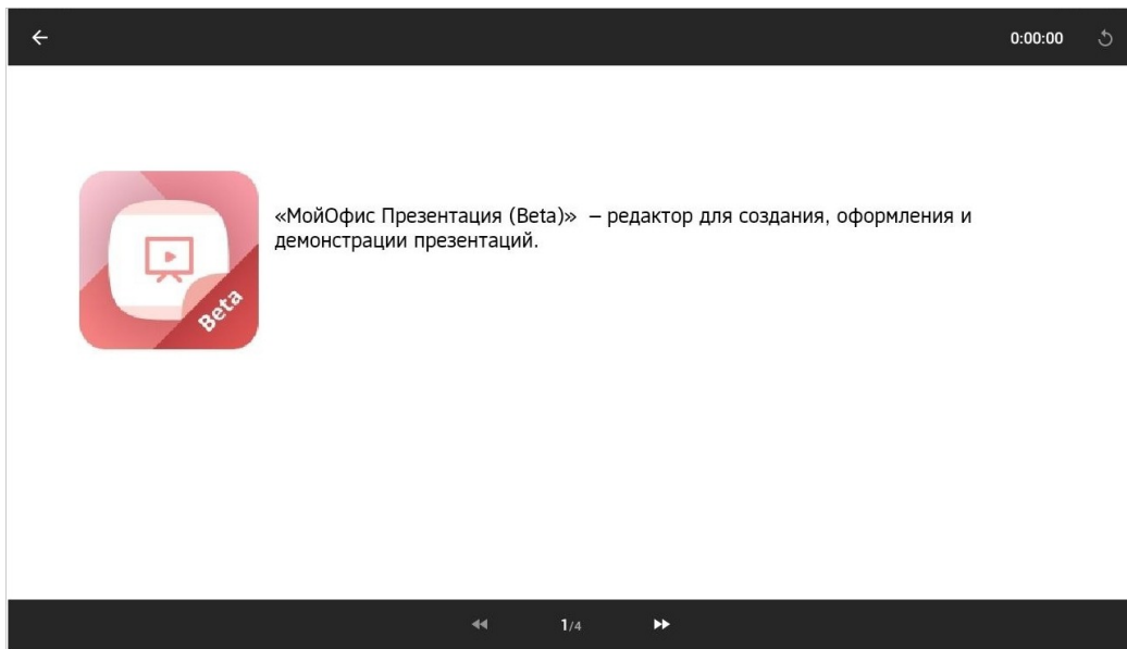
Рисунок 392 — Слайд-шоу
