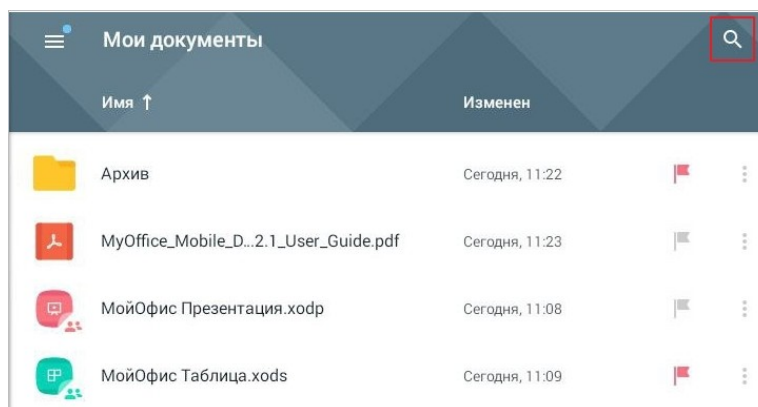
Рисунок 59 — Кнопка Поиск
