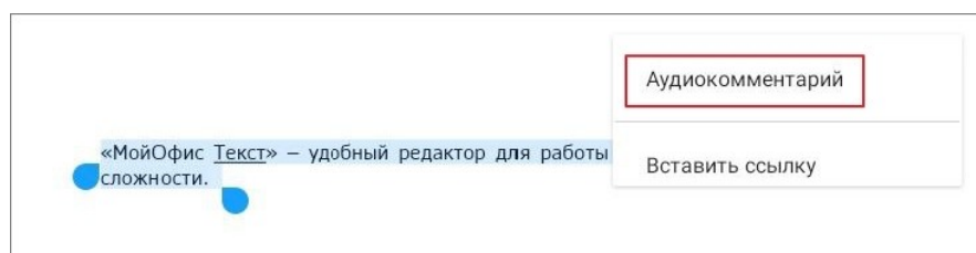
Рисунок 227 — Команда Аудиокомментарий
