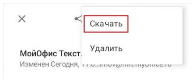
Рисунок 55 — Команда Скачать
