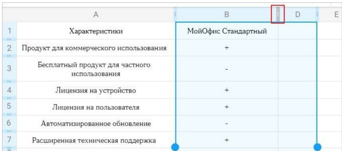
Рисунок 323 — Скрытые столбцы
