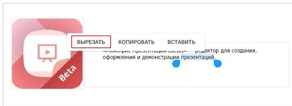
Рисунок 398 — Команда Вырезать
