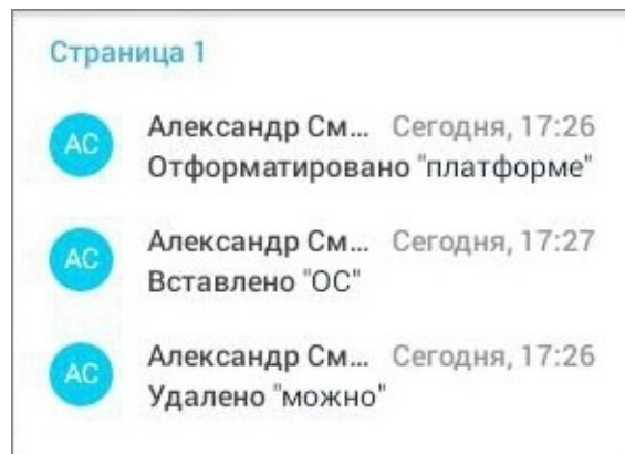
Рисунок 214 — Панель рецензирования
