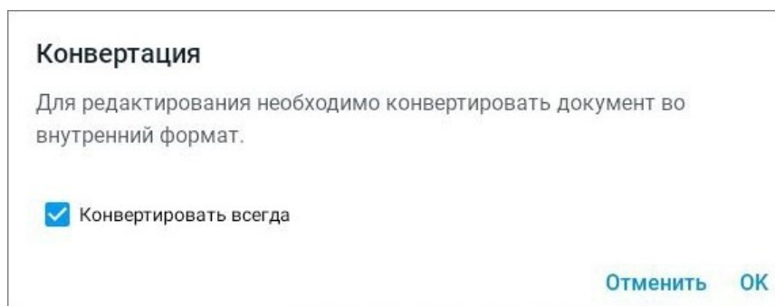
Рисунок 85 — Окно Конвертация
