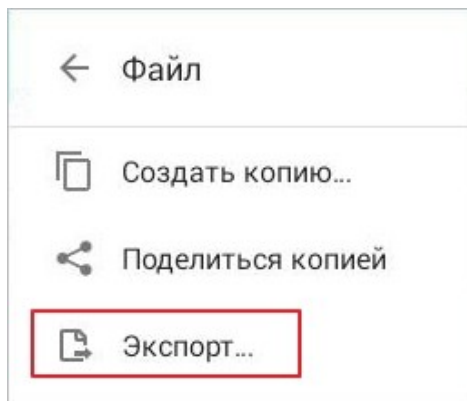
Рисунок 475 — Команда Экспорт
