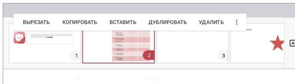
Рисунок 382 — Контекстное меню
