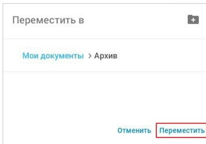
Рисунок 38 — Кнопка Переместить
