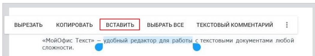
Рисунок 121 — Команда Вставить
