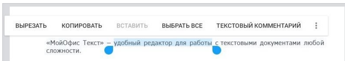
Рисунок 117 — Выделение текста
