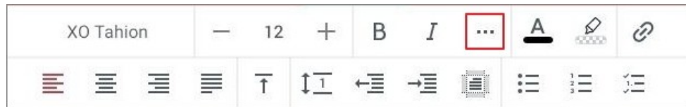
Рисунок 406 — Кнопка Больше
