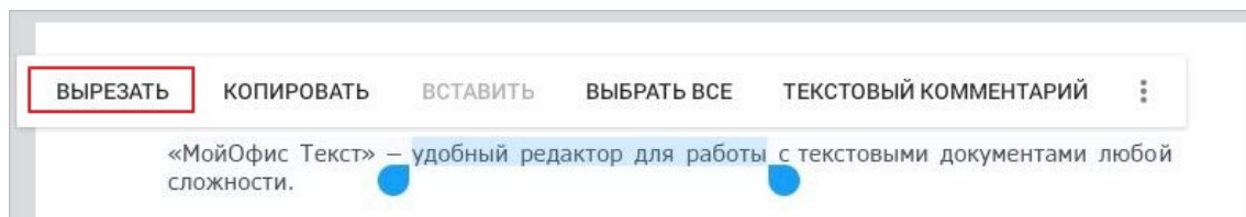
Рисунок 119 — Команда Вырезать
