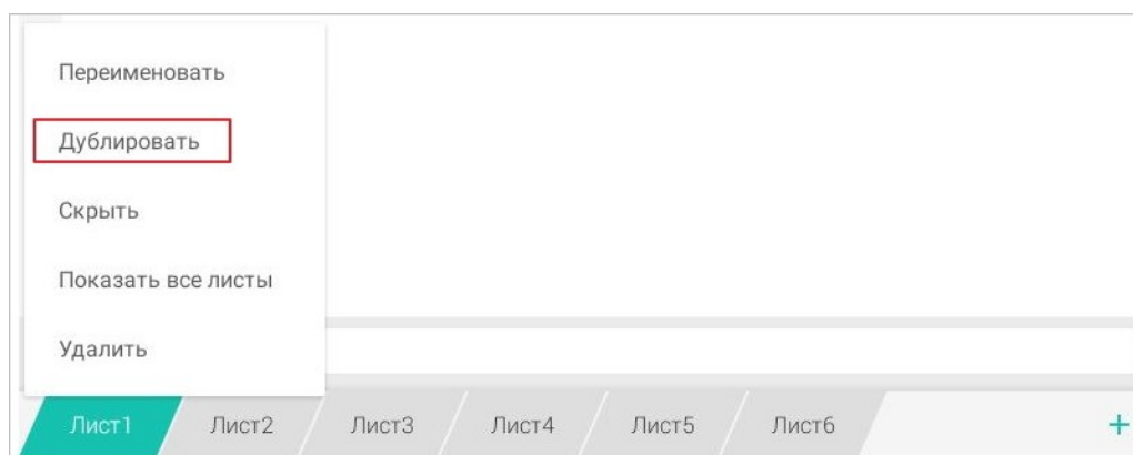
Рисунок 257 — Команда Дублировать
