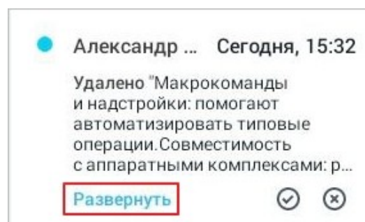
Рисунок 215 — Кнопка Развернуть
