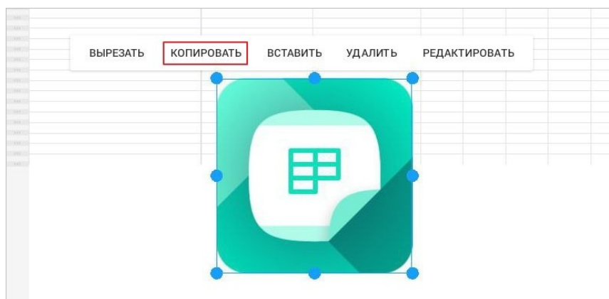
Рисунок 344 — Команда Копировать
