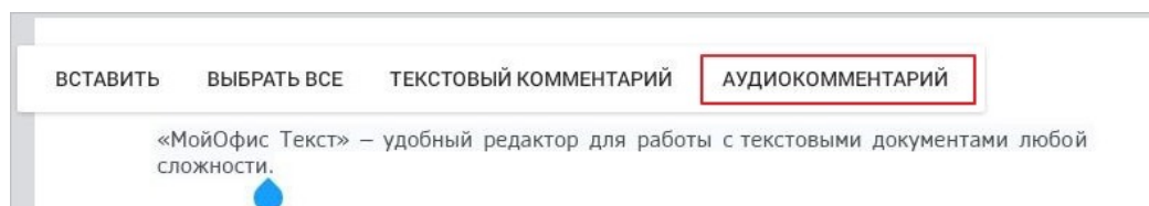
Рисунок 226 — Команда Аудиокомментарий
