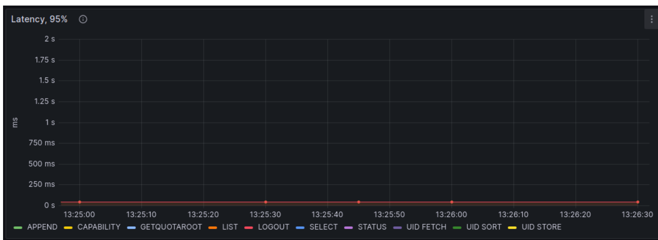
Рисунок 36 – Панель Latency, 95%
