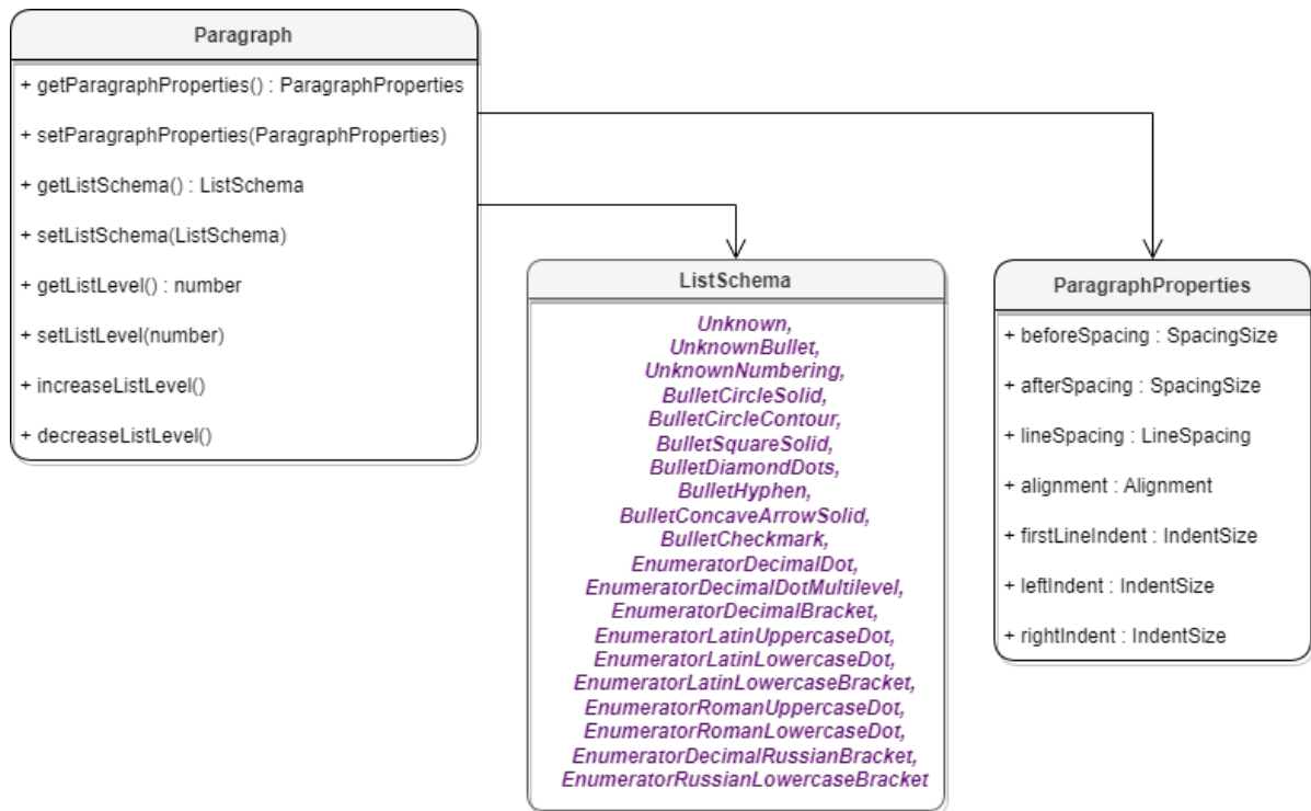
Рисунок 34 – Объектная модель таблиц для работы со свойствами параграфа
