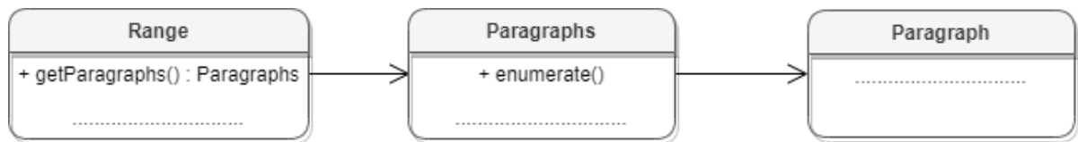
Рисунок 36 – Объектная модель для работы со списком абзацев
