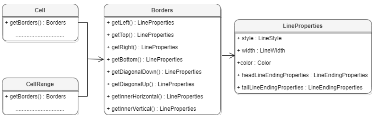
Рисунок 19 – Таблицы для работы с границами ячеек
