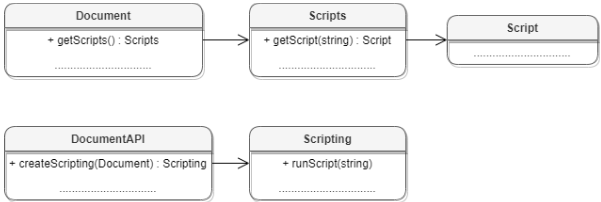
Рисунок 16 – Объектная модель таблиц для работы с макросами
