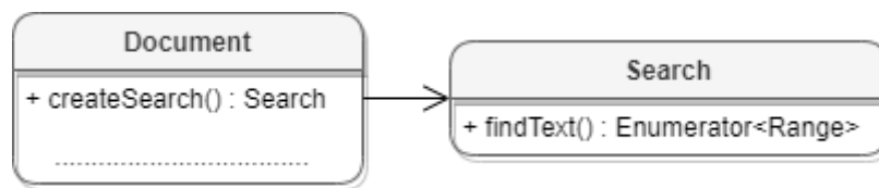
Рисунок 8 – Объектная модель для поиска в документе
