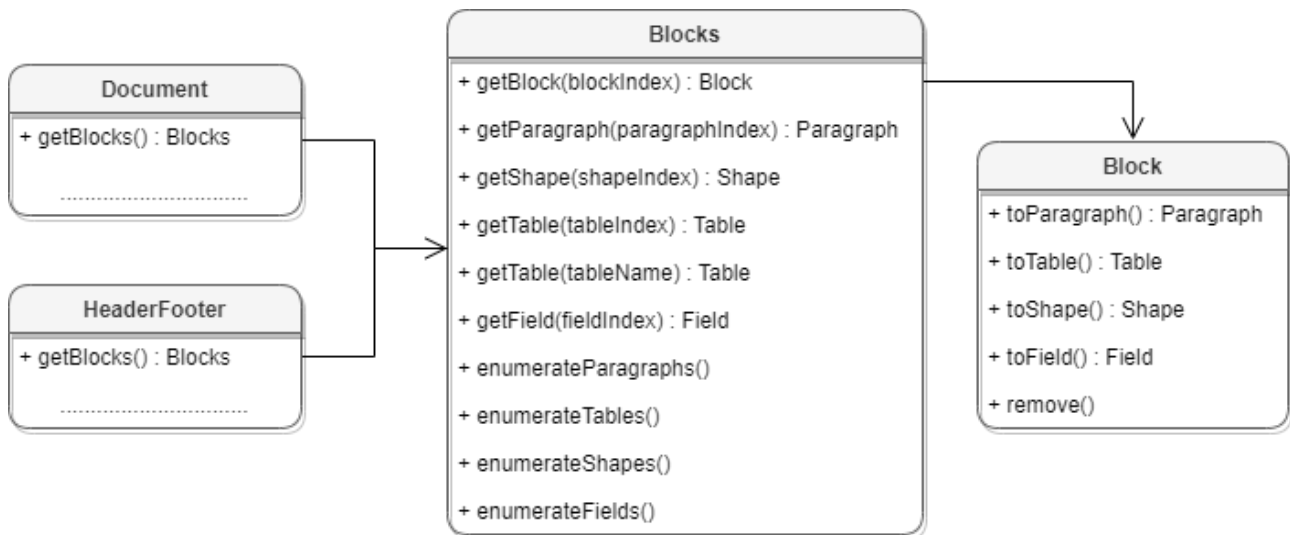
Рисунок 22 – Объектная модель таблицы DocumentAPI.Blocks
