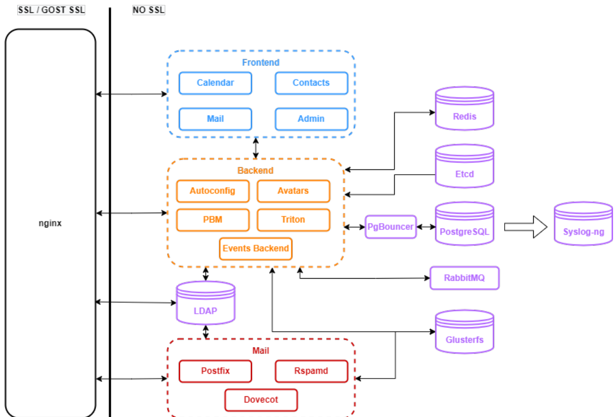
Рисунок 1. Архитектурная схема «МойОфис Почта»
