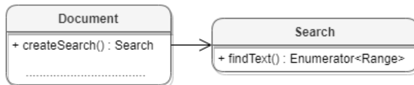
Рисунок 16 – Объектная модель для поиска в документе
