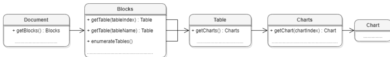
Рисунок 10 – Объектная модель таблиц для работы с диаграммами
