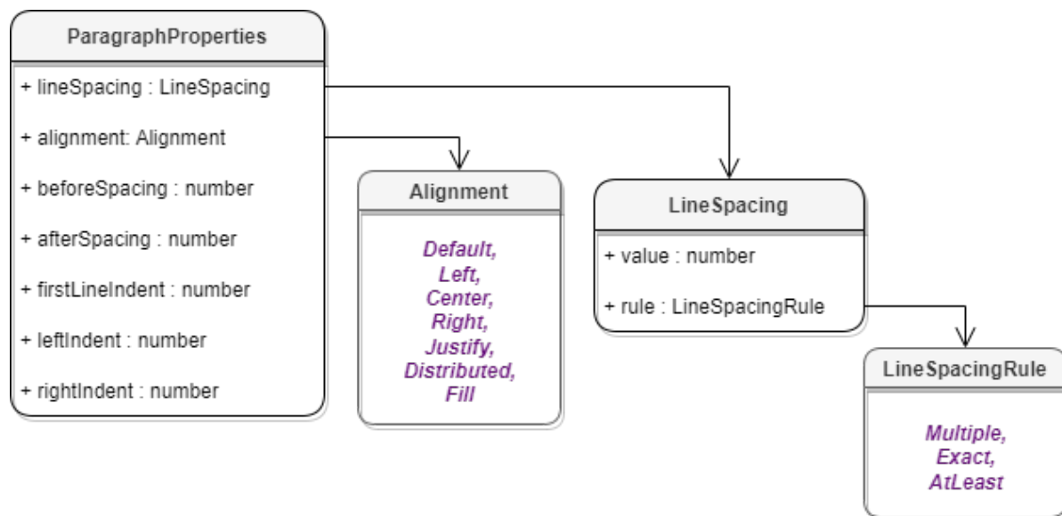
Рисунок 37 – Объектная модель таблиц для работы со свойствами параграфа
