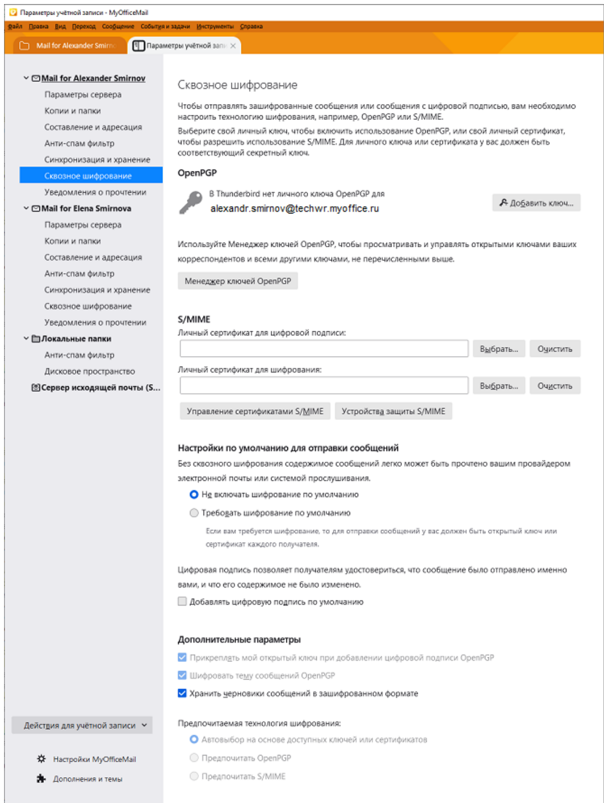
Рисунок 116 - Панель настройки сквозного шифрования
