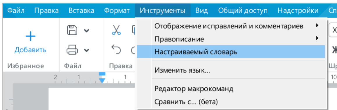
Рисунок 6 – Командное меню
