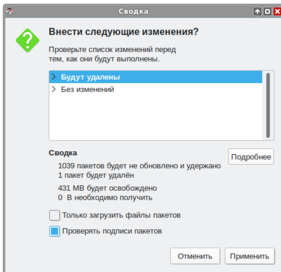
Рисунок 22 – Окно Сводка
