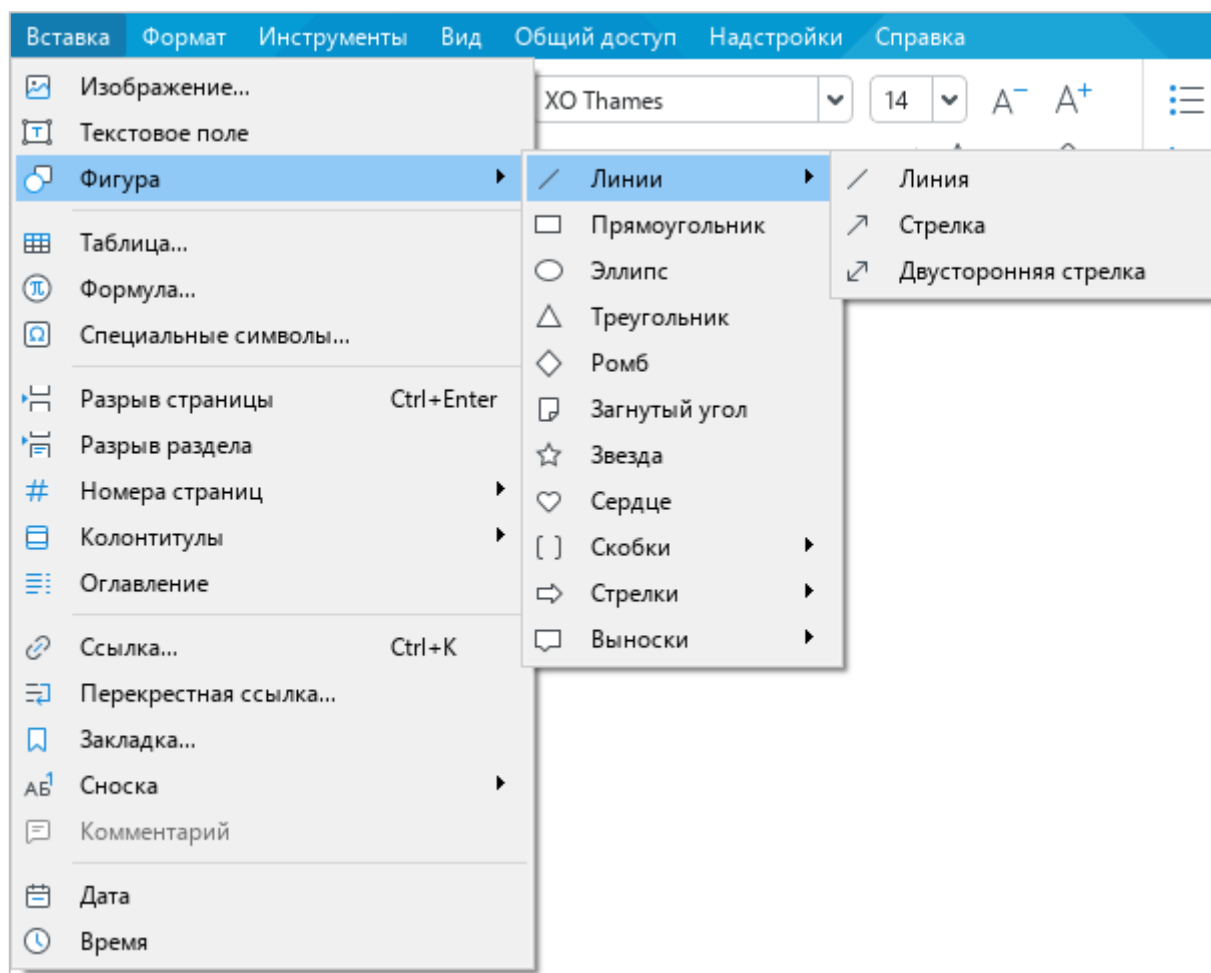
Рисунок 193 – Командное меню Вставка
