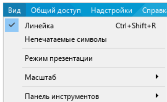
Рисунок 20 – Меню Вид
