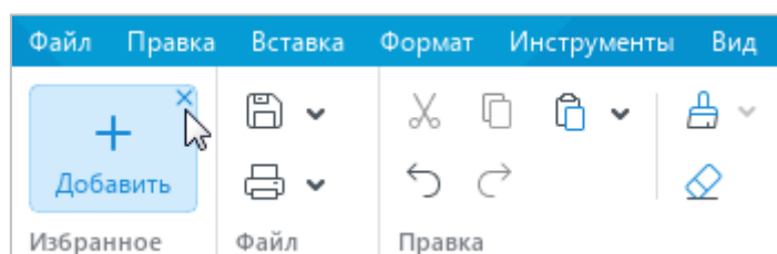
Рисунок 33 – Раздел Избранное
