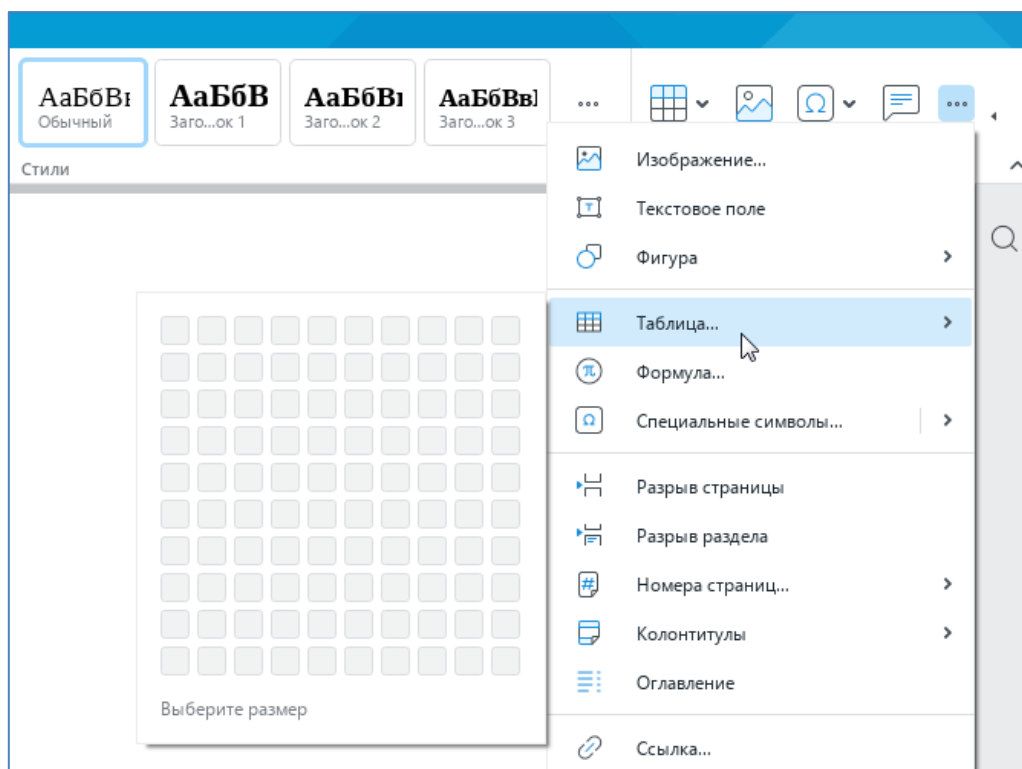
Рисунок 217 – Панель вставки
