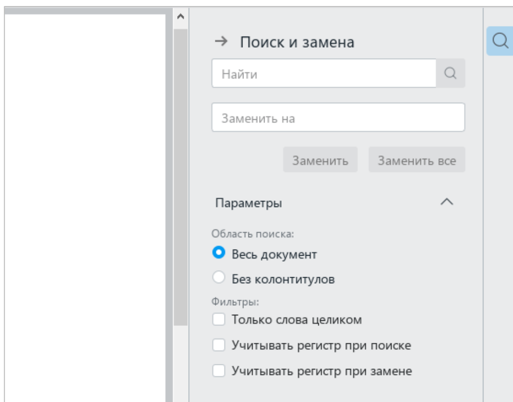
Рисунок 148 – Параметры поиска
