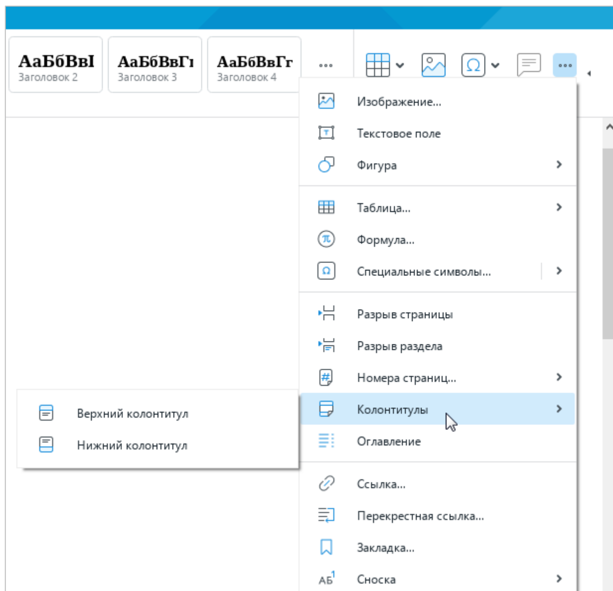
Рисунок 279 – Панель вставки
