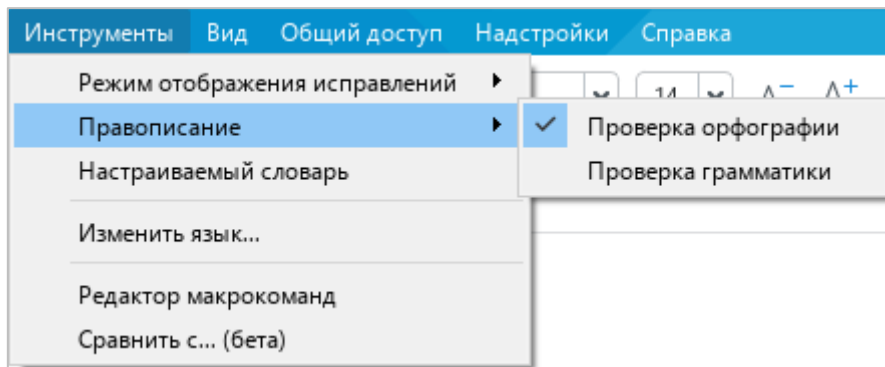
Рисунок 19 – Подменю Правописание
