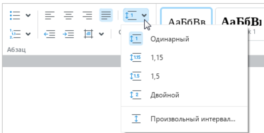
Рисунок 56 – Межстрочный интервал
