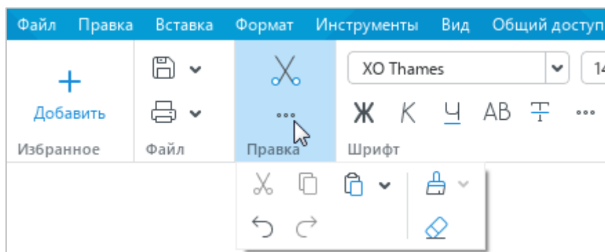
Рисунок 30 – Инструменты раздела
