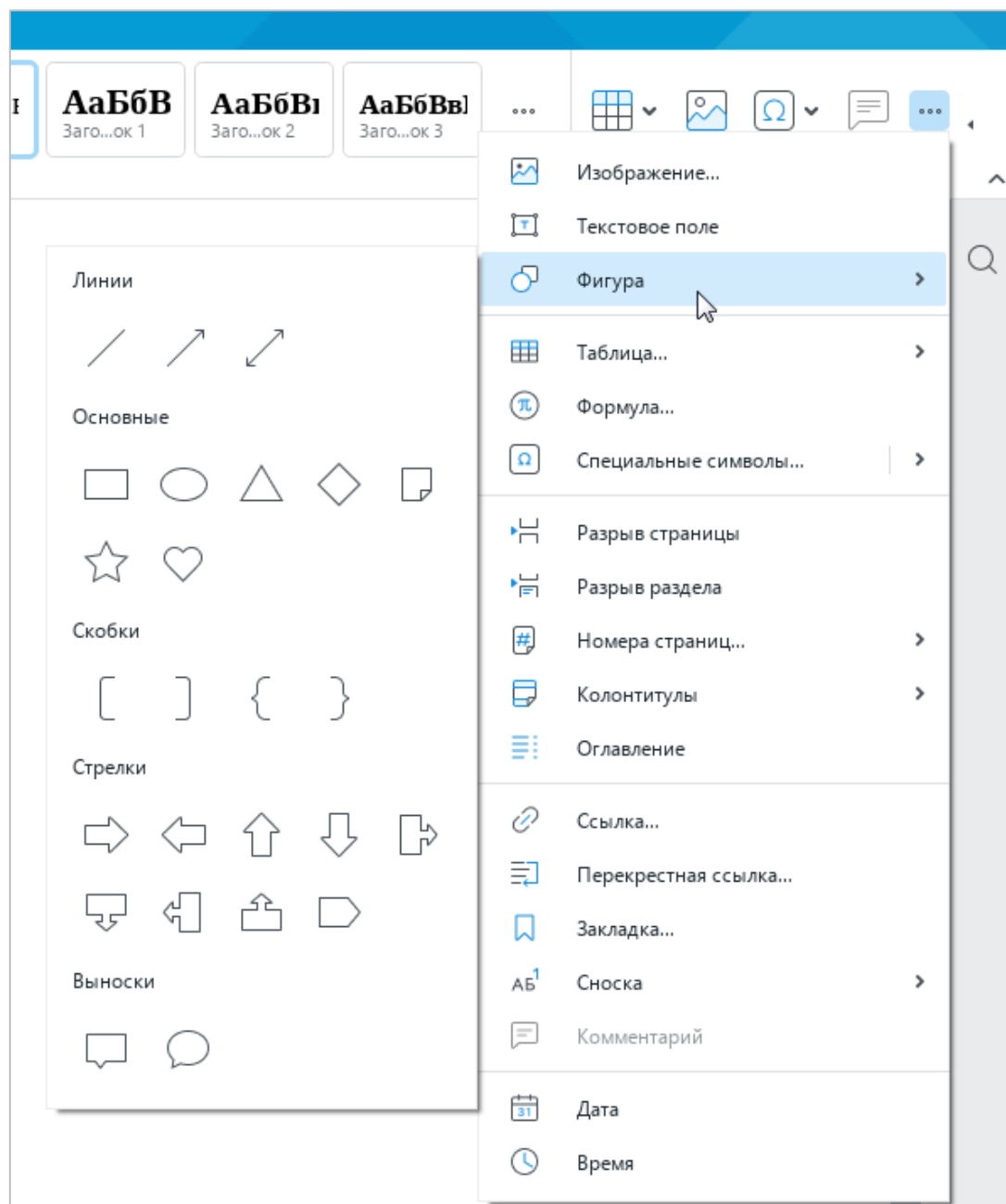
Рисунок 241 – Панель вставки
