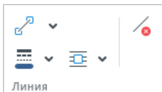
Рисунок 72 – Раздел Линия
