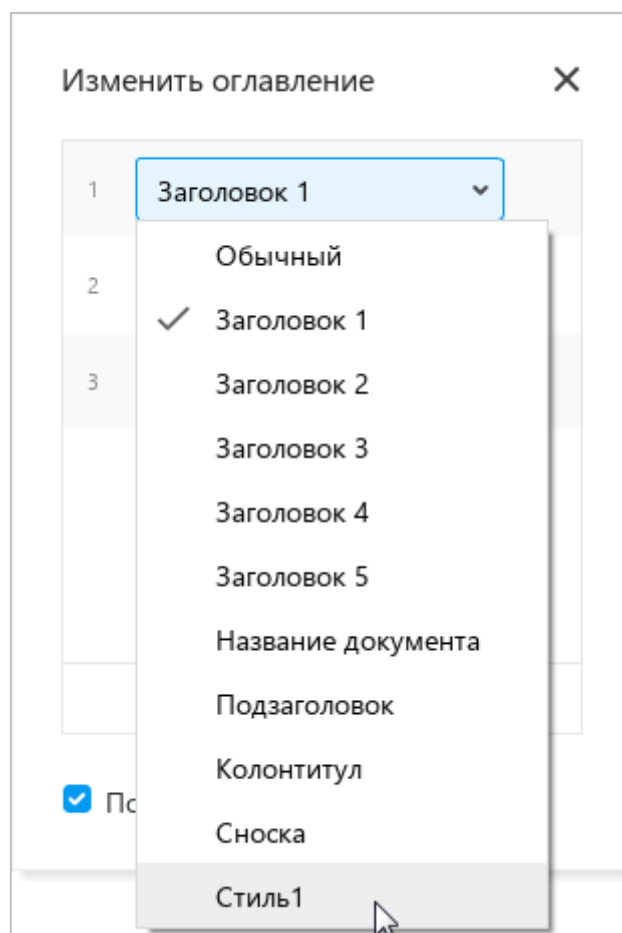
Рисунок 306 – Выбор стиля
