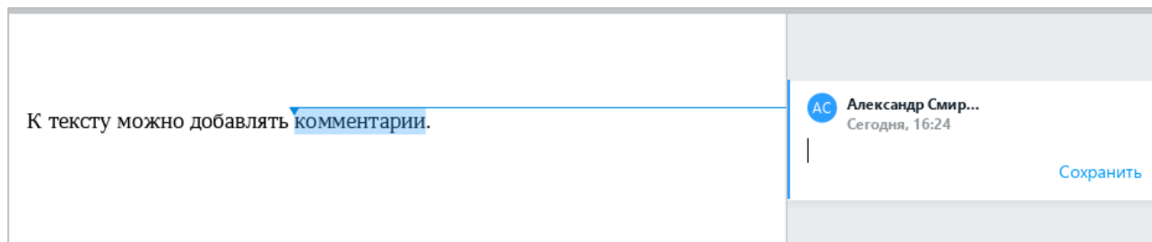
Рисунок 345 – Удаление комментария
