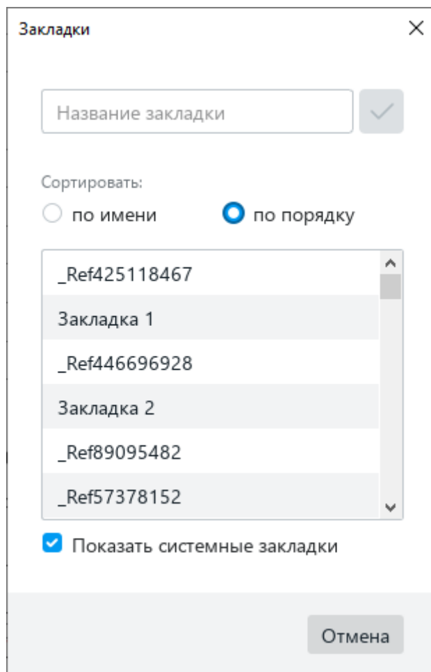
Рисунок 127 – Окно Закладки
