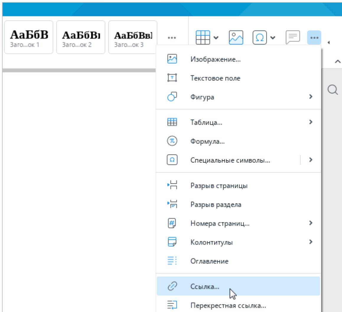
Рисунок 113 – Панель вставки
