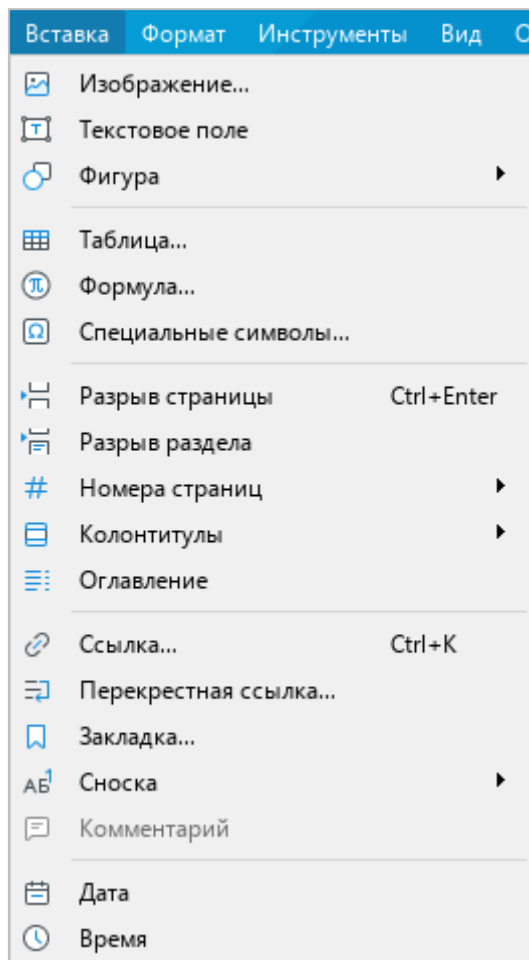
Рисунок 12 – Меню Вставка
