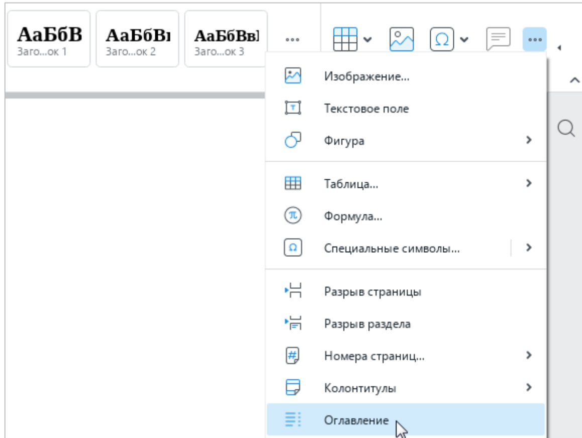
Рисунок 301 – Панель вставки
