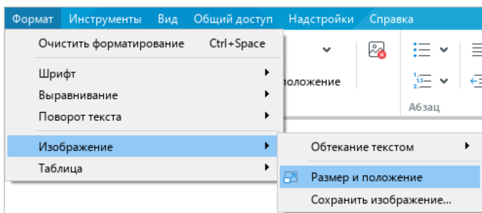
Рисунок 226 – Подменю Изображение
