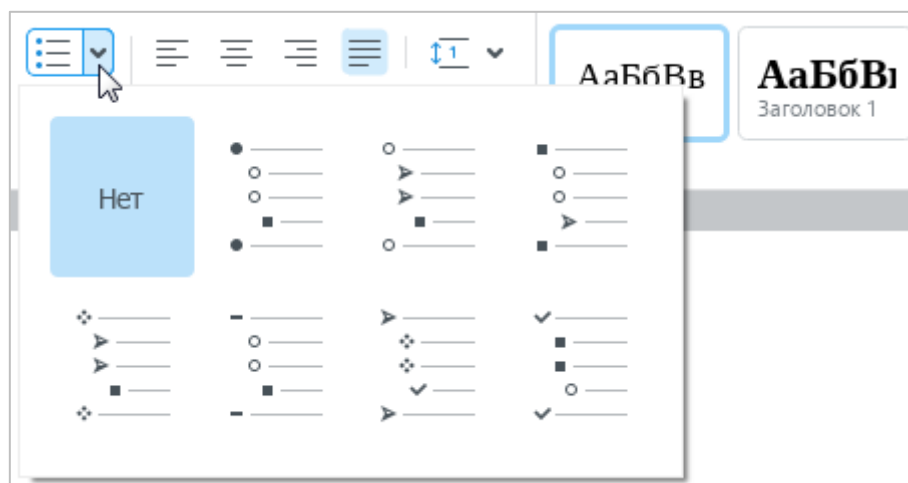
Рисунок 53 – Маркированный список
