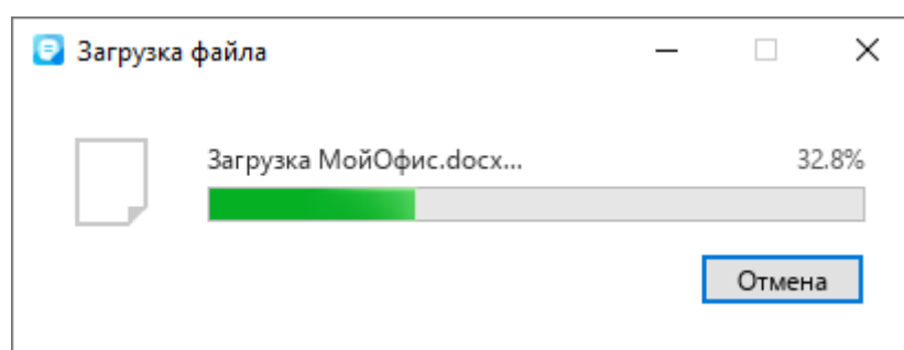
Рисунок 366 – Загрузка файла
