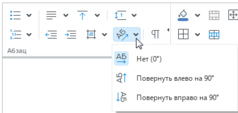
Рисунок 58 – Поворот текста
