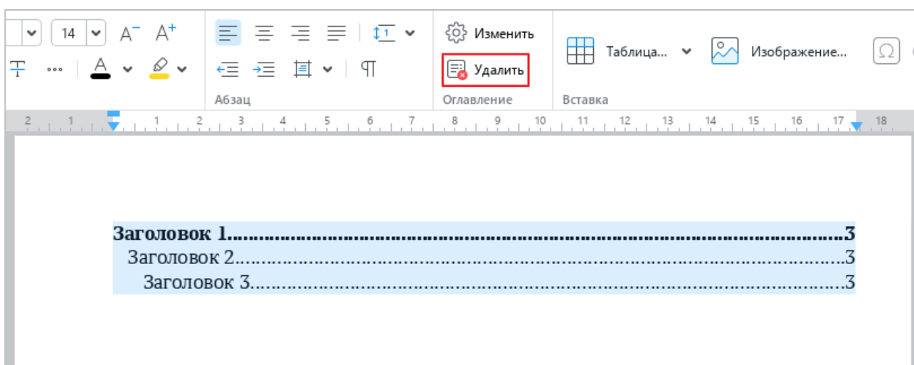
Рисунок 308 – Кнопка Удалить
