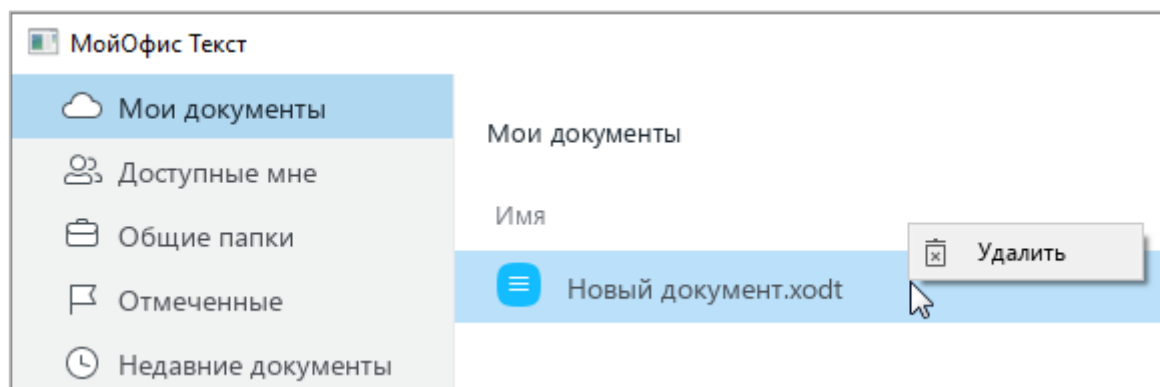
Рисунок 368 – Команда Удалить
