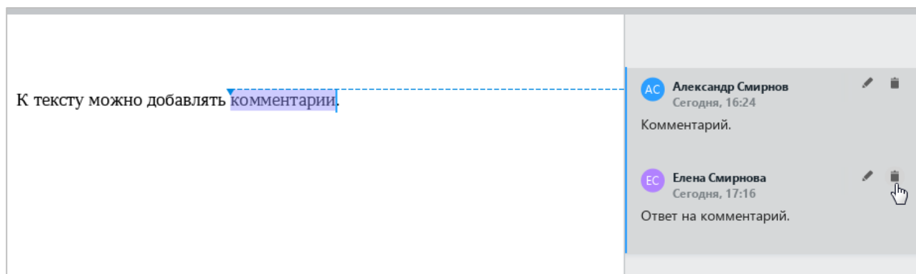
Рисунок 347 – Удаление ответа
