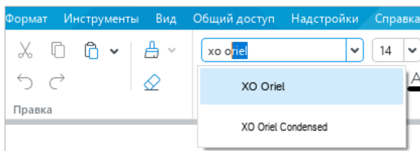
Рисунок 159 – Поиск шрифта
