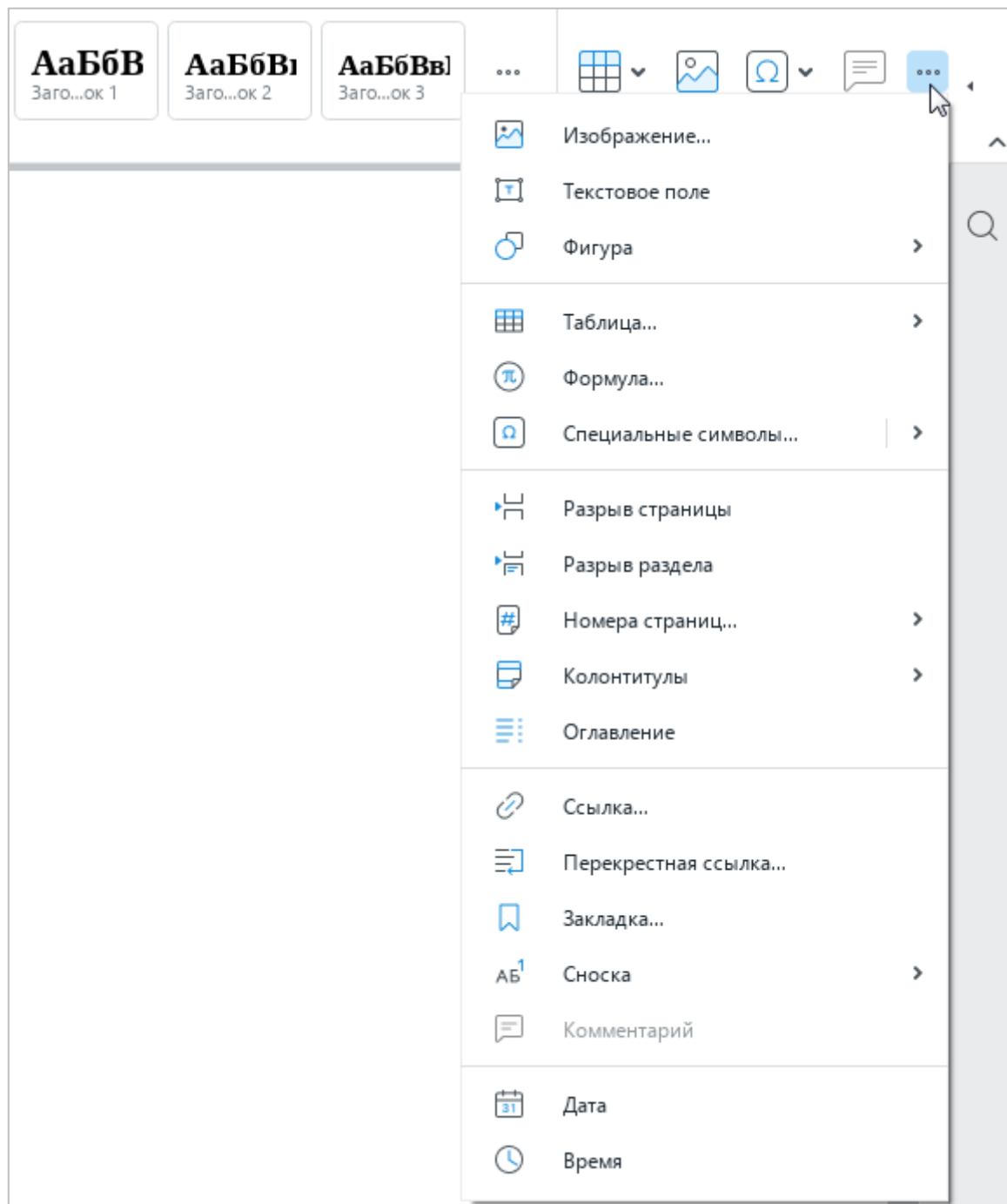
Рисунок 62 – Панель вставки
