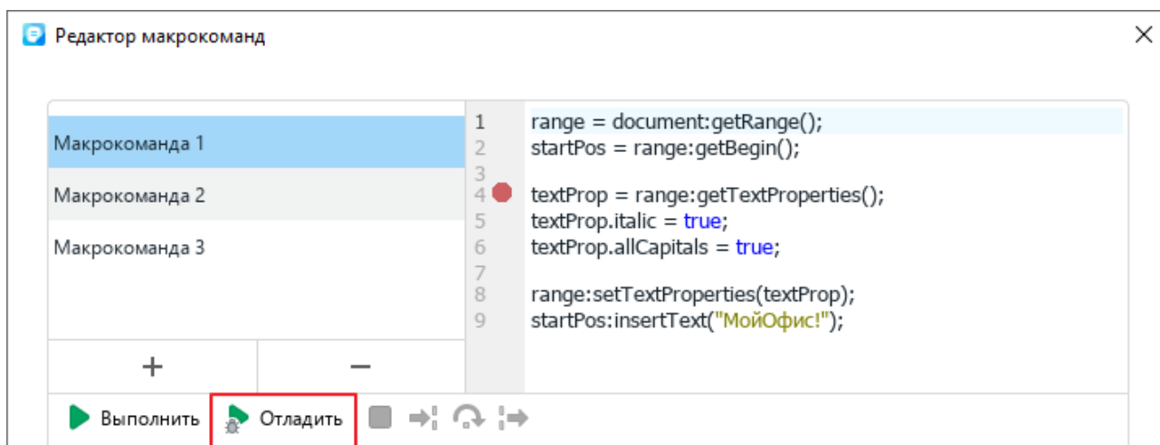
Рисунок 395 – Кнопка Отладить
