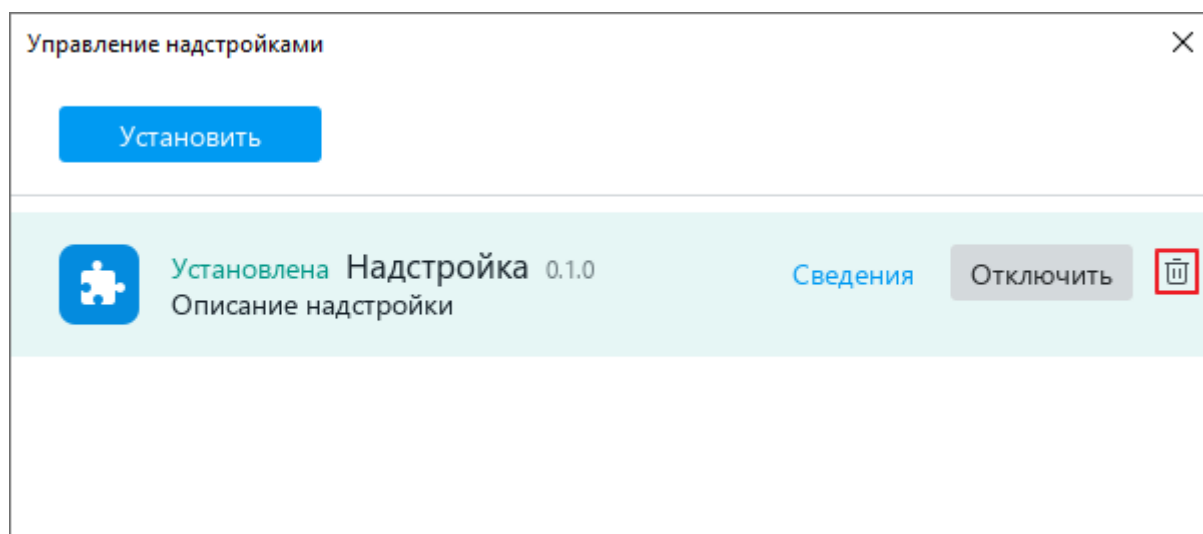
Рисунок 416 – Удаление надстройки
