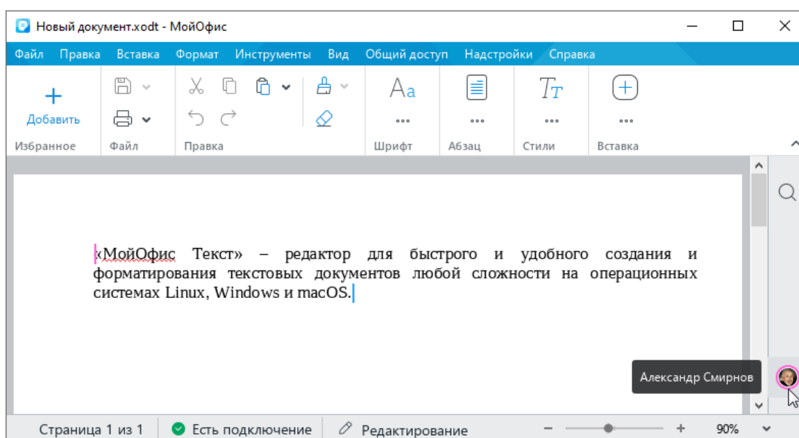
Рисунок 353 – Совместное редактирование
