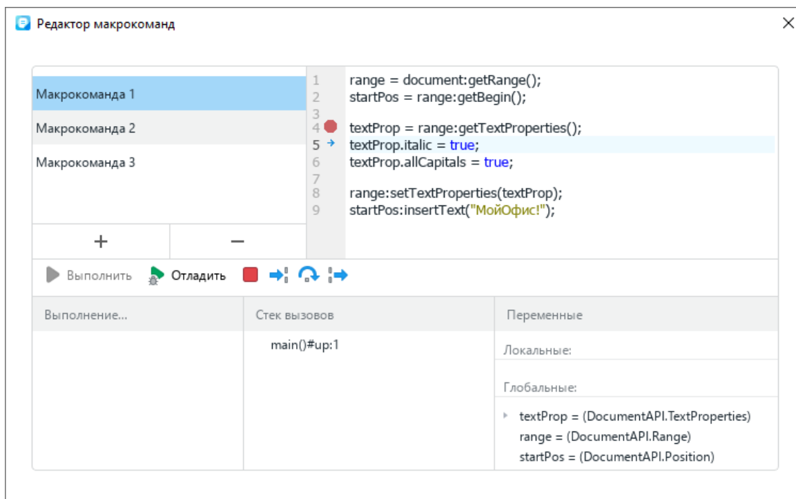
Рисунок 396 – Отладка макроккоманды
