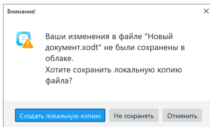
Рисунок 361 – Диалоговое окно
