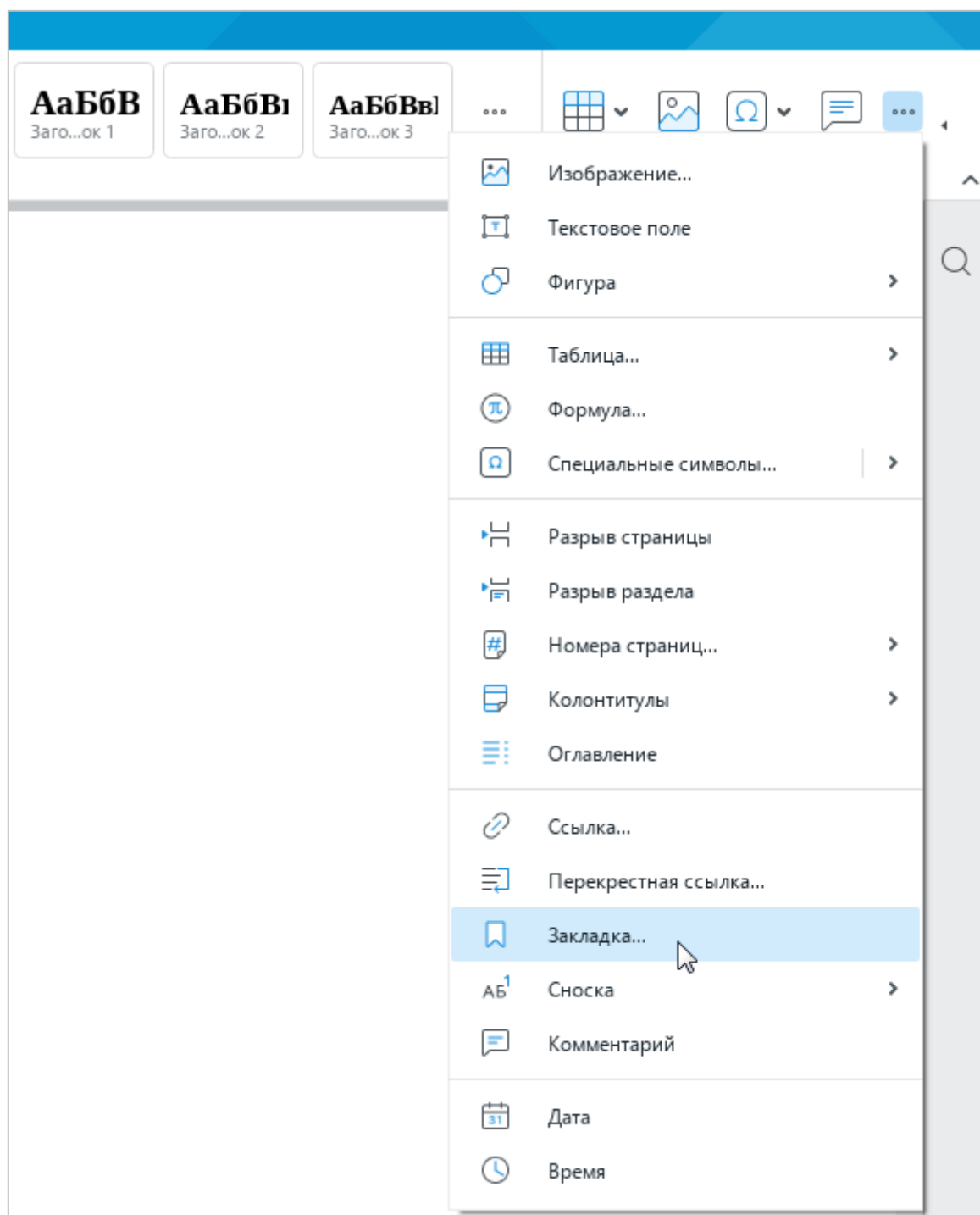
Рисунок 123 – Панель вставки
