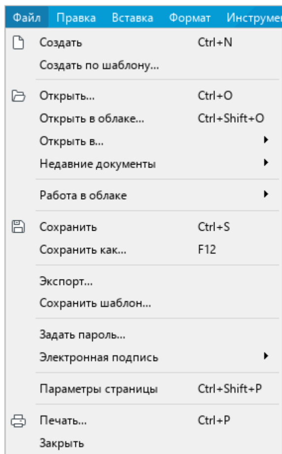
Рисунок 8 – Меню Файл
