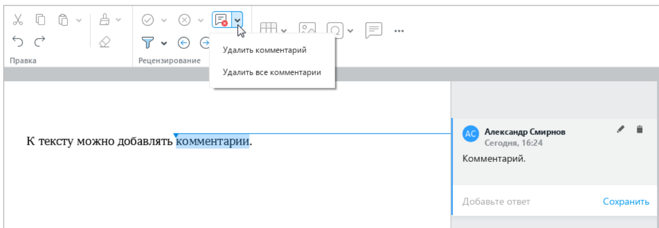
Рисунок 344 – Удаление комментария
