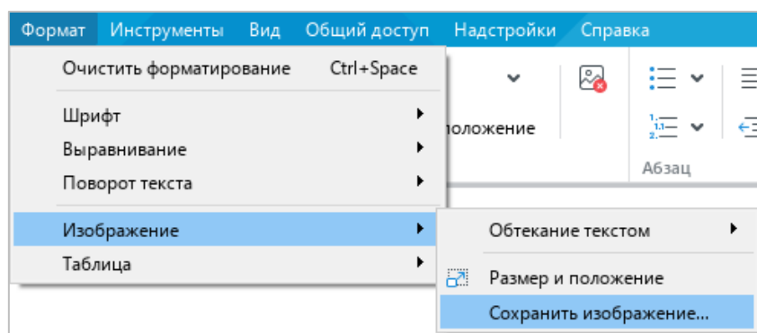
Рисунок 238 – Подменю Изображение
