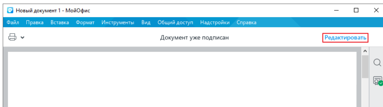
Рисунок 440 – Кнопка Редактировать
