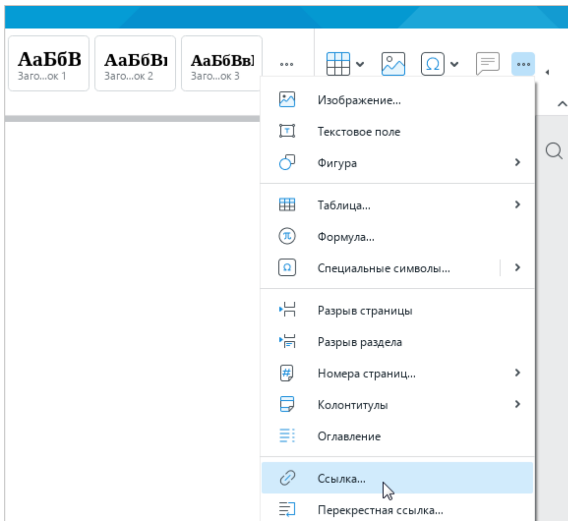
Рисунок 116 – Панель вставки
