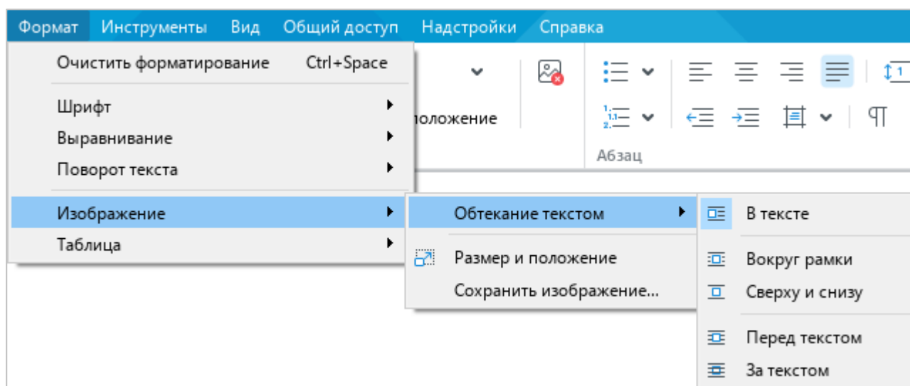
Рисунок 16 – Подменю Изображение
