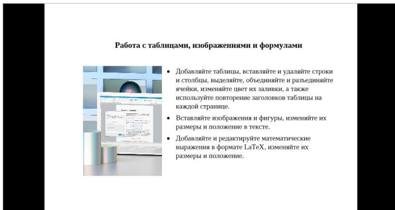
Рисунок 317 – Режим презентации
