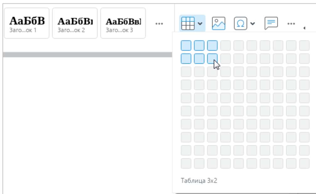
Рисунок 189 – Кнопка Таблица
