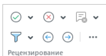
Рисунок 77 – Раздел Рецензирование
