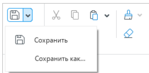
Рисунок 43 – Команды сохранения
