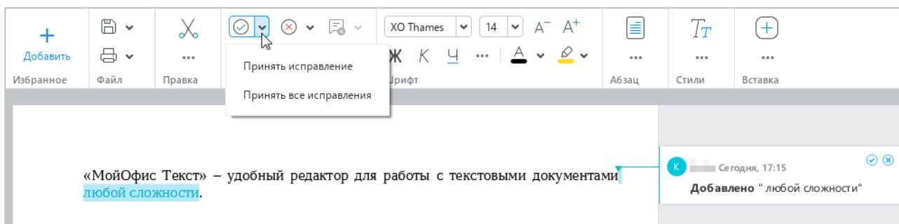
Рисунок 323 – Принятие исправлений
