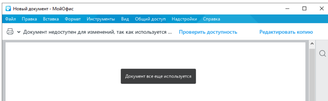
Рисунок 95 – Всплывающее сообщение
