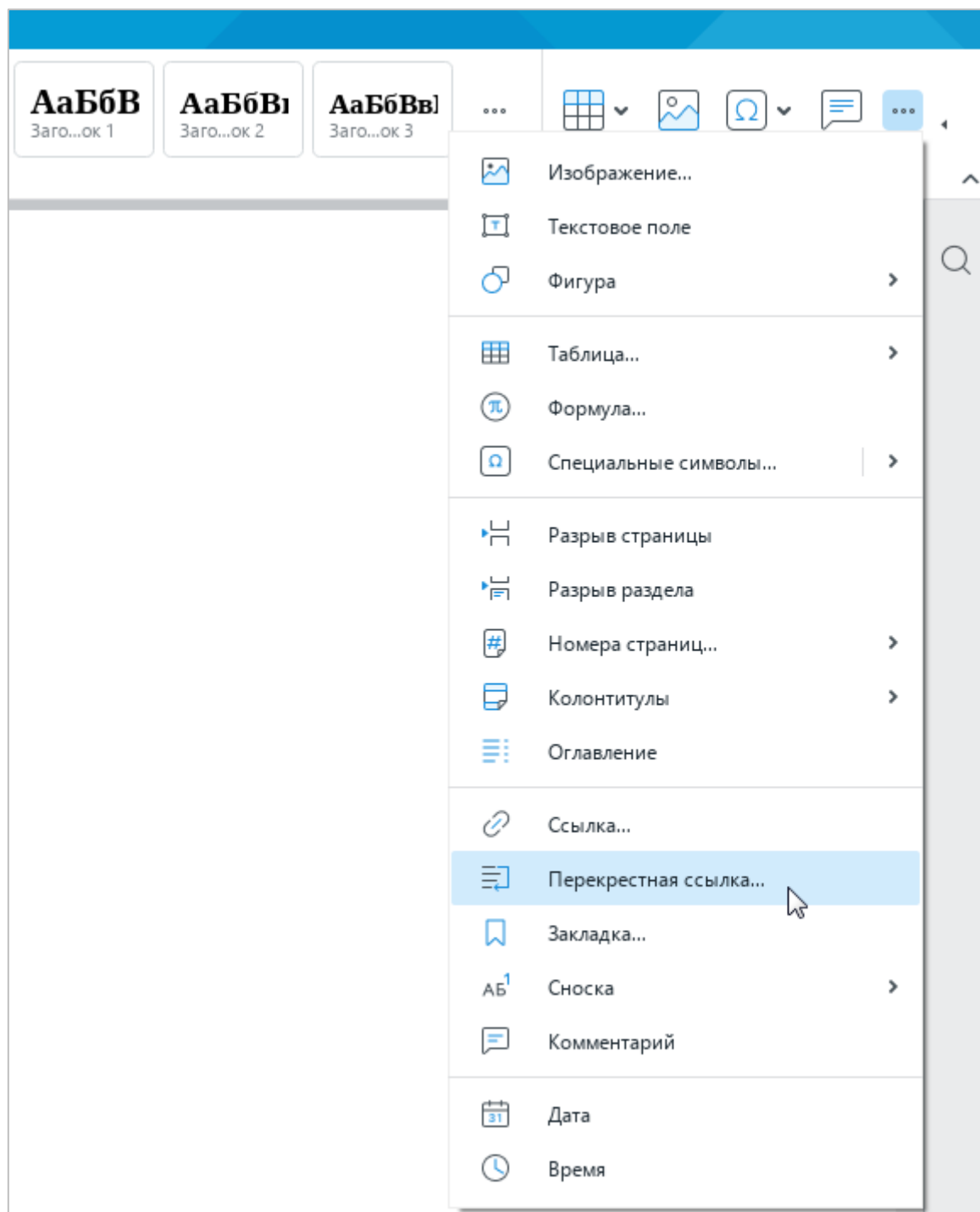
Рисунок 120 – Панель вставки
