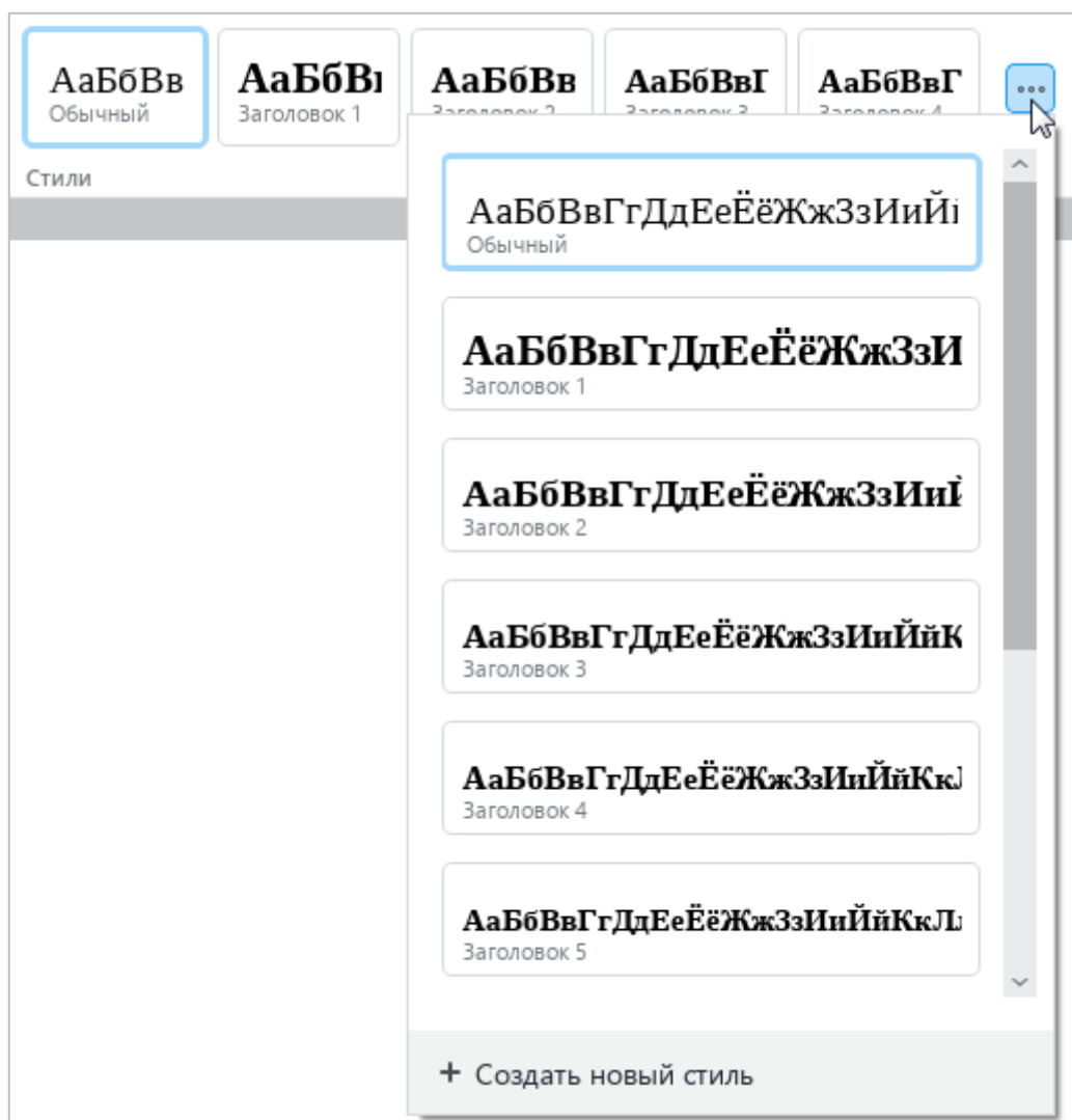
Рисунок 299 – Список стилей
