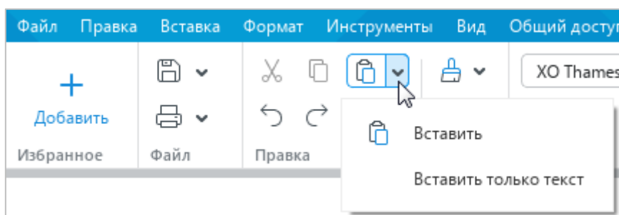
Рисунок 270 – Кнопка Вставить
