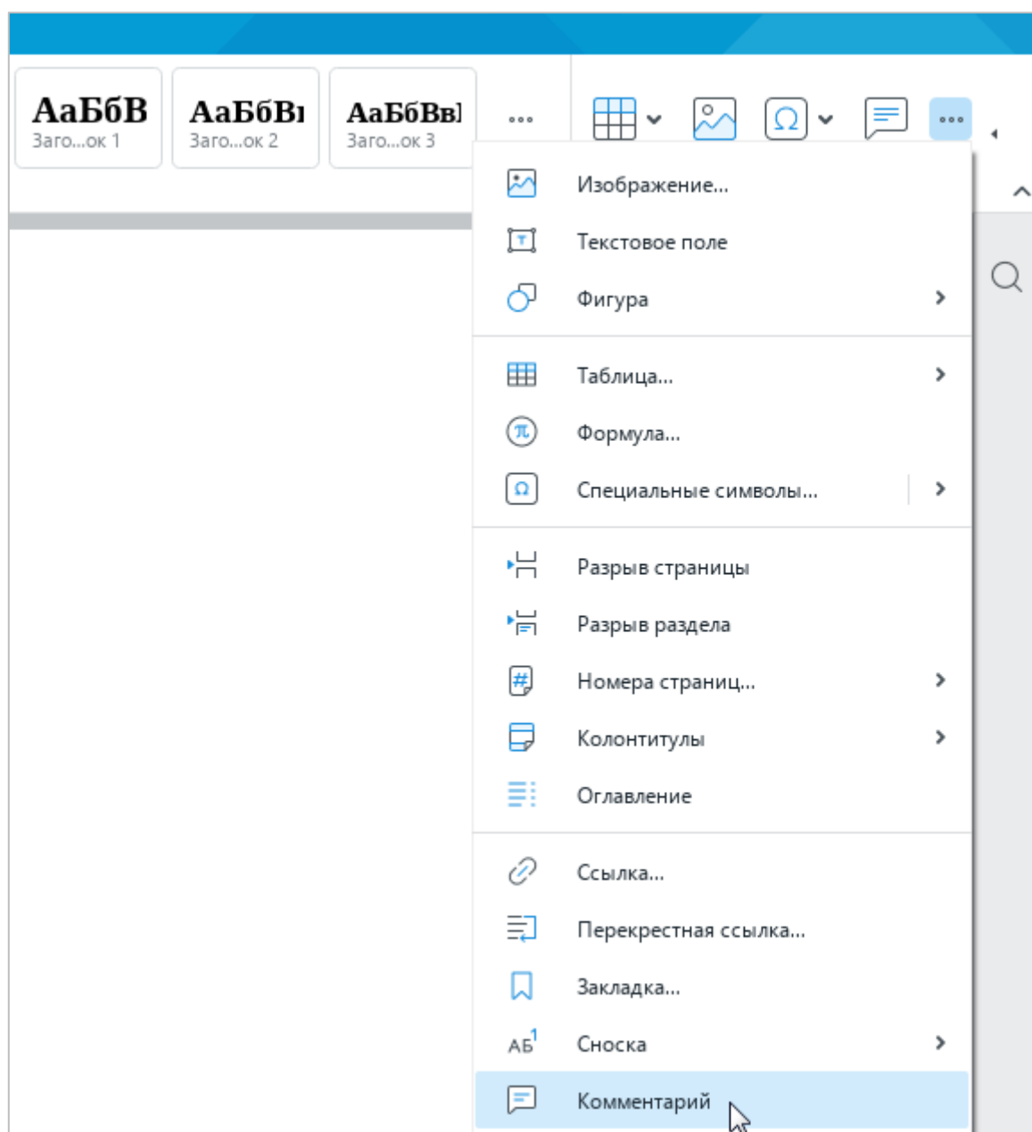
Рисунок 332 – Панель вставки
