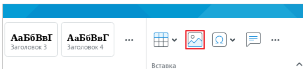
Рисунок 221 – Кнопка Изображение
