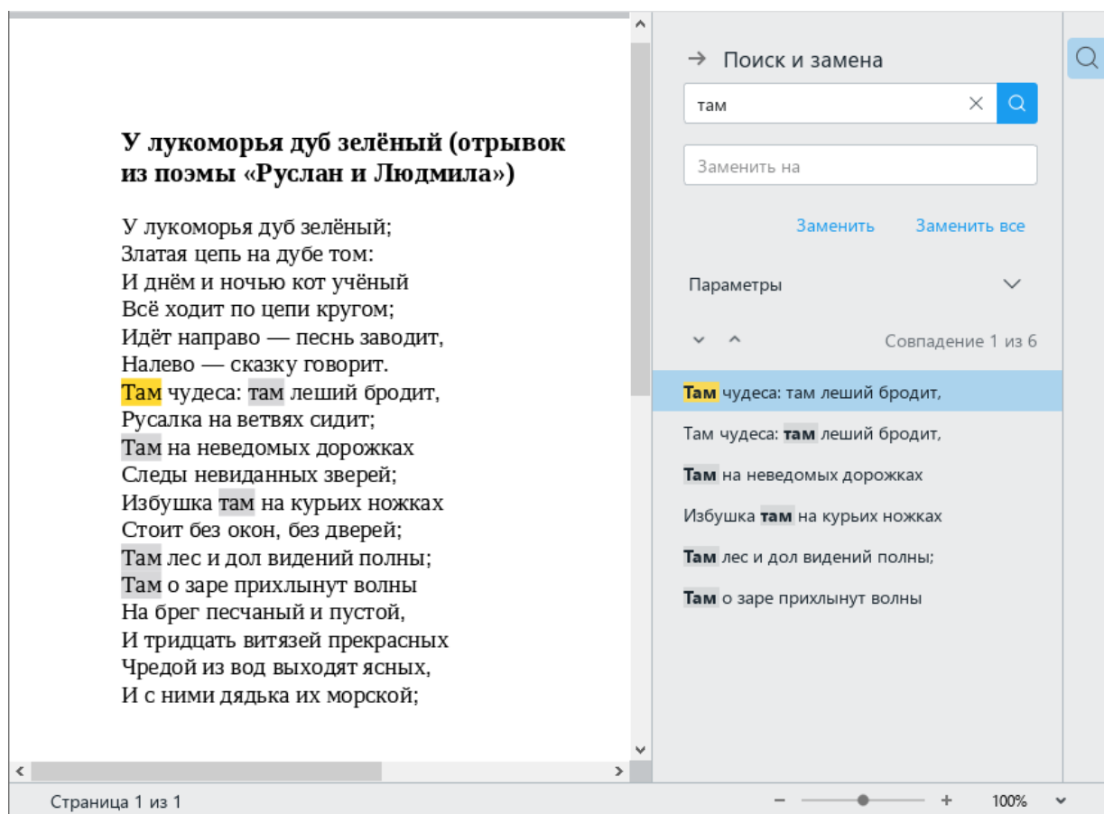
Рисунок 150 – Найденные совпадения
