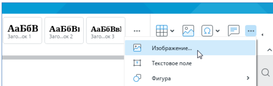
Рисунок 222 – Панель вставки
