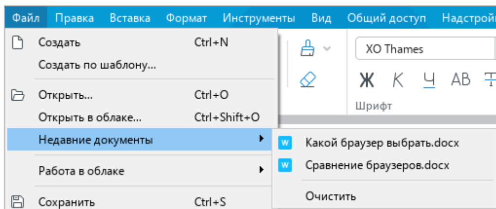
Рисунок 96 – Недавние документы
