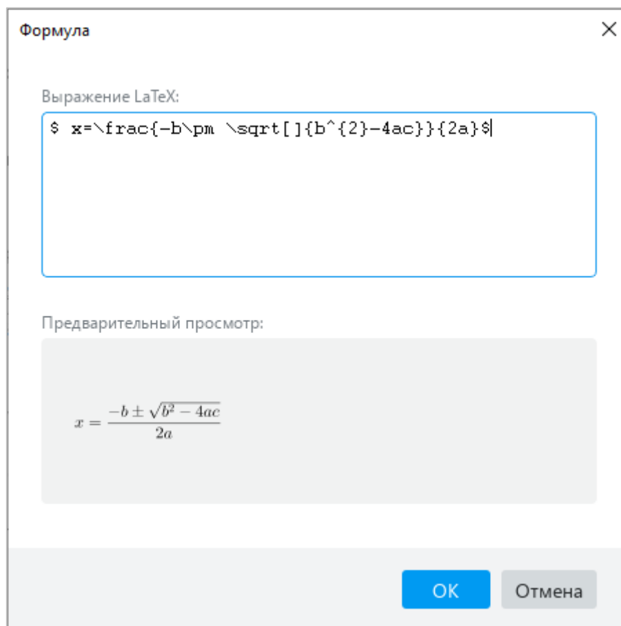
Рисунок 263 – Окно Формула
