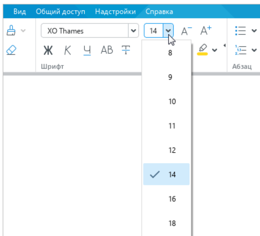
Рисунок 161 – Размер шрифта
