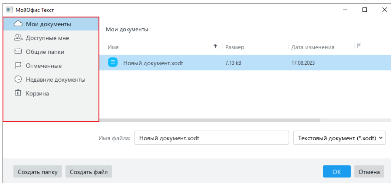
Рисунок 352 – Облачное хранилище
