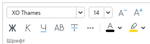
Рисунок 48 – Раздел Шрифт
