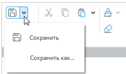
Рисунок 98 – Кнопка Сохранить
