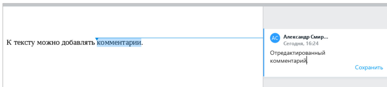
Рисунок 341 – Поле комментария
