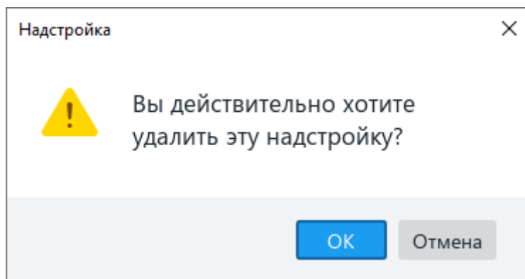
Рисунок 417 – Диалоговое окно
