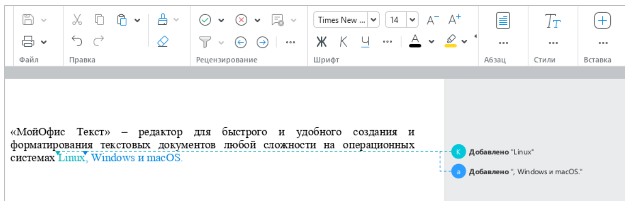
Рисунок 319 – Исправления
