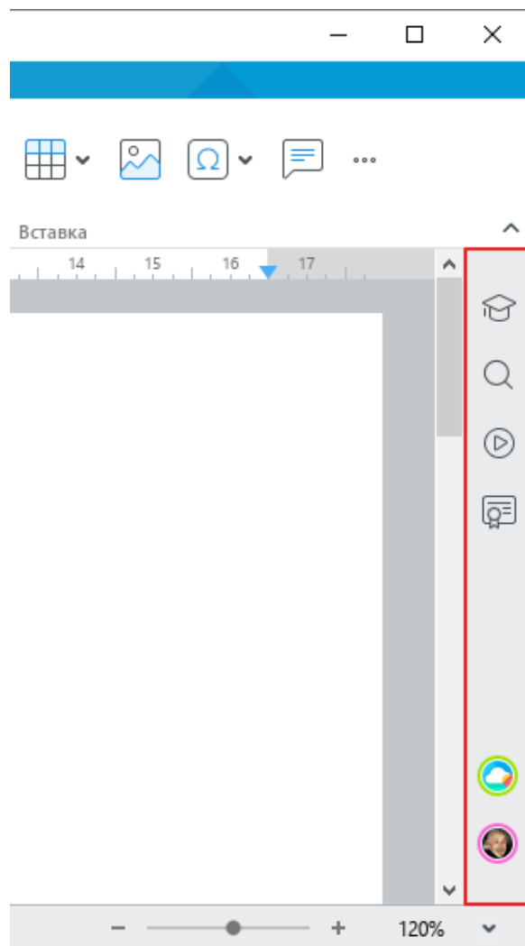
Рисунок 84 – Боковая панель
