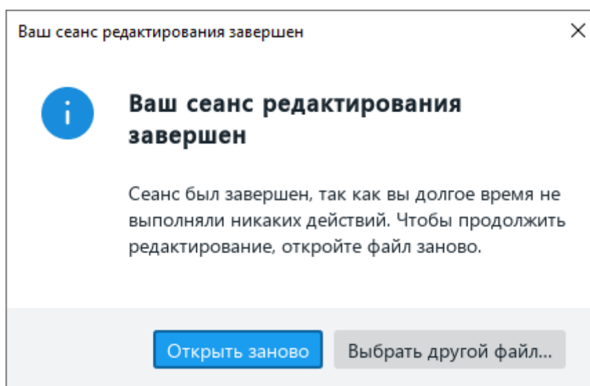
Рисунок 360 – Диалоговое окно
