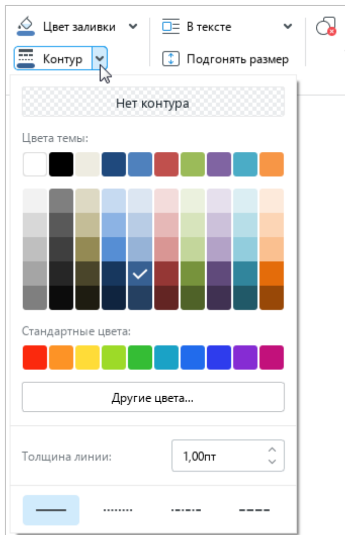
Рисунок 70 – Кнопка Контур
