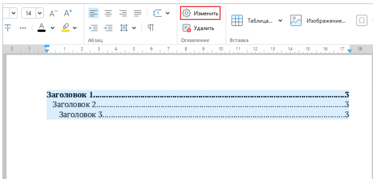
Рисунок 302 – Кнопка Изменить
