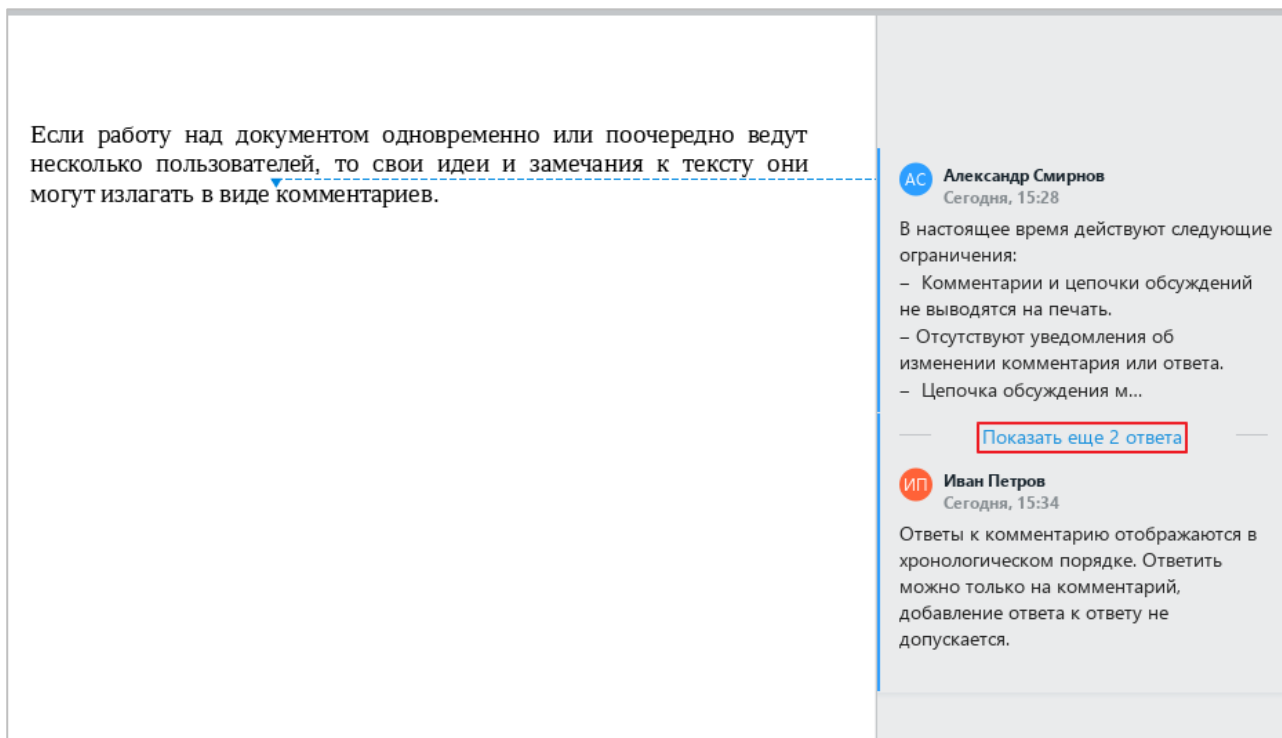
Рисунок 336 – Цепочка
