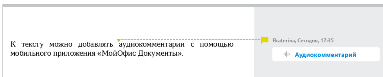
Рисунок 348 – Аудиокомментарий
