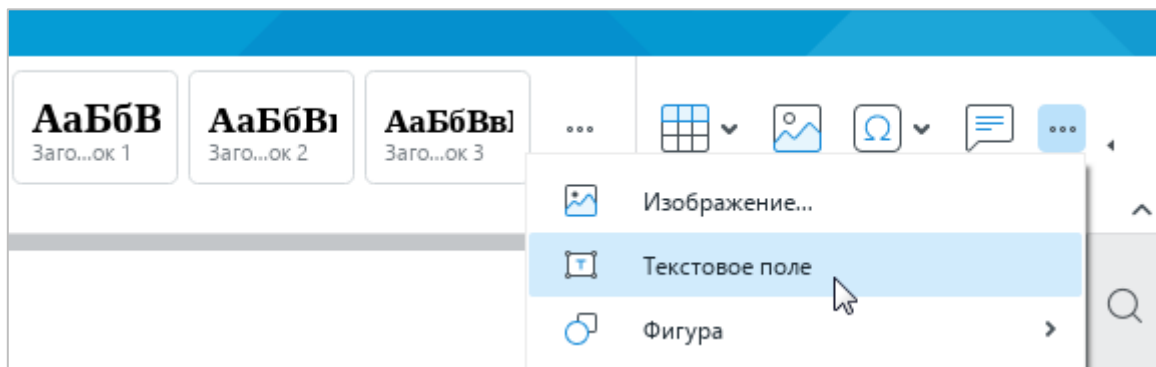
Рисунок 243 – Панель вставки
