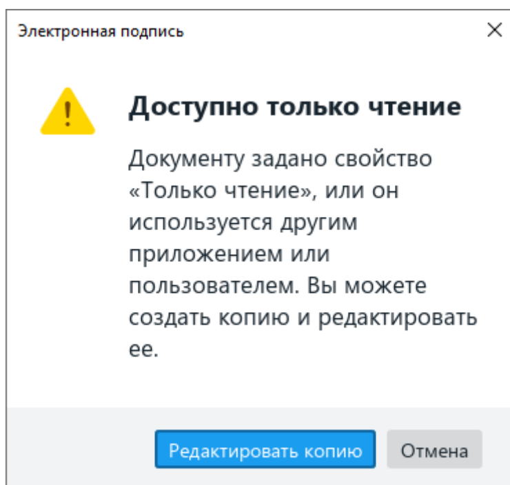
Рисунок 446 – Диалоговое окно
