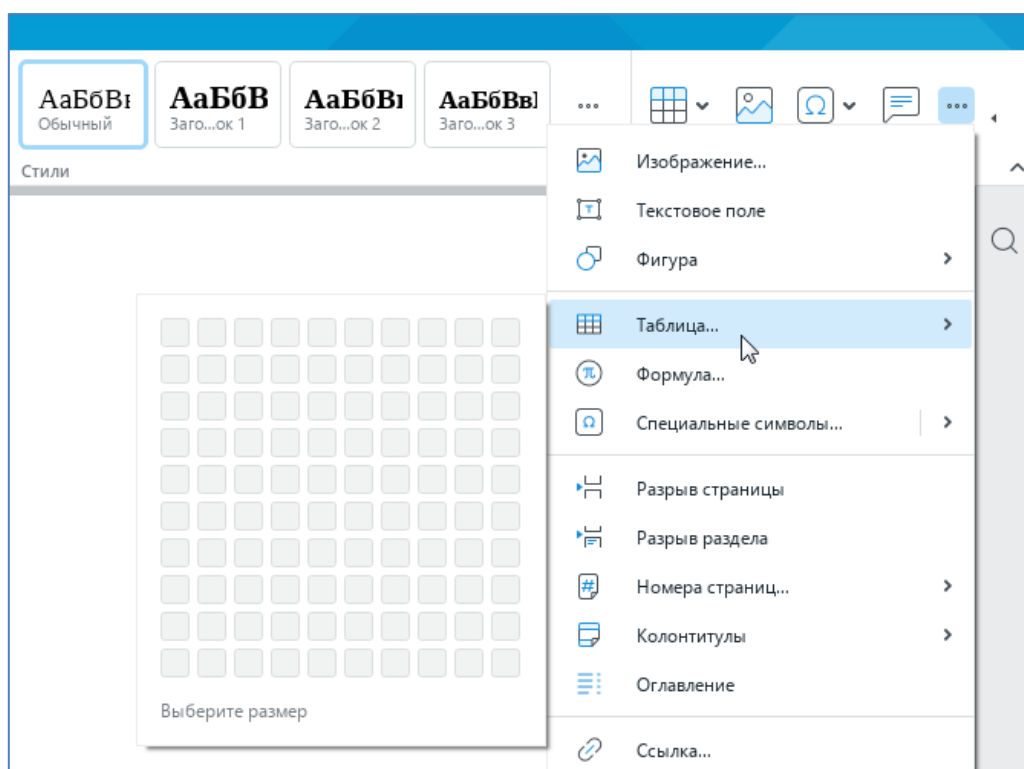
Рисунок 190 – Панель вставки
