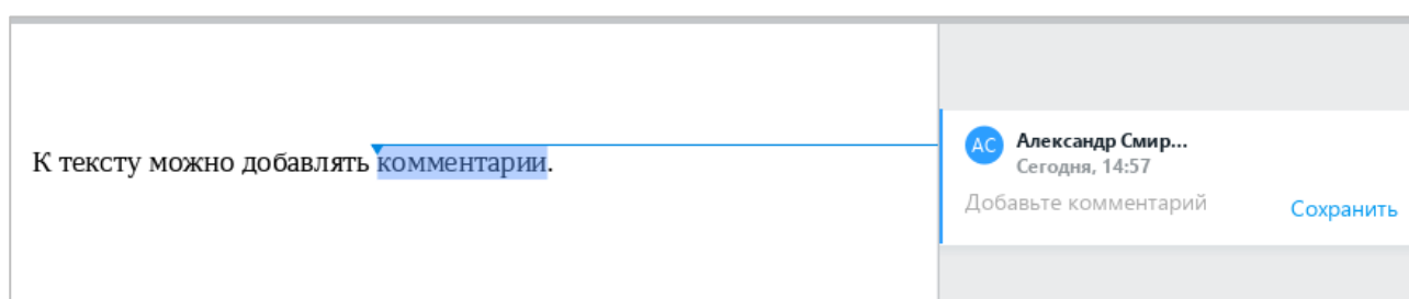
Рисунок 333 – Добавление комментария
