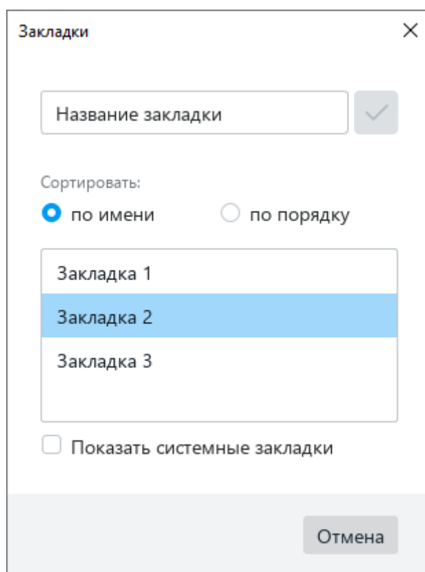
Рисунок 128 – Окно Закладки
