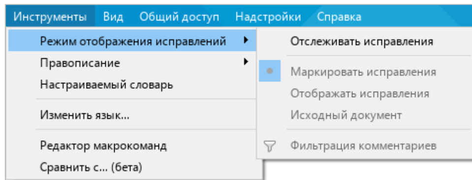
Рисунок 18 – Меню Инструменты
