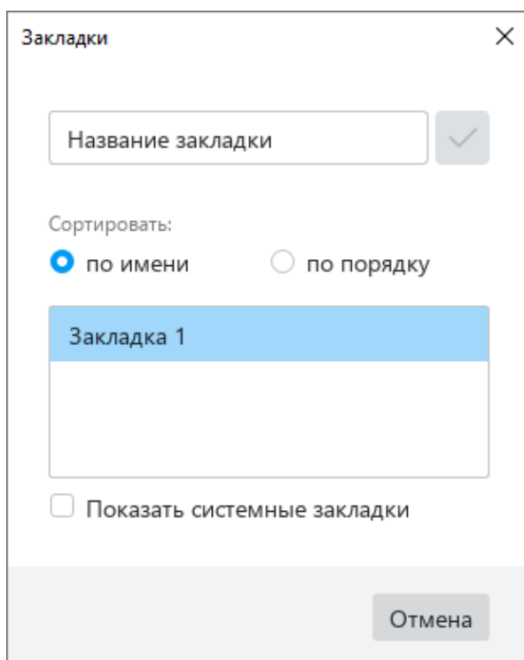
Рисунок 125 – Закладка добавлена
