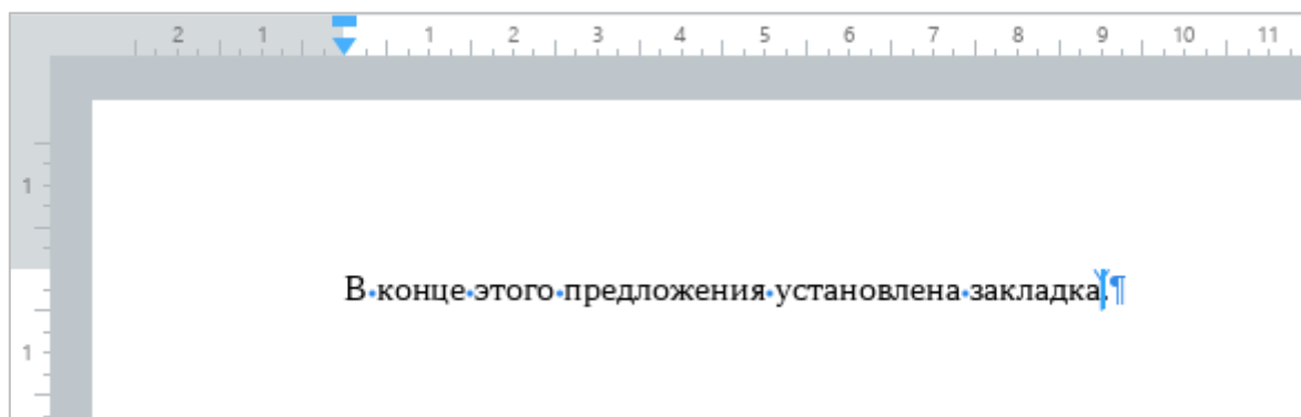
Рисунок 126 – Отображение закладки
