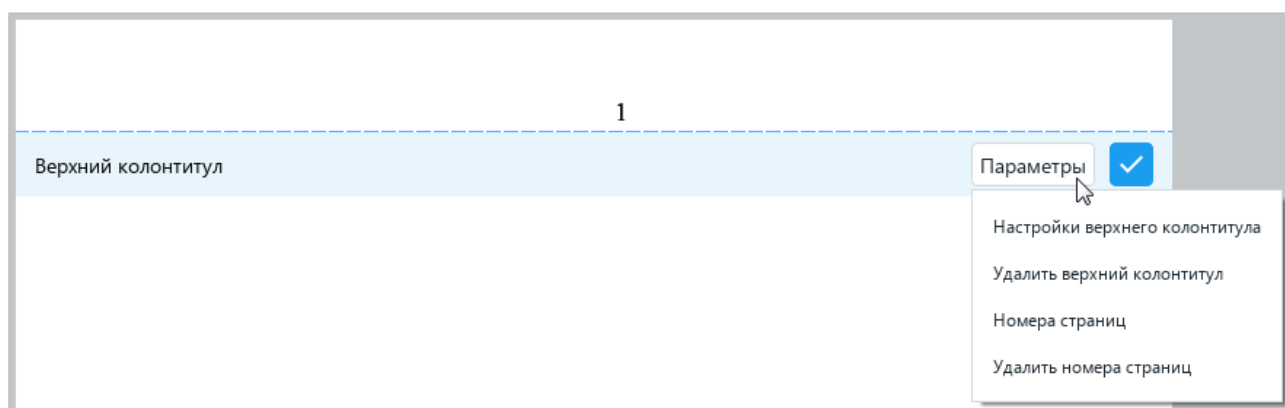
Рисунок 293 –Кнопка Параметры
