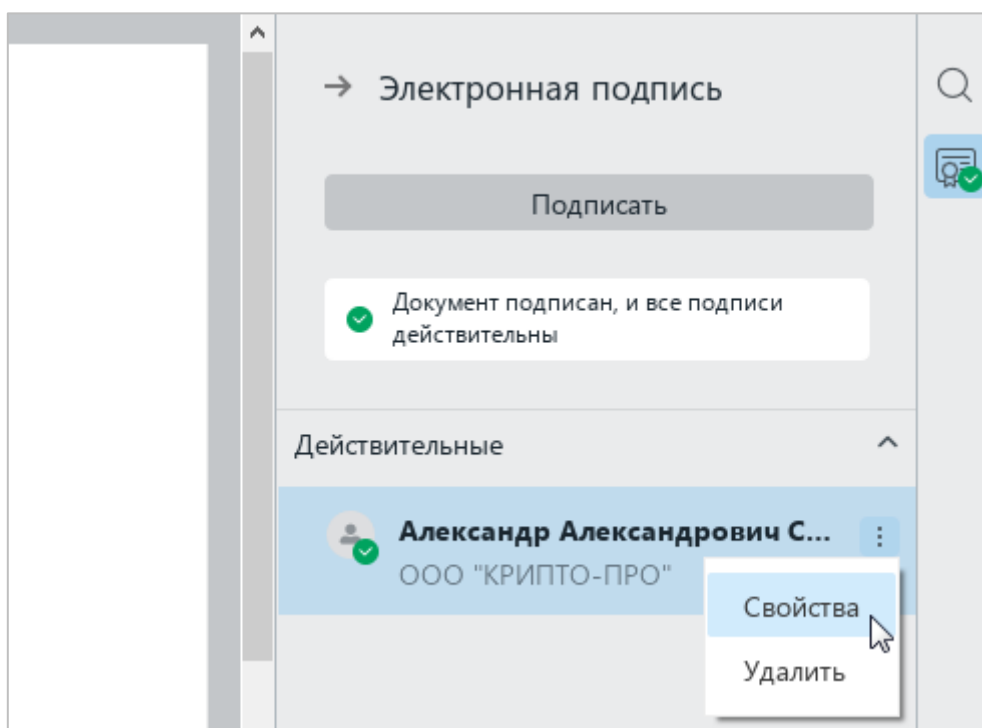
Рисунок 438 – Команда Свойства
