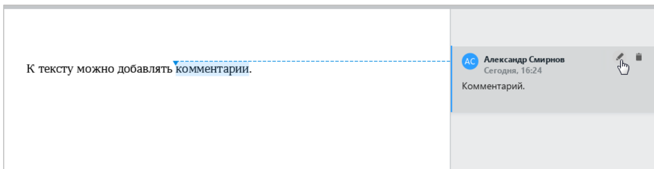
Рисунок 340 – Кнопка Редактировать
