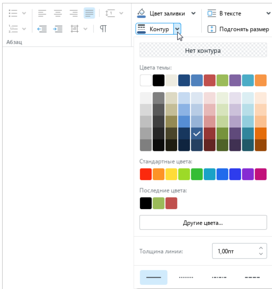
Рисунок 247 – Кнопка Контур
