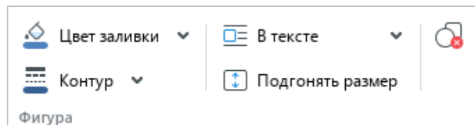
Рисунок 68 – Раздел Фигура
