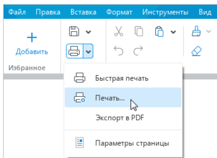
Рисунок 104 – Команда Печать
