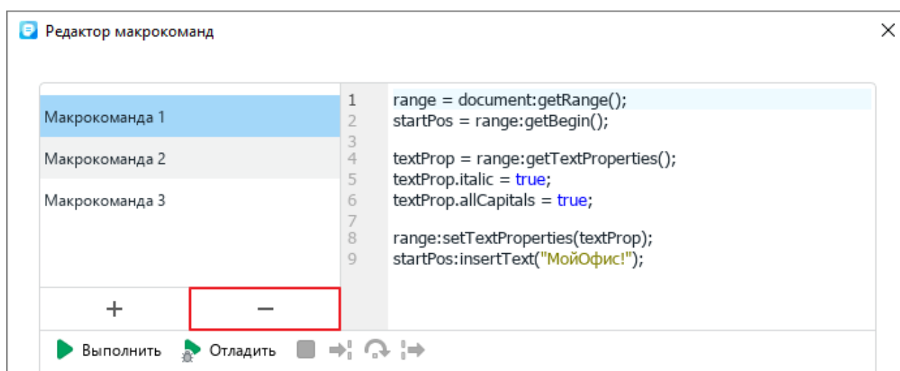
Рисунок 399 – Удаление макрокоманды
