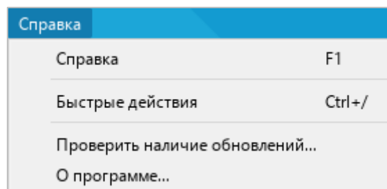
Рисунок 25 – Меню Справка
