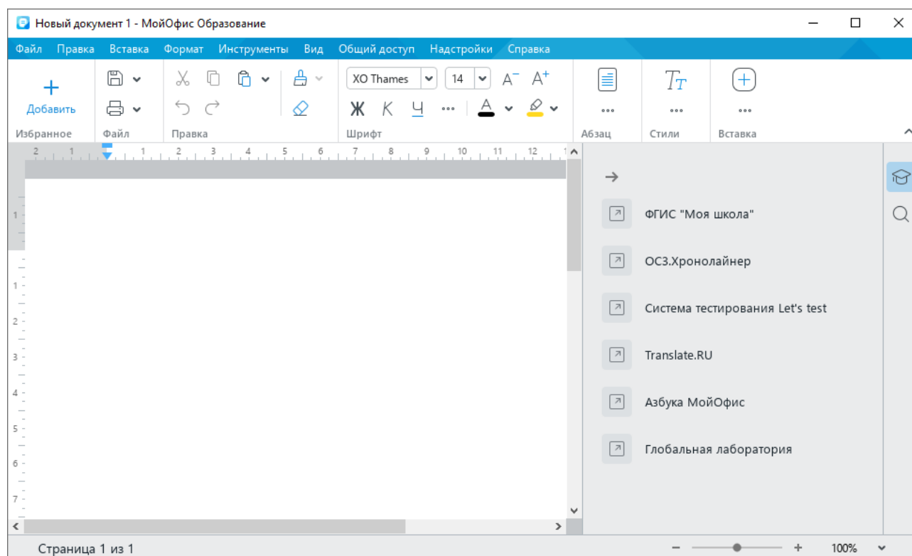
Рисунок 447 – Панель Образование
