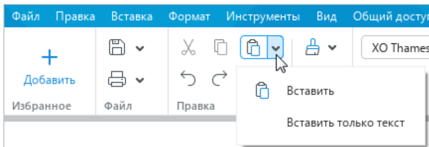
Рисунок 224 – Кнопка Вставить
