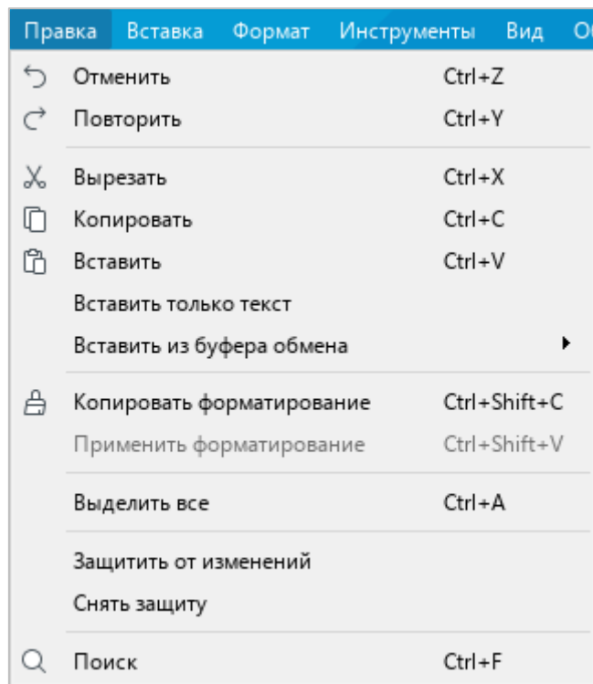
Рисунок 11 – Меню Правка
