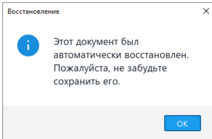
Рисунок 99 – Диалоговое окно
