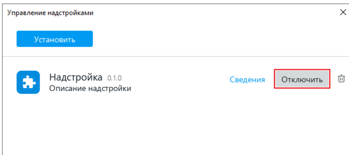
Рисунок 409 – Отключение надстройки
