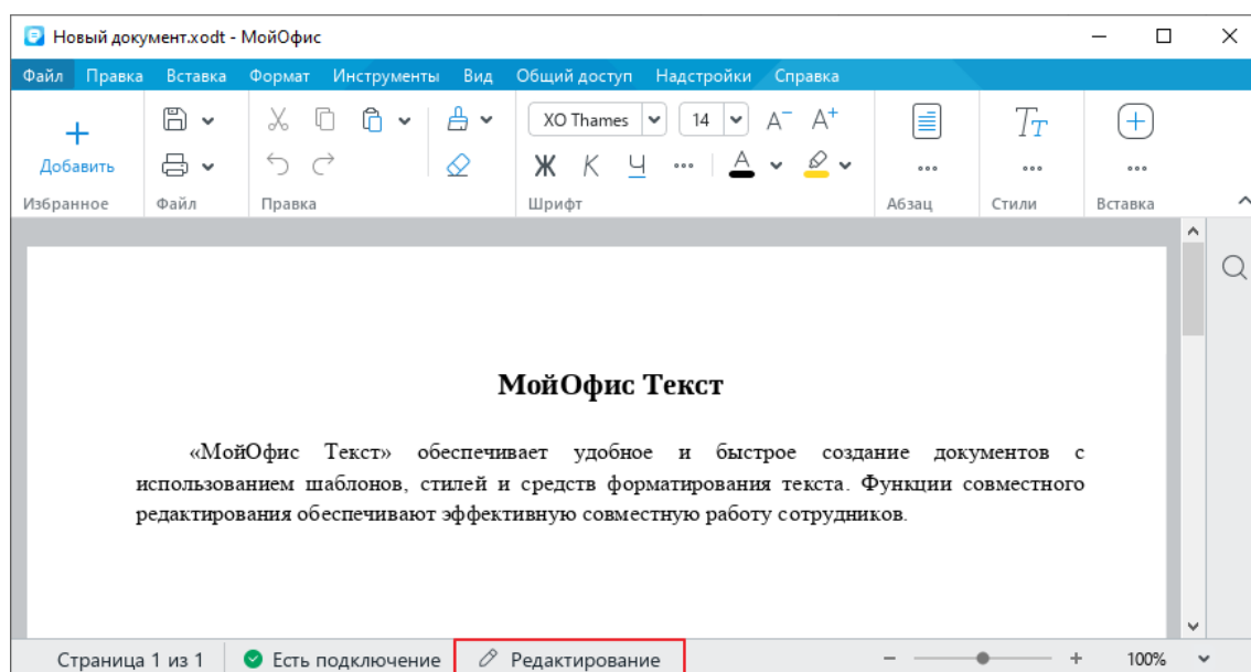
Рисунок 358 – Уровень доступа
