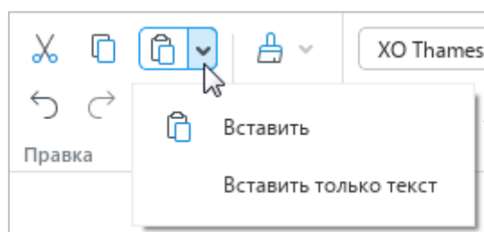
Рисунок 46 – Команды вставки
