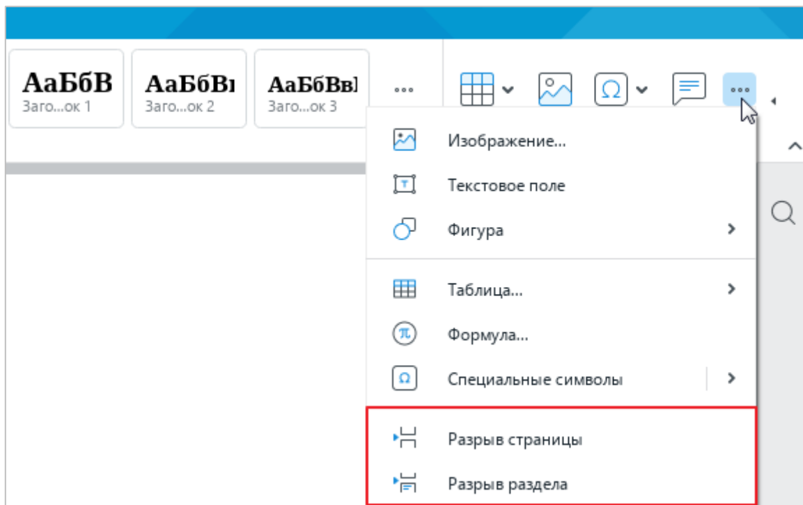
Рисунок 297 – Панель вставки
