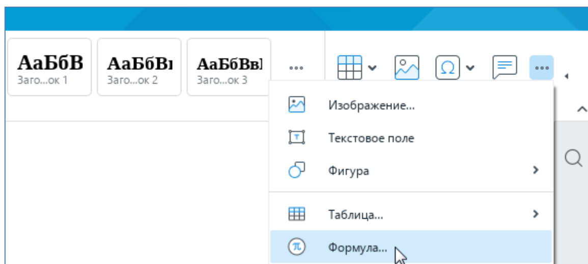
Рисунок 262 – Панель вставки
