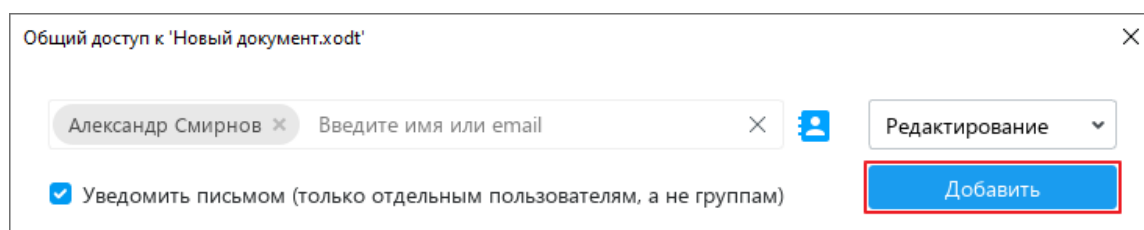
Рисунок 373 – Кнопка Добавить
