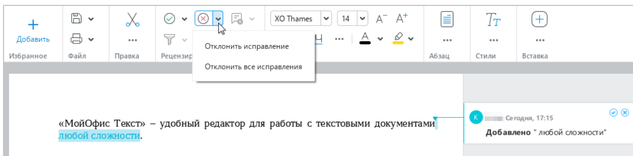
Рисунок 324 – Отклонение исправлений
