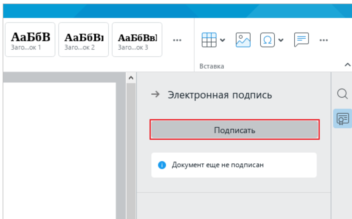
Рисунок 428 – Кнопка Подписать
