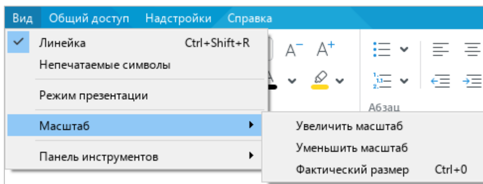
Рисунок 21 – Подменю Масштаб
