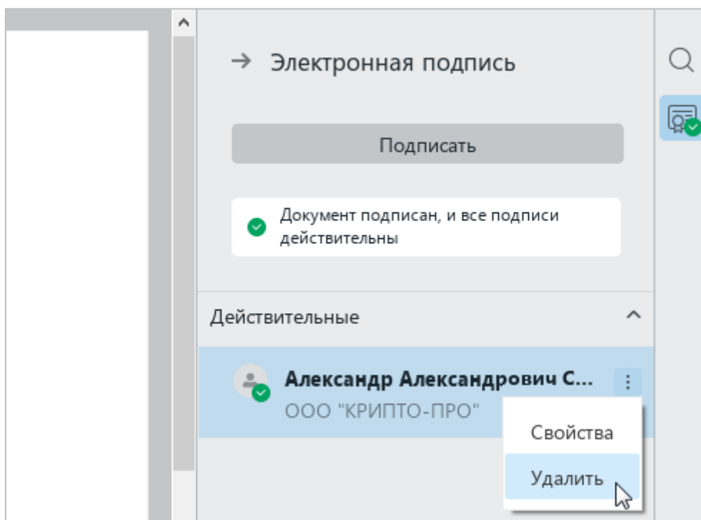
Рисунок 444 – Команда Удалить
