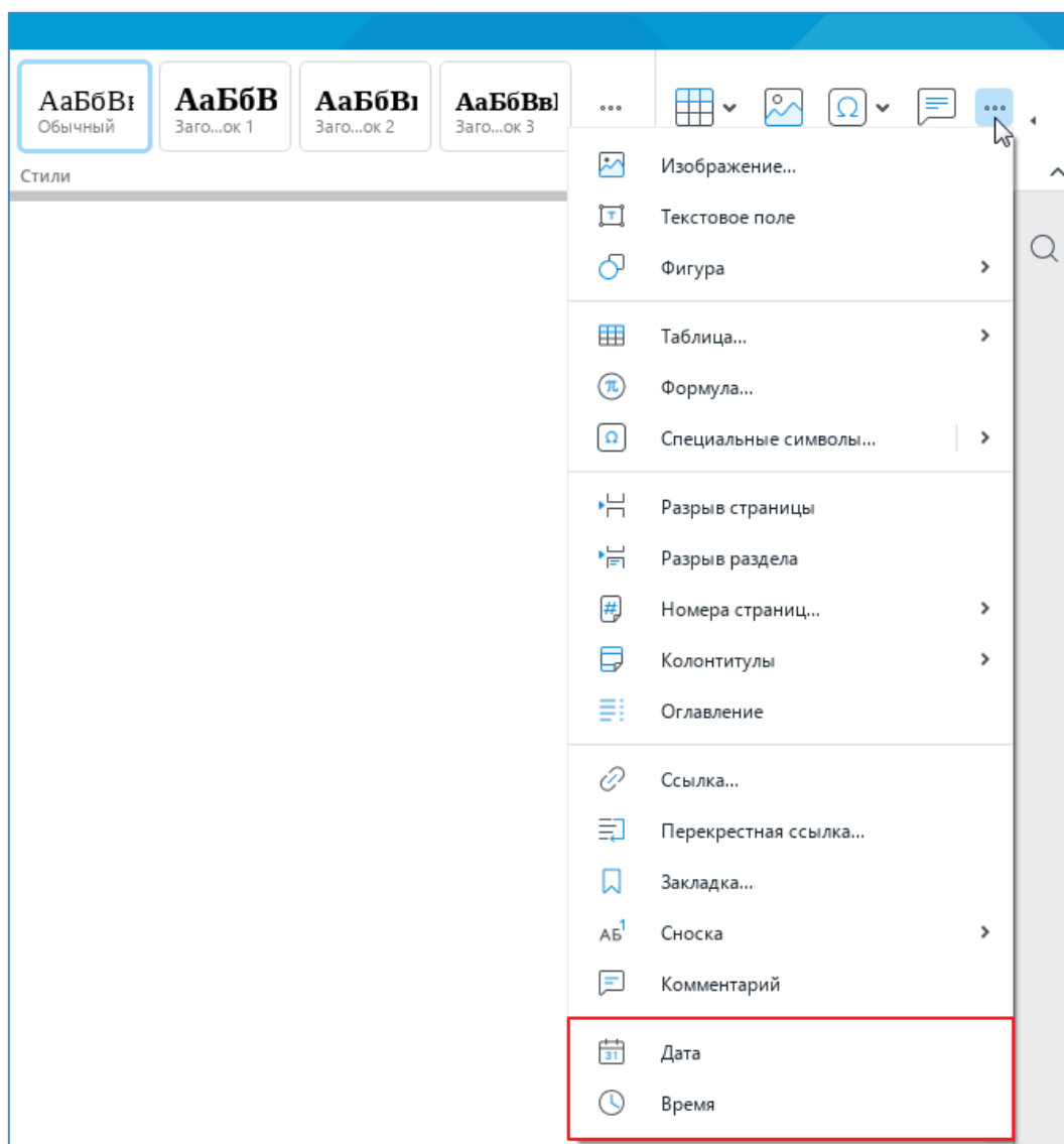
Рисунок 139 – Панель вставки
