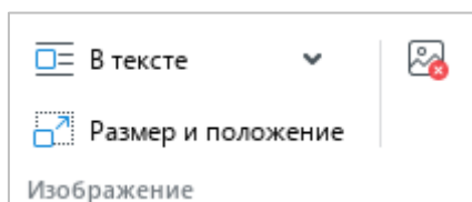
Рисунок 66 – Раздел Изображение
