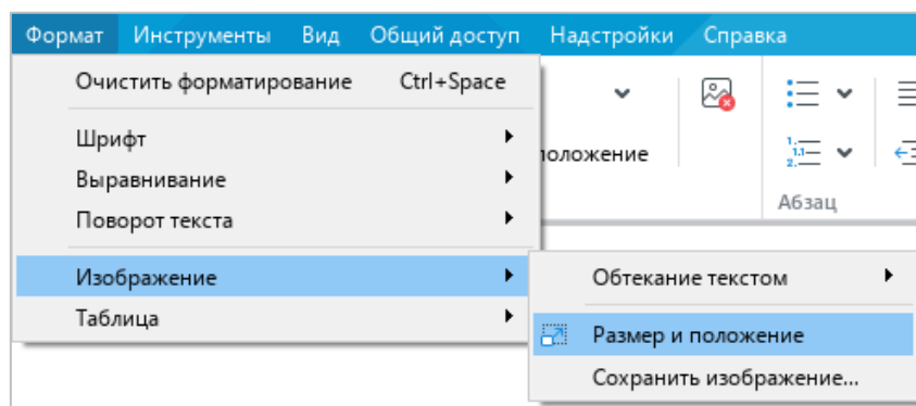
Рисунок 235 – Подменю Изображение
