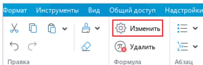
Рисунок 264 – Кнопка Изменить
