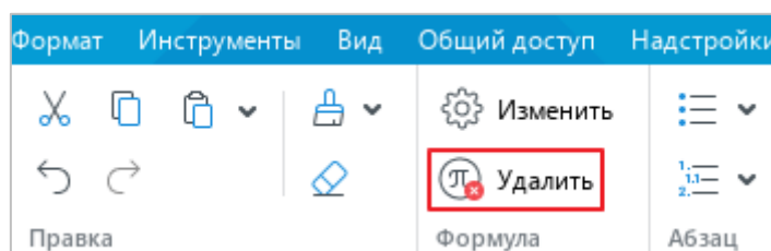
Рисунок 266 – Кнопка Удалить
