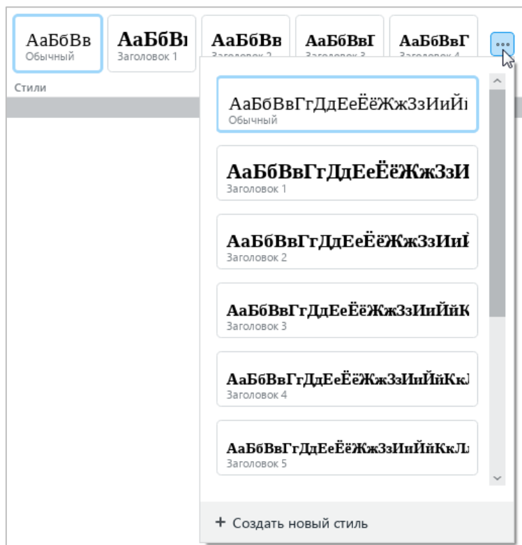
Рисунок 153 – Список стилей
