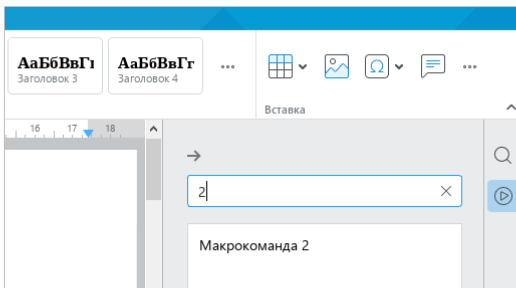
Рисунок 387 – Поиск макросов
