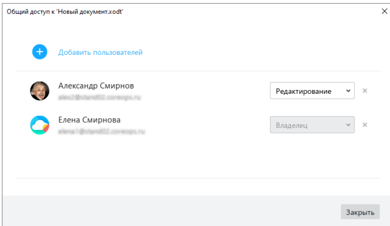
Рисунок 374 – Список пользователей
