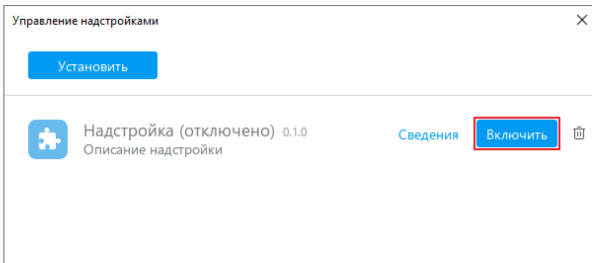
Рисунок 410 – Включение надстройки
