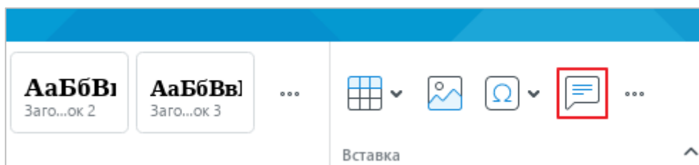
Рисунок 331 – Кнопка Комментарий
