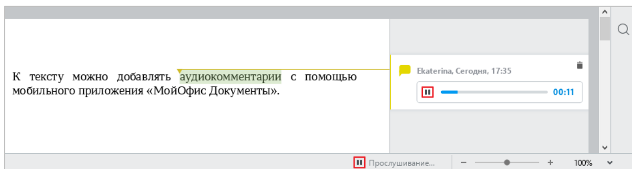
Рисунок 349 – Прослушивание аудиокomentarия
