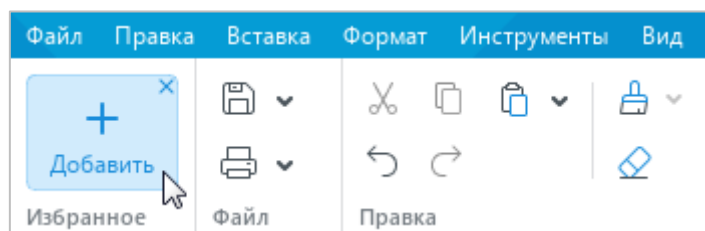
Рисунок 36 – Кнопка Добавить
