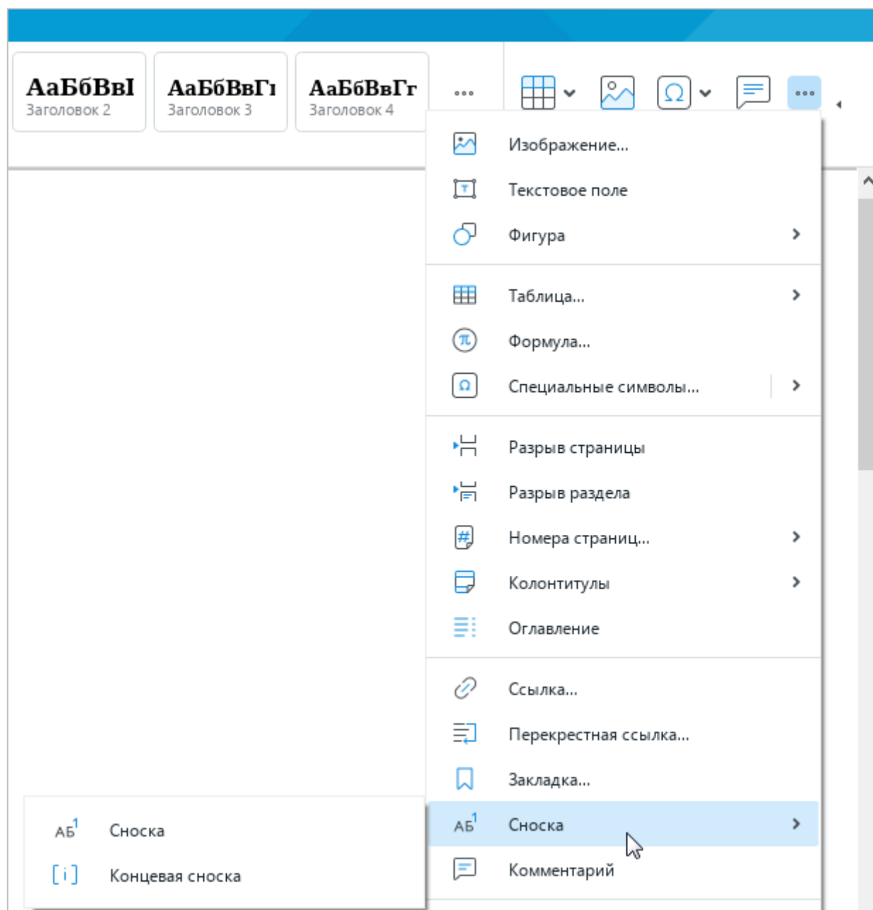
Рисунок 110 – Панель вставки
