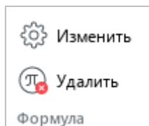
Рисунок 76 – Раздел Формула
