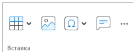
Рисунок 61 – Раздел Вставка
