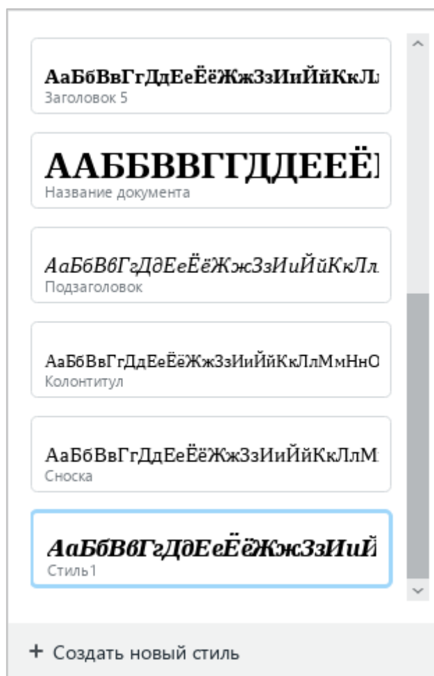
Рисунок 157 – Пользовательский стиль
