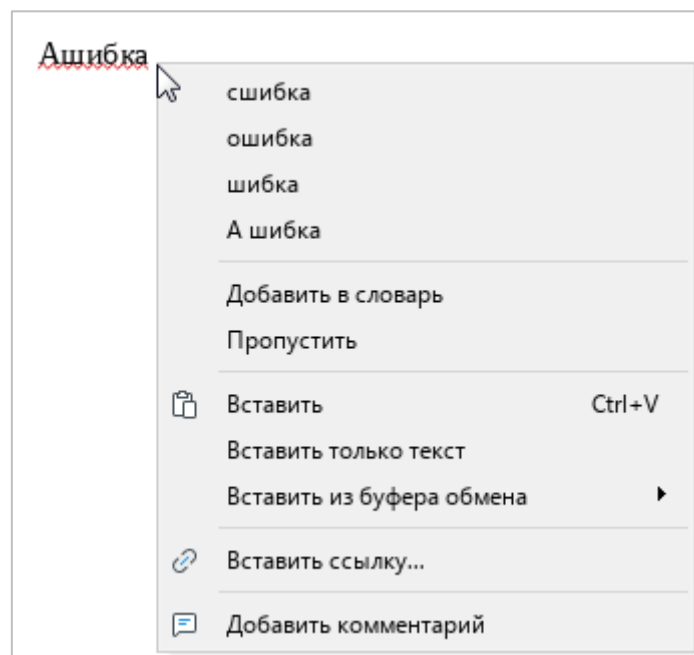
Рисунок 141 – Проверка правописания
