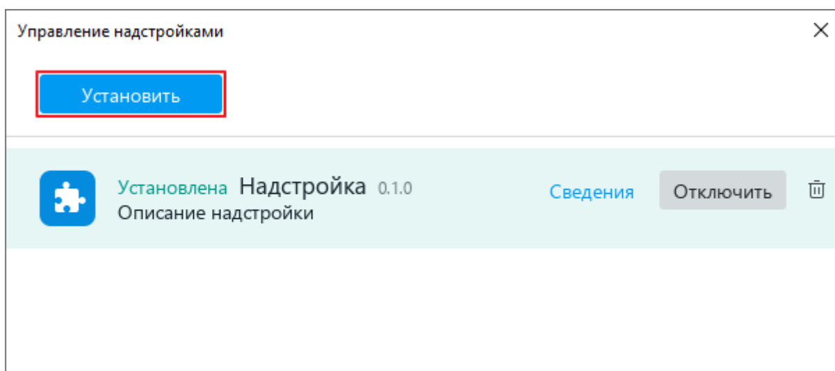
Рисунок 411 – Кнопка Установить
