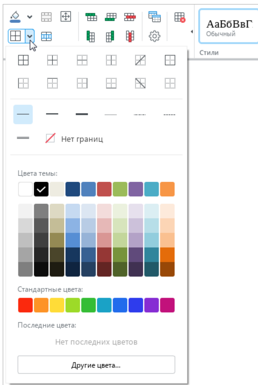
Рисунок 65 – Настройка границ
