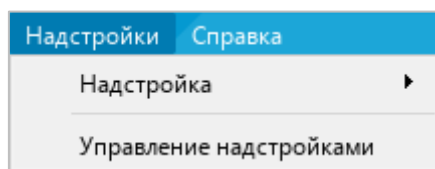
Рисунок 24 – Меню Надстройки
