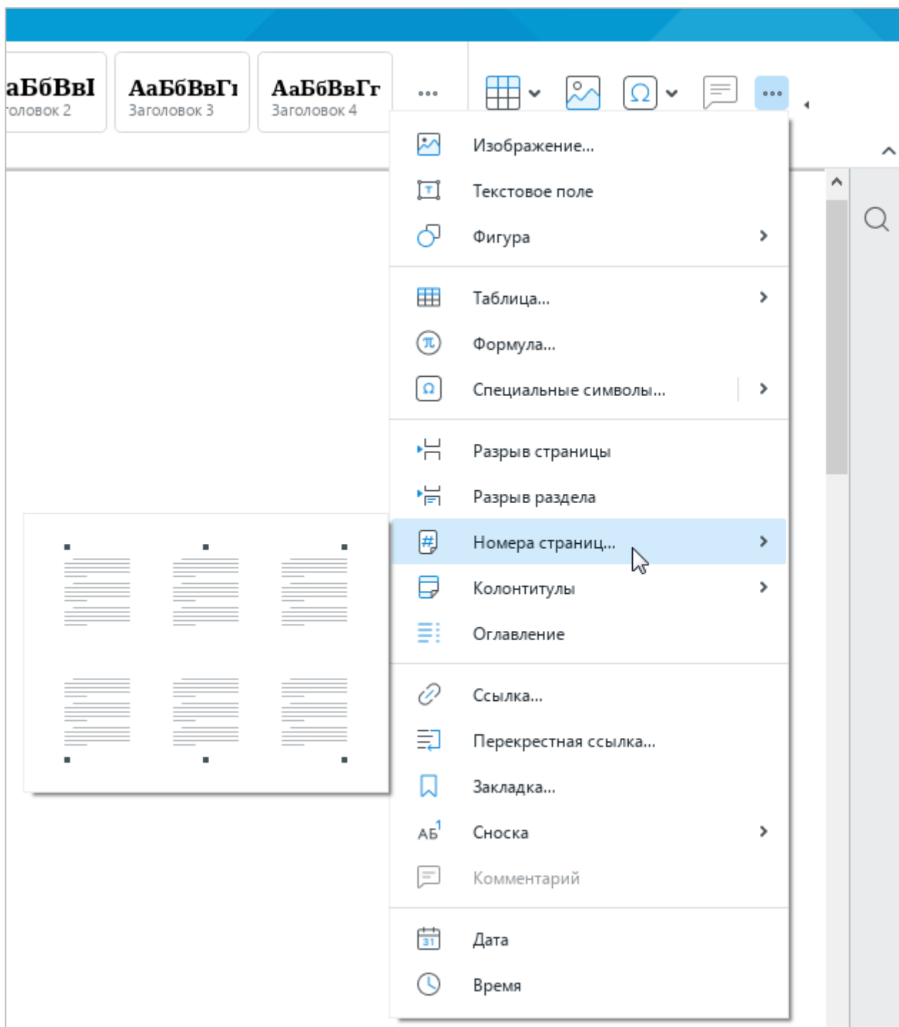
Рисунок 287 – Панель вставки
