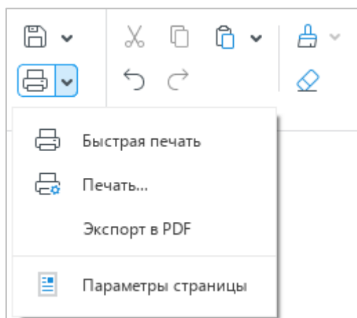
Рисунок 44 – Команды печати
