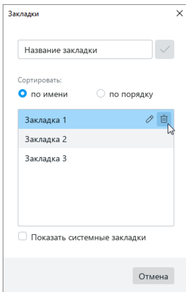
Рисунок 130 – Удаление закладки
