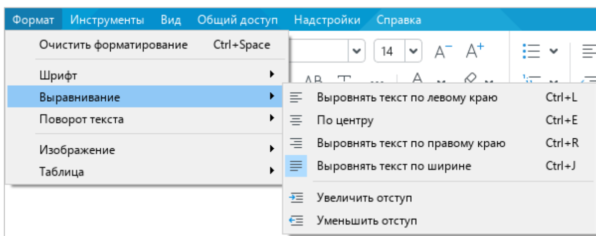
Рисунок 14 – Подменю Выравнивание
