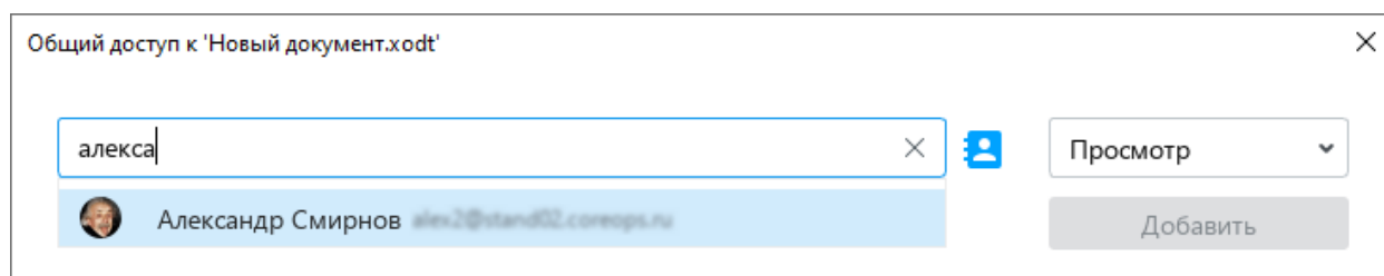
Рисунок 371 – Поиск пользователя
