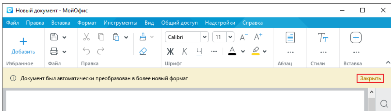
Рисунок 92 – Кнопка Заккрыть
