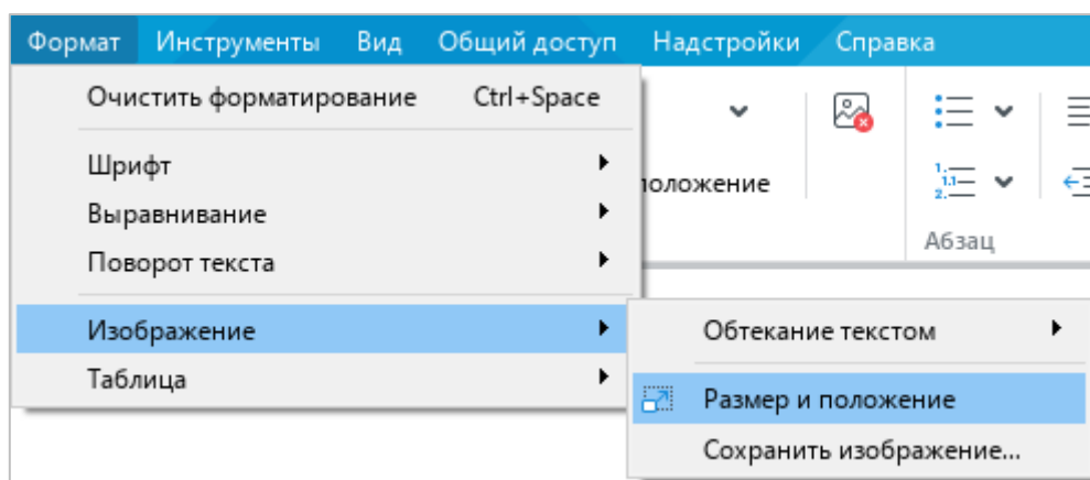
Рисунок 230 – Подменю Изображение
