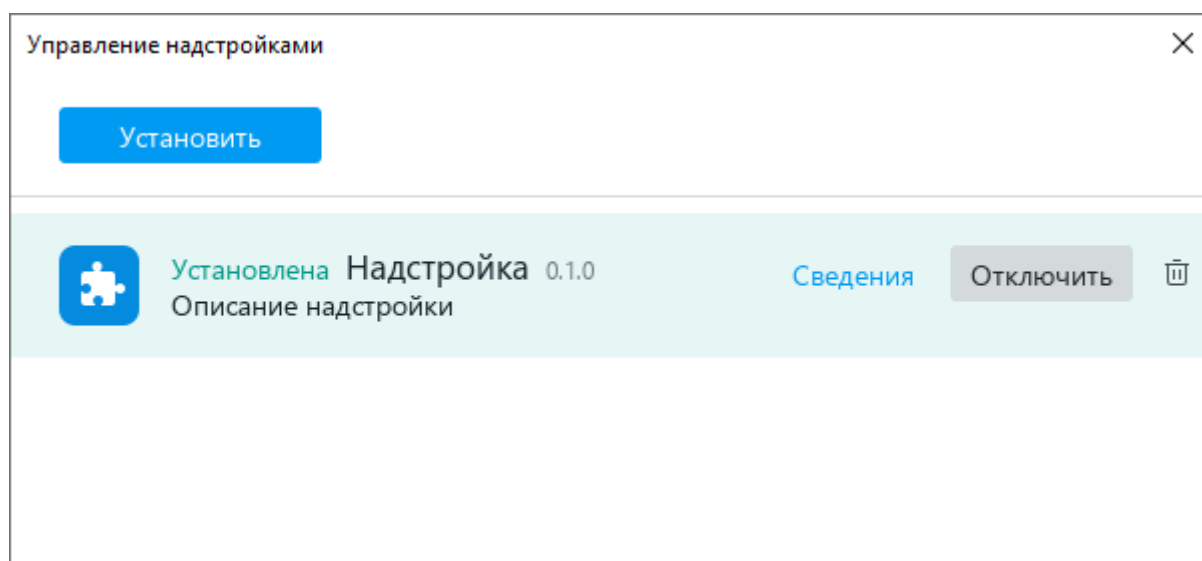
Рисунок 406 – Строка надстройки
