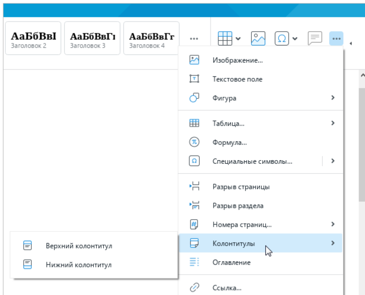
Рисунок 289 – Панель вставки
