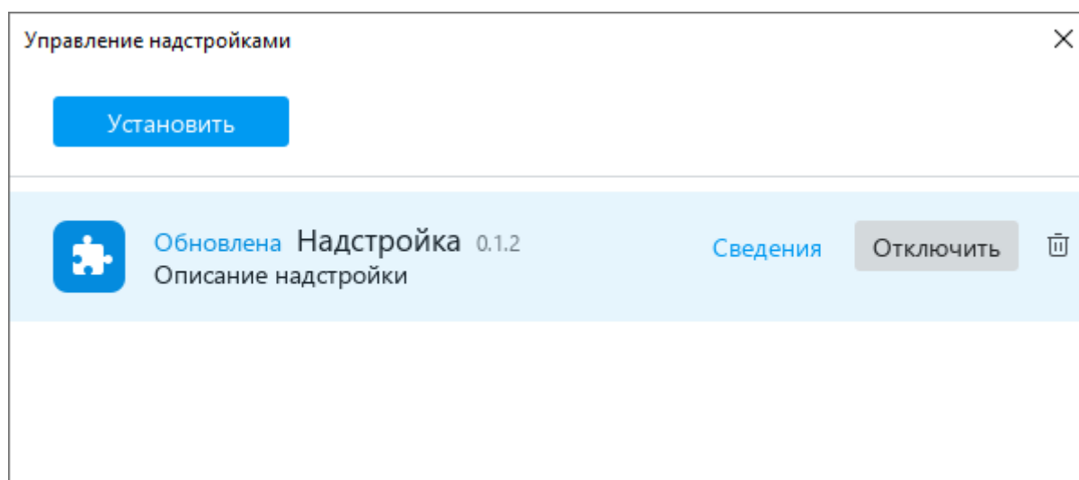
Рисунок 414 – Надстройка обновлена
