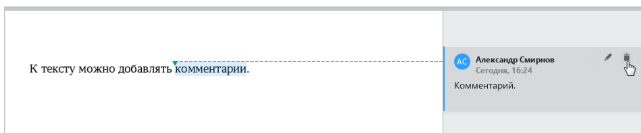
Рисунок 342 – Кнопка Удалить
