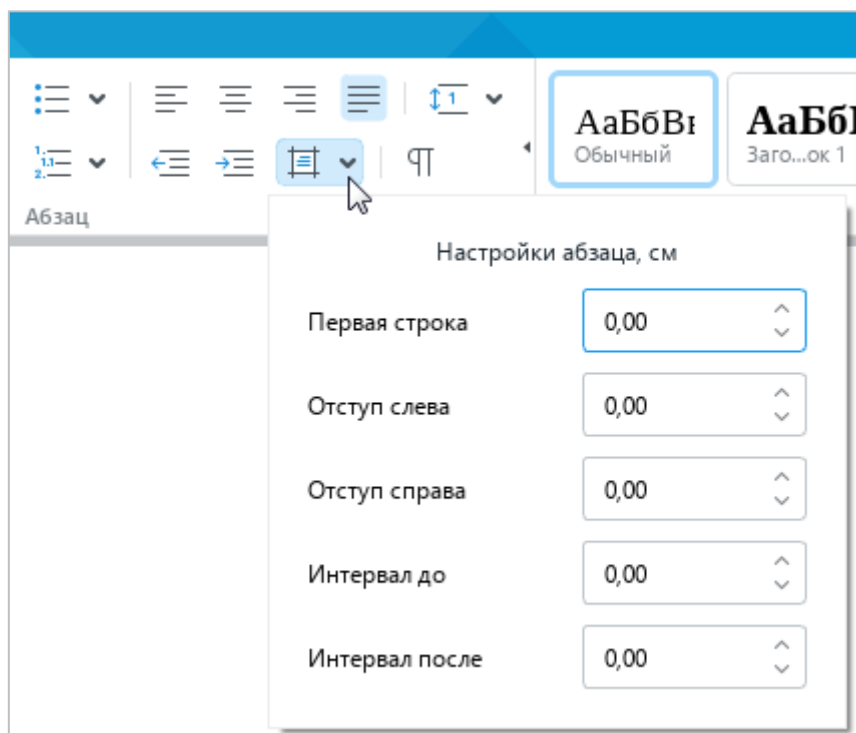
Рисунок 172 – Настройки абзаца
