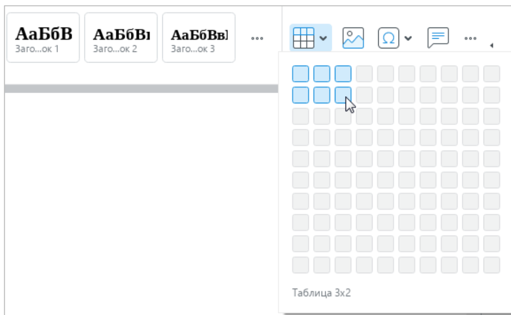
Рисунок 216 – Кнопка Таблица
