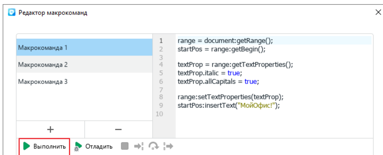
Рисунок 389 – Кнопка Выполнить
