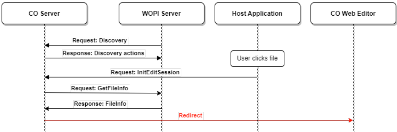
Рисунок 6 - Перенаправление на CO-веб-редактор
