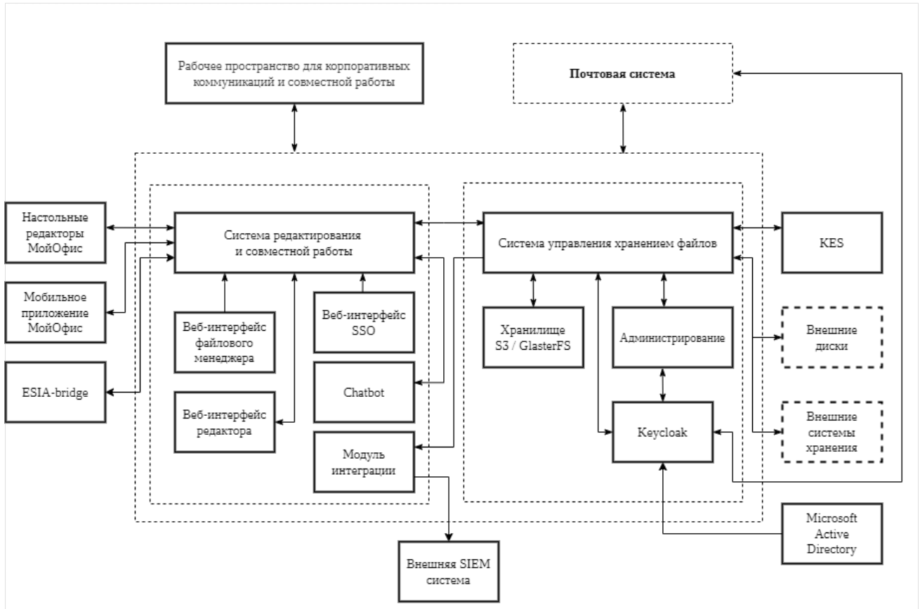
Рисунок 1 — Общая компонентная схема «МойОфис Профессиональный 3»
