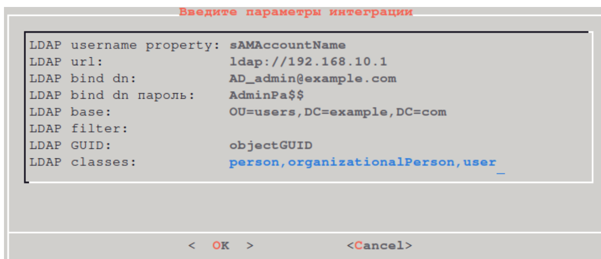
Рисунок 32 — Окно параметров интеграции с AD
