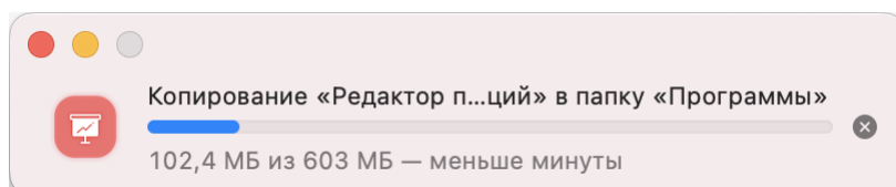
Рисунок 8 – Копирование приложения
