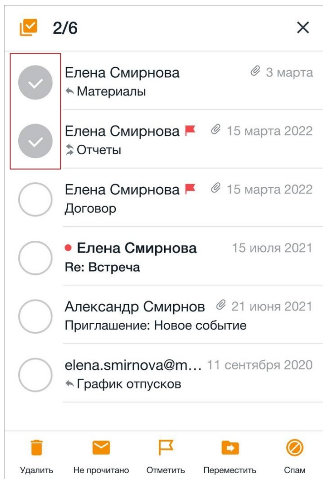
Рисунок 38 — Выбранные письма
