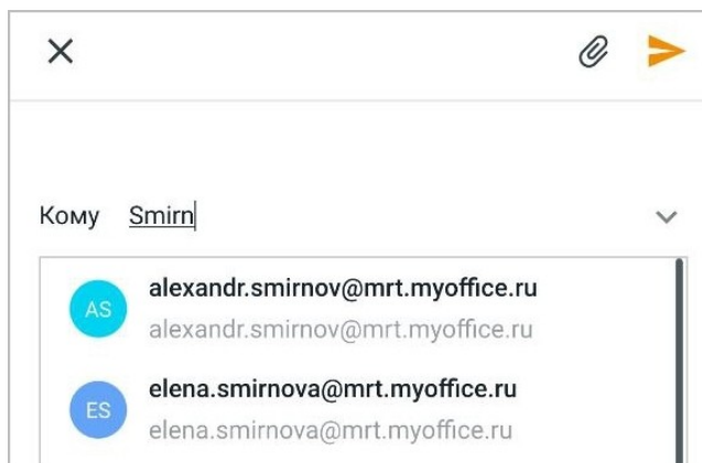
Рисунок 22 — Выбор получателя
