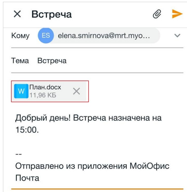
Рисунок 27 — Миниатюра вложения
