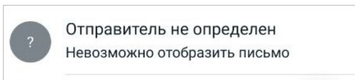
Рисунок 30 — Неподдерживаемое письмо
