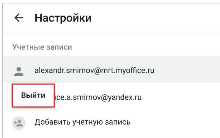
Рисунок 70 — Кнопка Выйти
