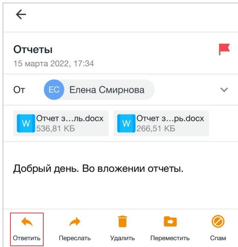
Рисунок 36 — Кнопка Ответить
