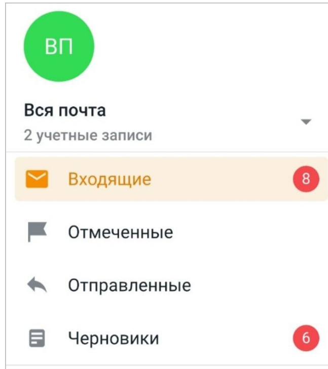
Рисунок 61 — Список смарт-папок
