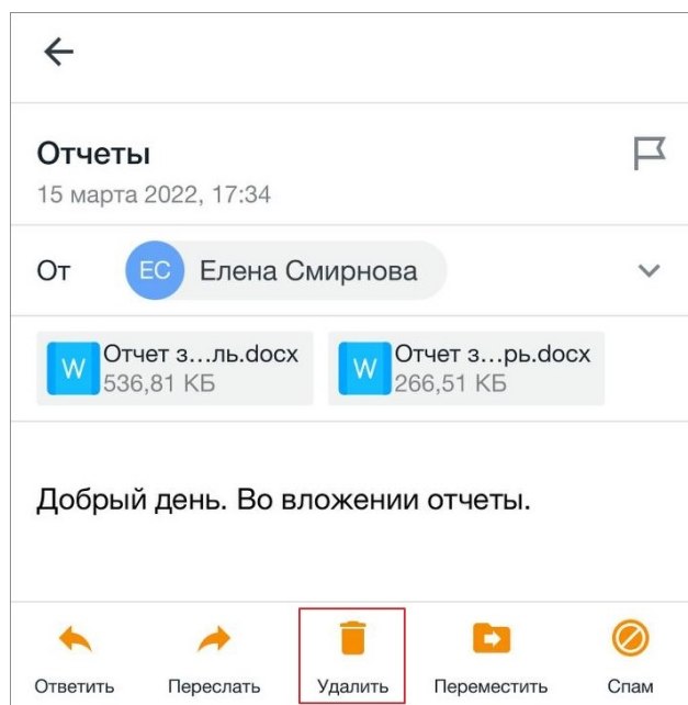
Рисунок 54 — Кнопка Удалить
