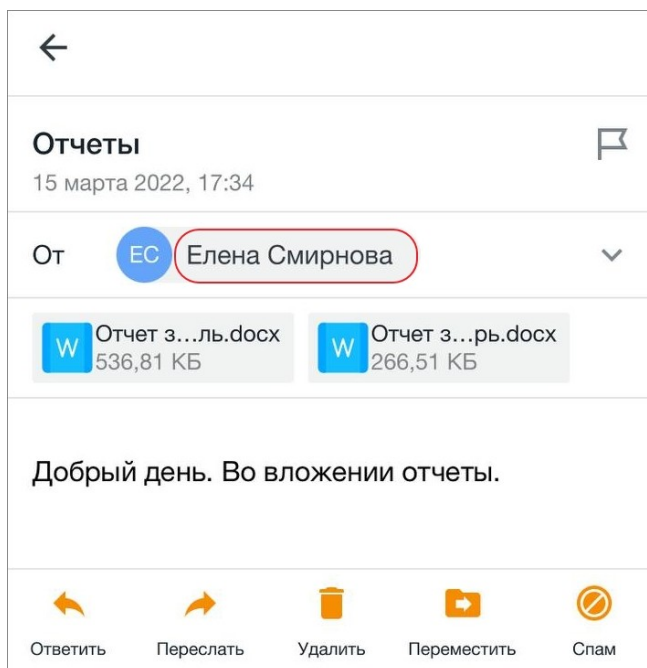
Рисунок 33 — Адрес отправителя
