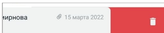
Рисунок 53 — Индикатор Удалить
