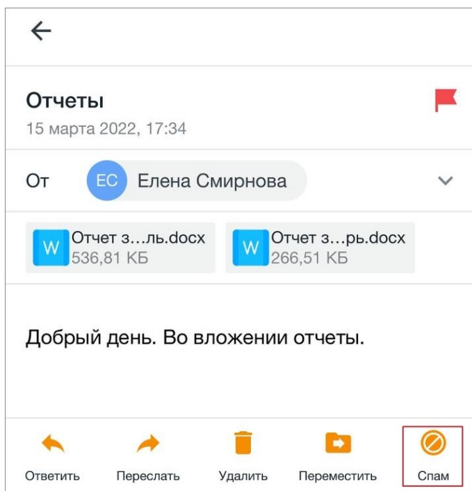
Рисунок 51 — Кнопка Спам
