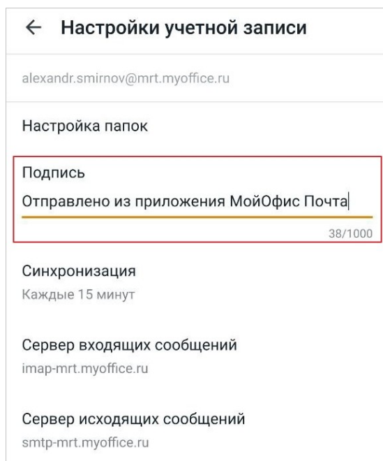
Рисунок 69 — Добавление подписи
