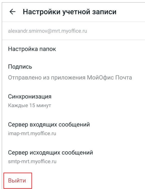
Рисунок 71 — Кнопка Выйти
