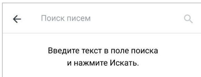
Рисунок 56 — Поисковая строка
