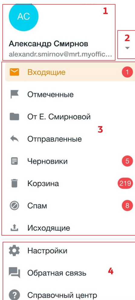
Рисунок 19 — Панель навигации
