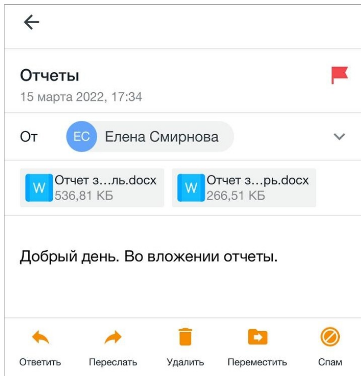
Рисунок 29 — Просмотр письма
