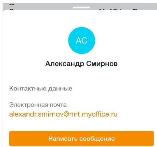
Рисунок 34 — Карточка контакта
