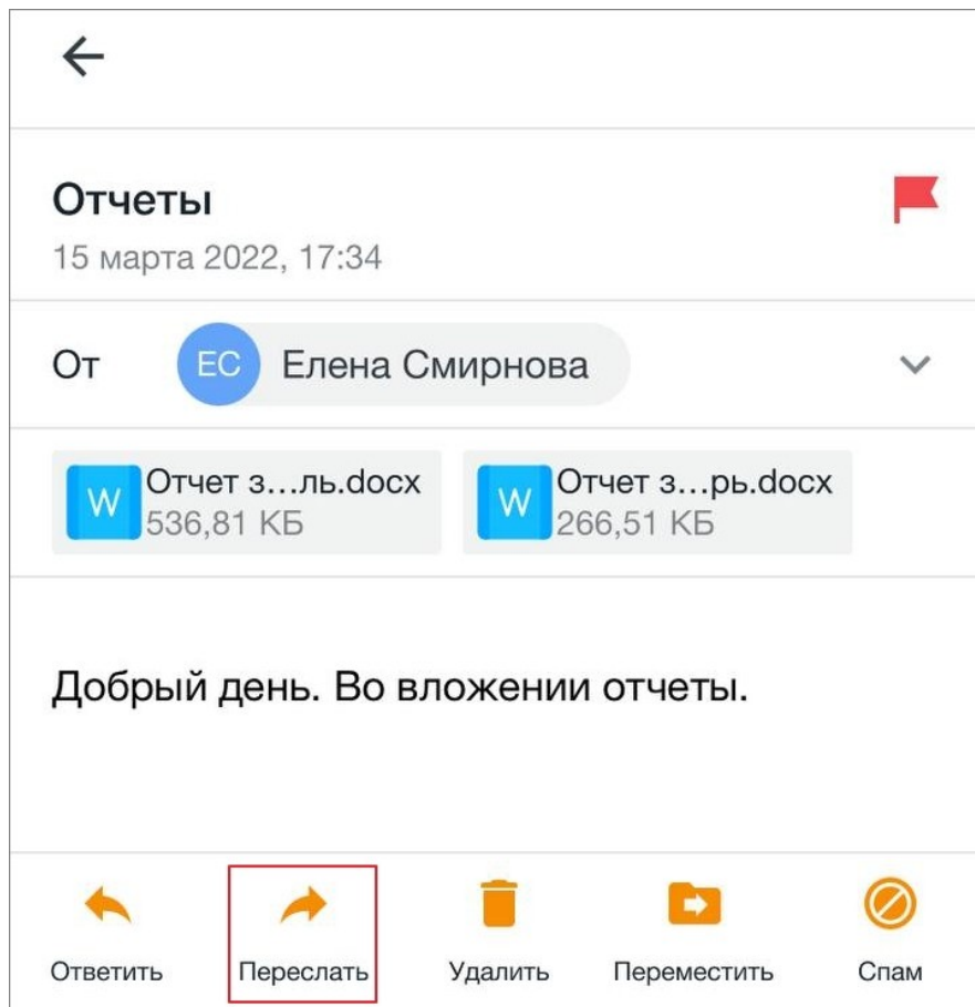
Рисунок 37 — Кнопка Переслать
