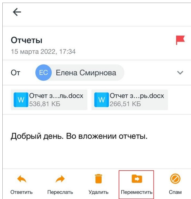
Рисунок 40 — Кнопка Переместить
