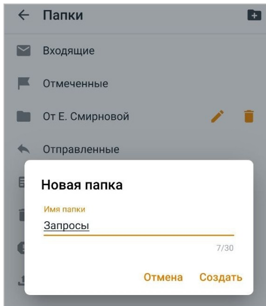
Рисунок 64 — Создание папки
