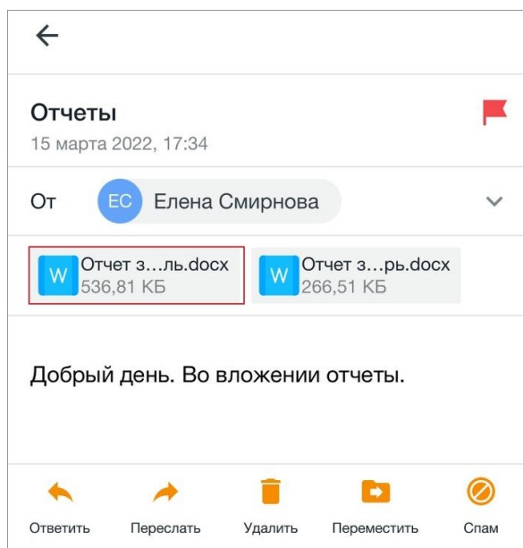
Рисунок 31 — Миниатюра вложения
