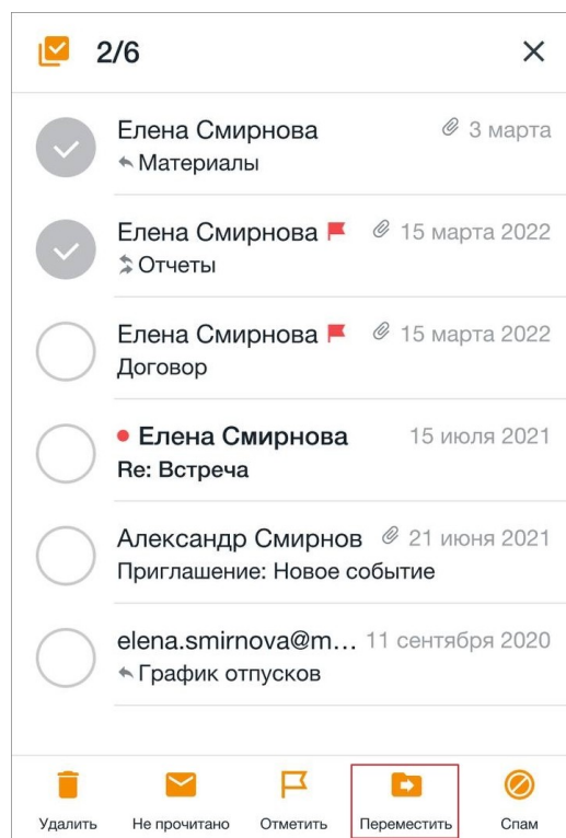
Рисунок 42 — Кнопка Переместить
