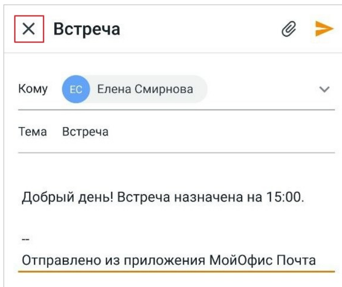
Рисунок 28 — Кнопка Закреть
