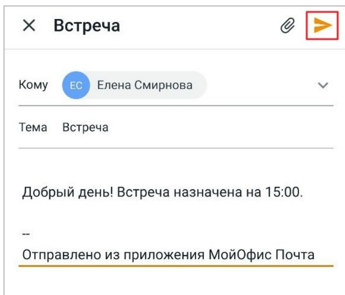
Рисунок 25 — Кнопка Отправить
