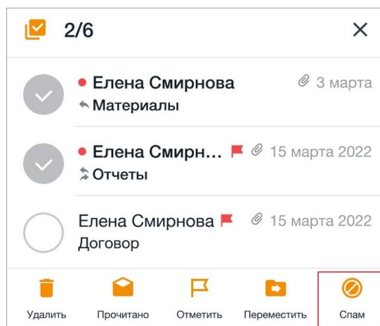
Рисунок 52 — Кнопка Спам
