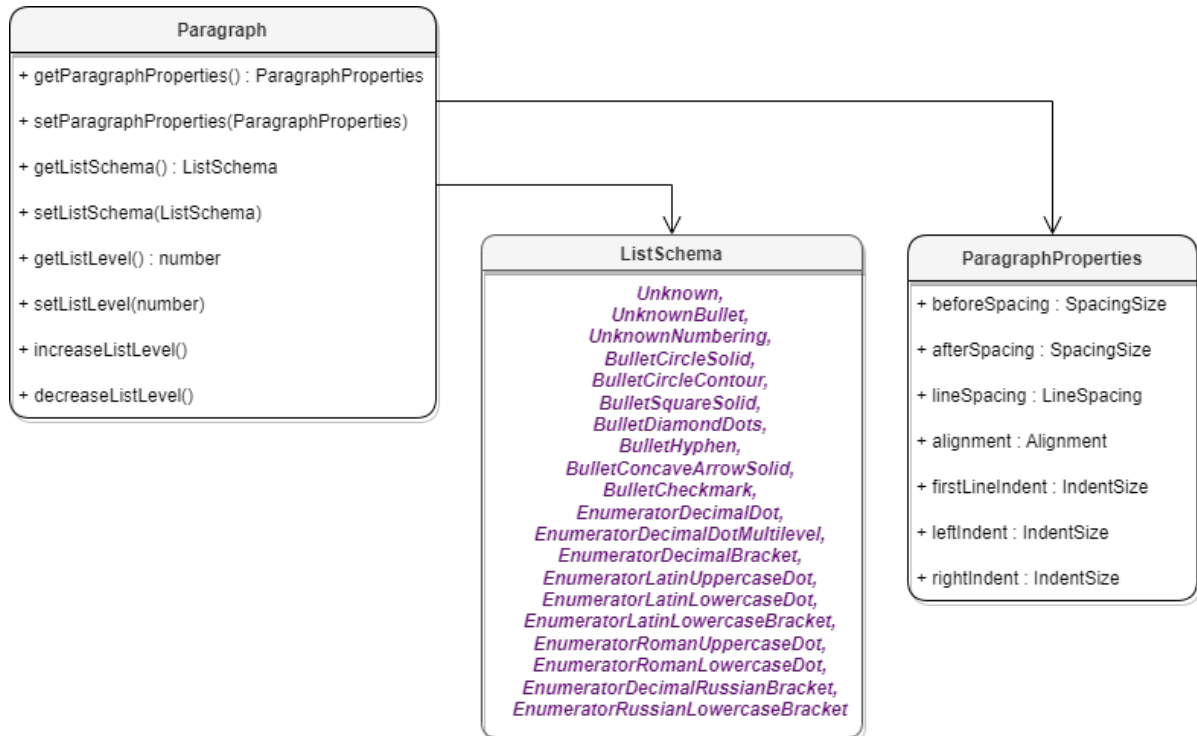
Рисунок 33 – Объектная модель таблиц для работы со свойствами параграфа
