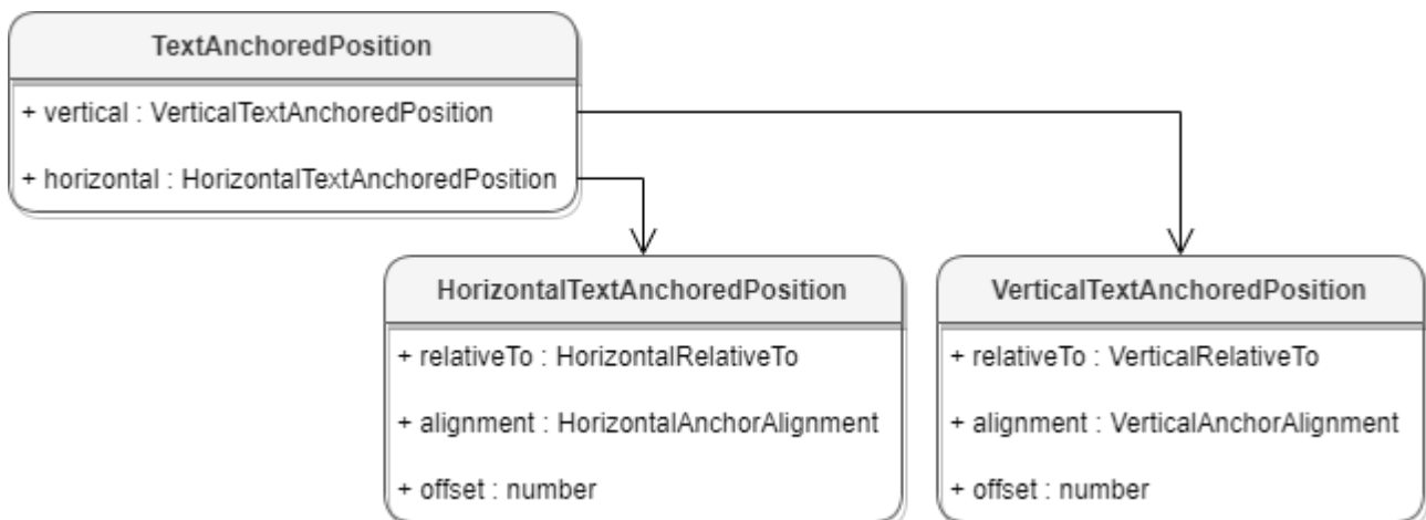
Рисунок 43 – Поля таблицы DocumentAPI.TextAnchoredPosition
