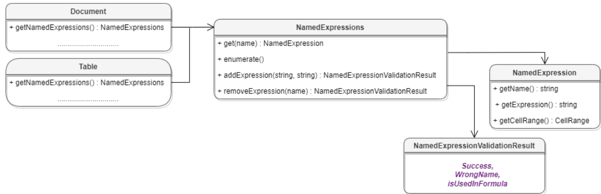
Рисунок 16 – Таблицы для работы с именованными диапазонами
