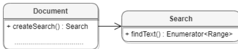
Рисунок 14 – Объектная модель для поиска в документе
