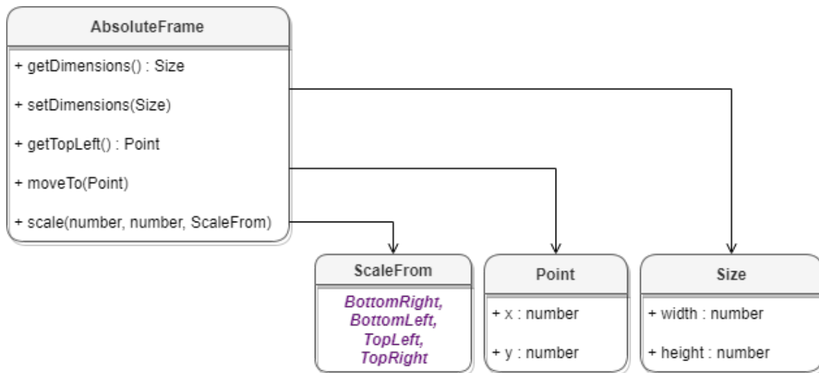
Рисунок 19 – Объектная модель таблицы DocumentAPI.AbsoluteFrame
