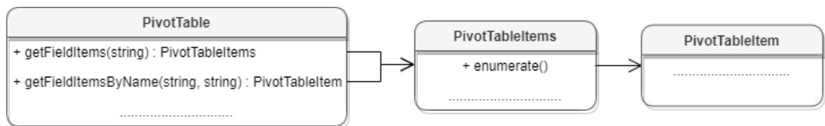
Рисунок 39 – Объектная модель таблиц для работы с элементами сводных таблиц
