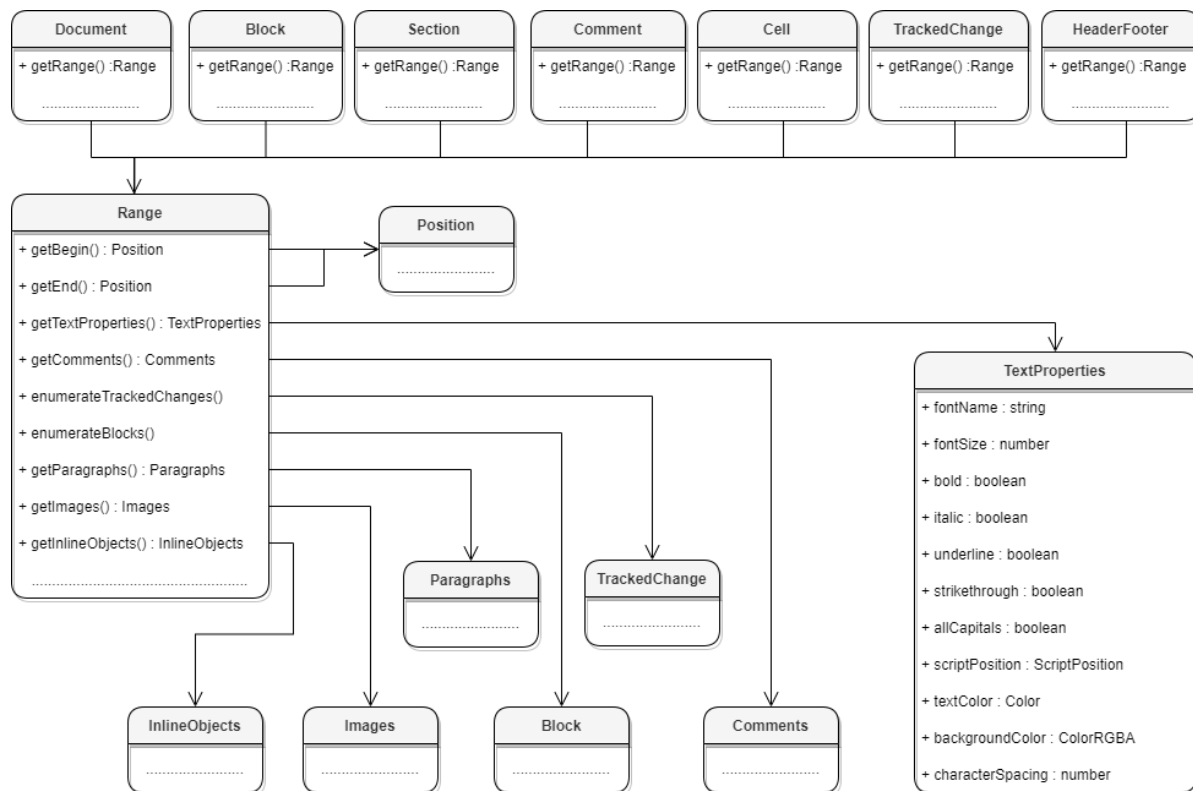
Рисунок 40 – Объектная модель для работы с таблицей DocumentAPI . Range
