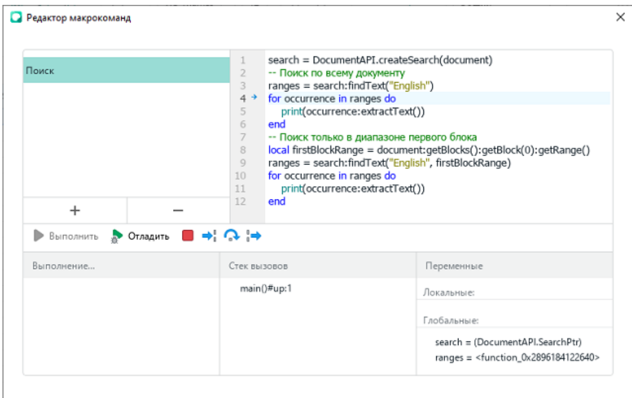
Рисунок 2 – Окно редактора макрокоманд в начале отладки
