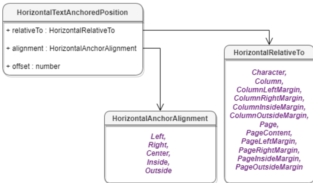
Рисунок 29 – Поля таблицы DocumentAPI.HorizontalTextAnchoredPosition
