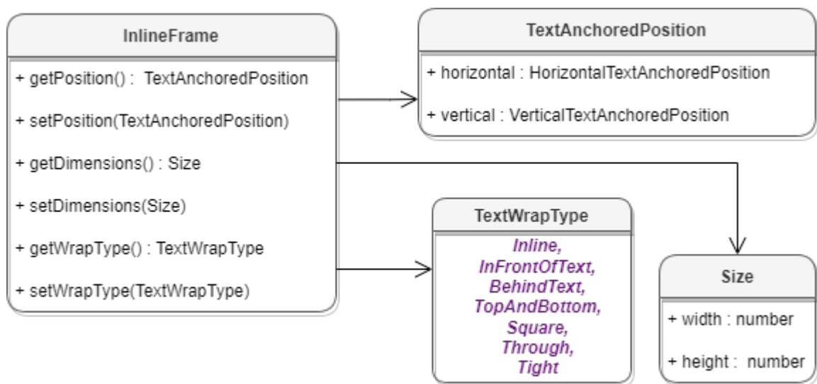
Рисунок 30 – Объектная модель таблицы DocumentAPI.InlineFrame
