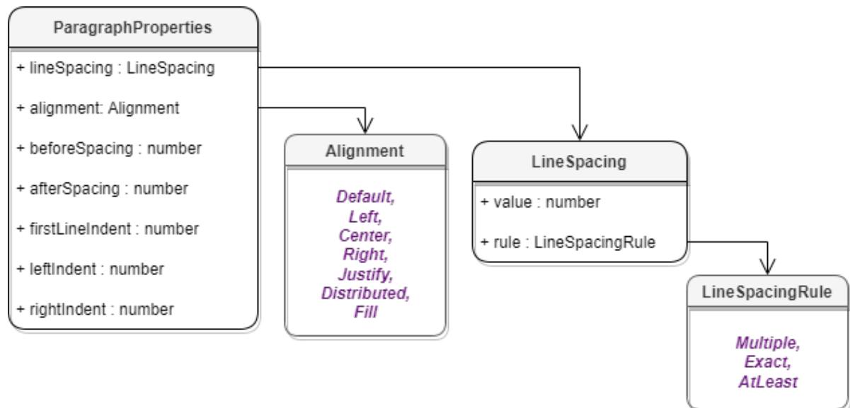
Рисунок 34 – Объектная модель таблиц для работы со свойствами параграфа
