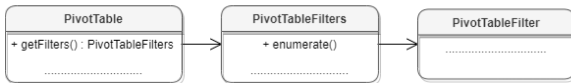
Рисунок 37 – Объектная модель таблиц для работы с фильтрами
