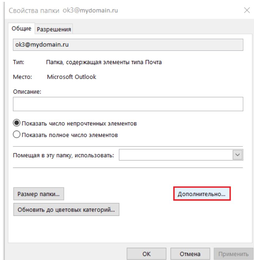
Рисунок 36 – Кнопка Дополнительно
