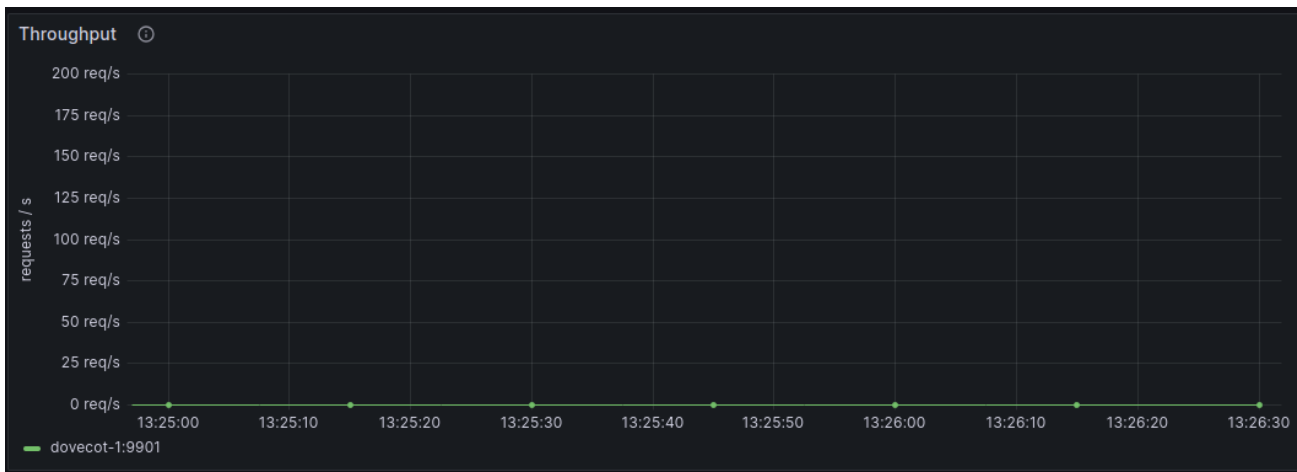
Рисунок 35 – Панель Throughput
