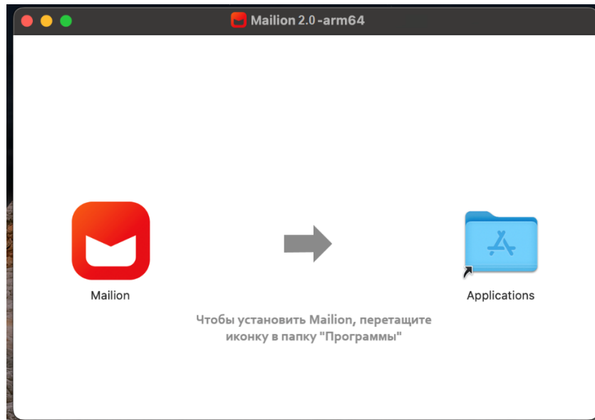
Рисунок 9 — Установка приложения
