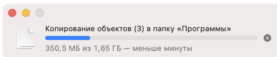
Рисунок 11 – Копирование приложений
