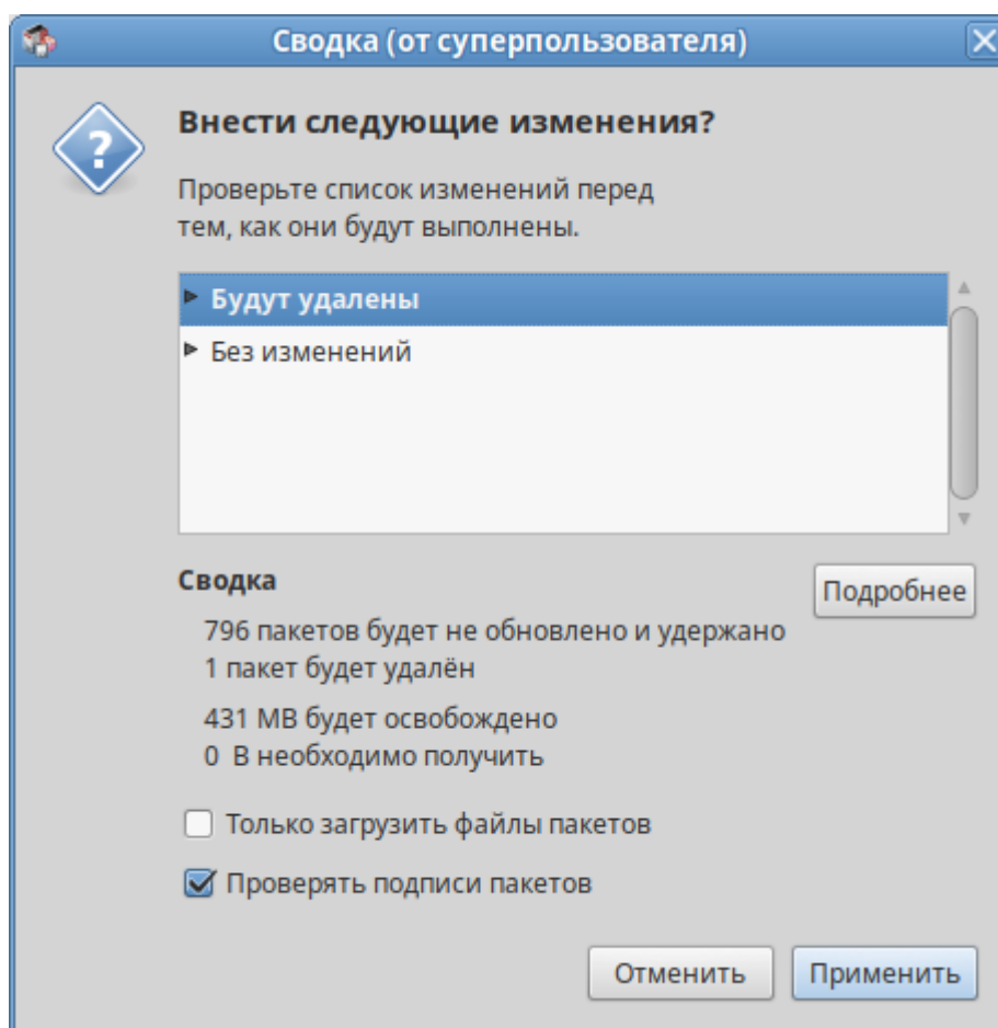
Рисунок 27 – Окно Сводка
