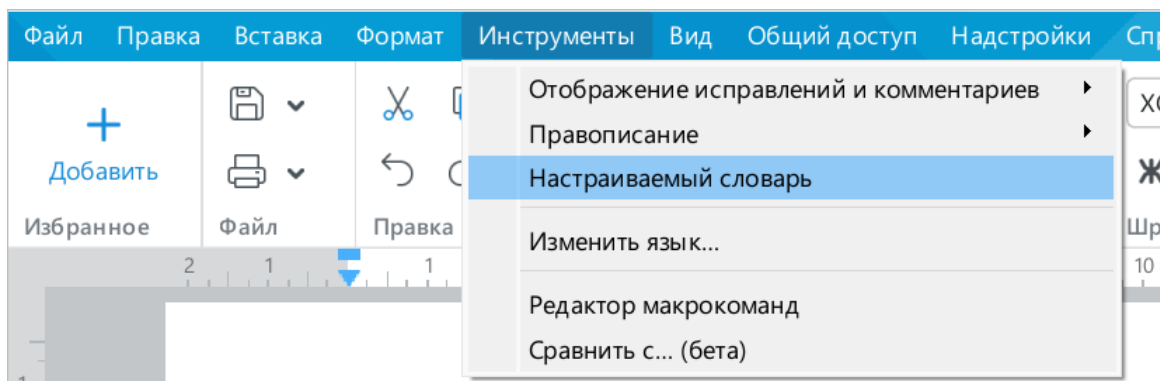
Рисунок 11 – Командное меню
