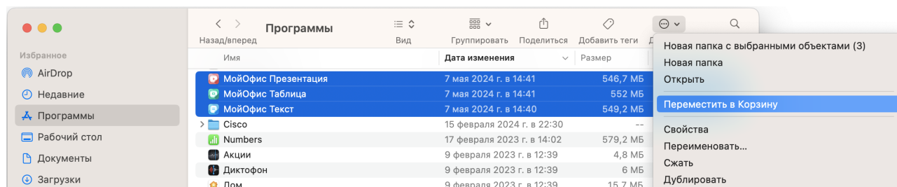
Рисунок 29 – Кнопка Действие
