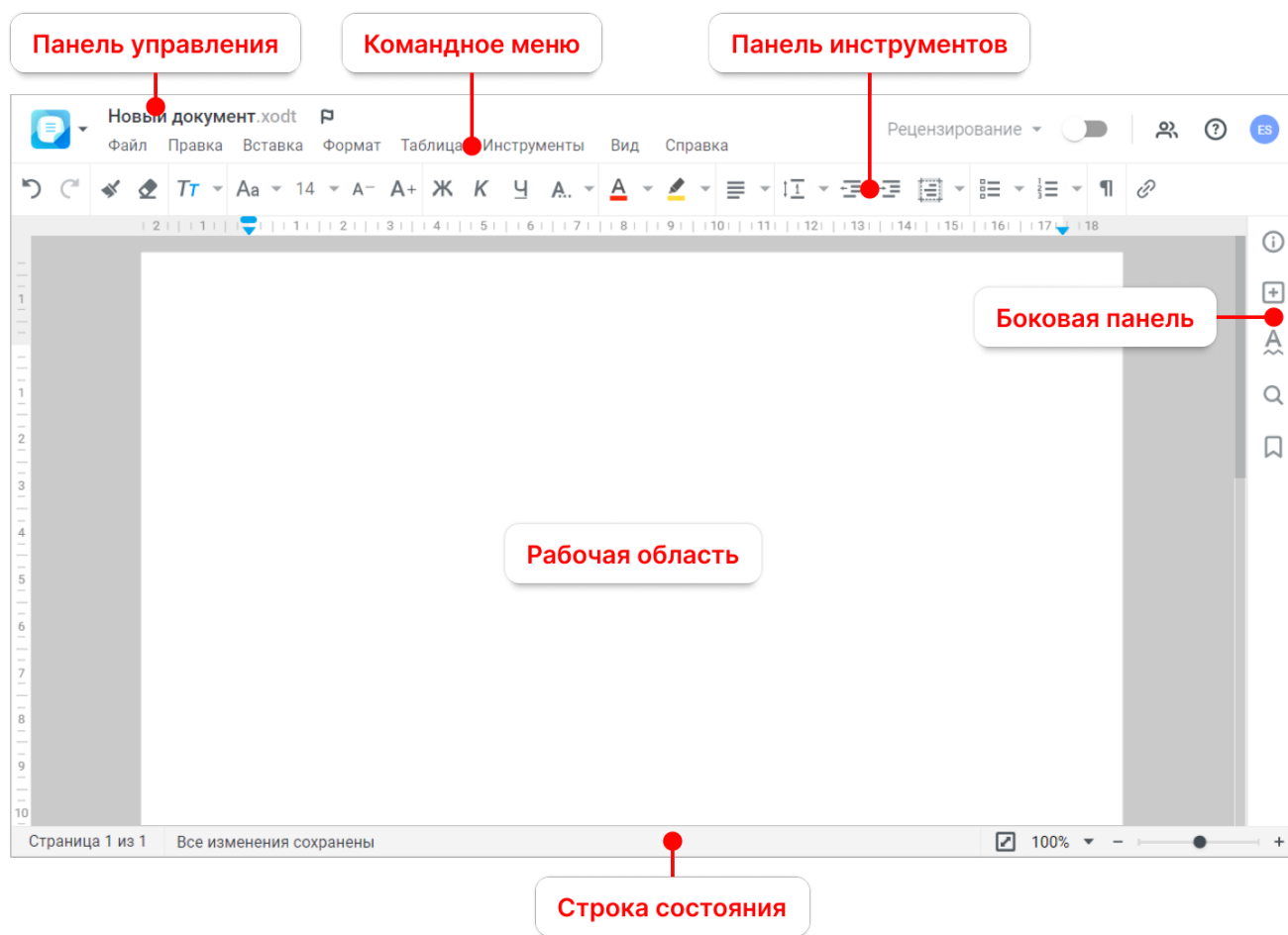
Рисунок 1 – Интерфейс приложения
