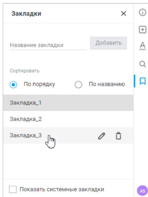
Рисунок 57 – Список закладок
