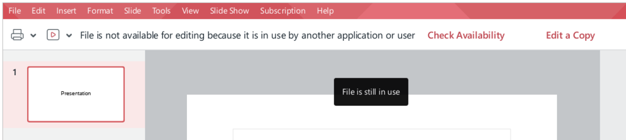
Figure 47. Tooltip message
