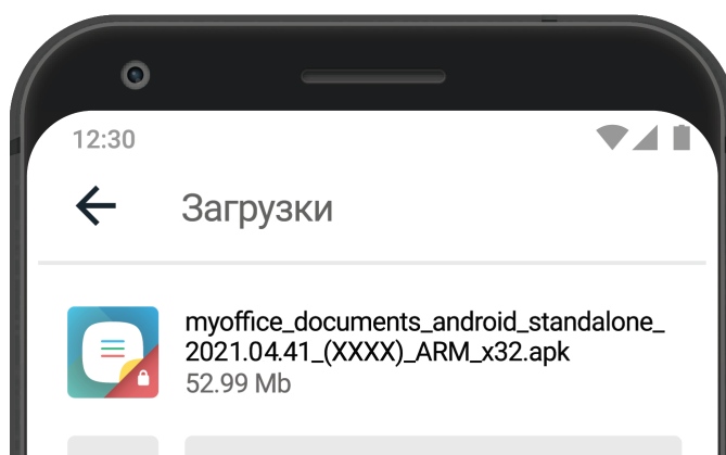
Рисунок 1 — Папка «Загрузки»
