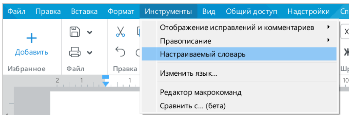
Рисунок 11 – Командное меню
