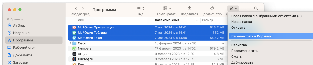
Рисунок 29 – Кнопка Действие
