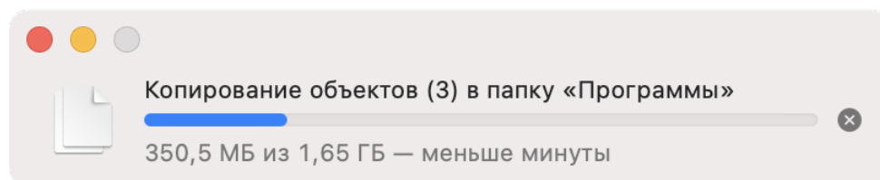
Рисунок 3 – Копирование приложений
