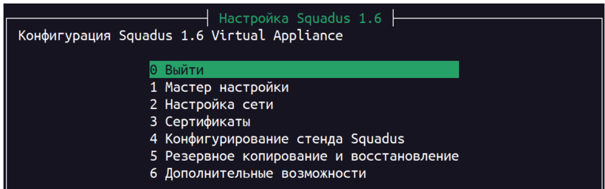
Рисунок 8 — Основное меню утилиты va-squadus
