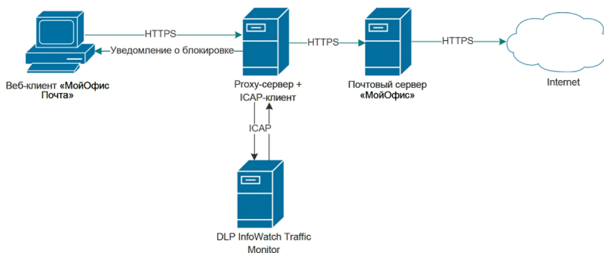
Рисунок 32 - Установка DLP Infowatch traffic monitor “в разрыв” (режим блокировки)
