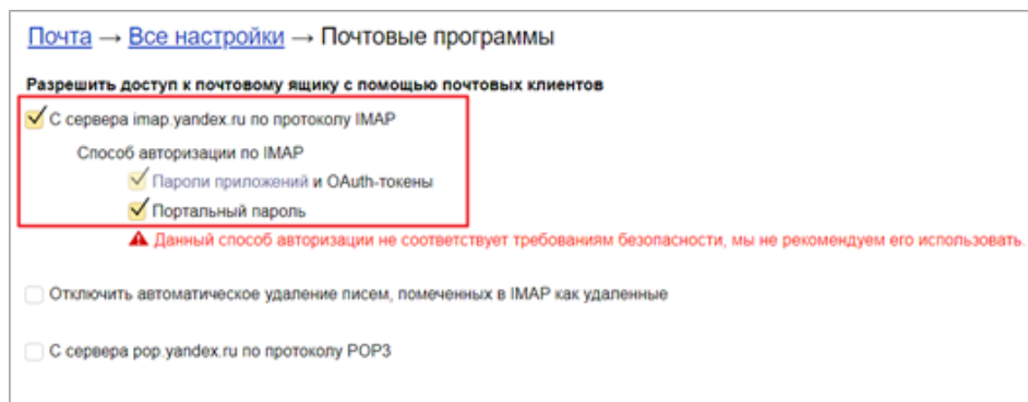
Рисунок 14 — Настройки в почтовом клиенте «Яндекс»
