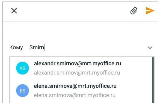
Рисунок 23 — Выбор получателя
