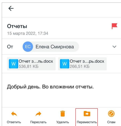
Рисунок 41 — Кнопка Переместить
