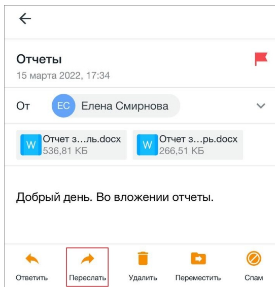
Рисунок 38 — Кнопка Переслать
