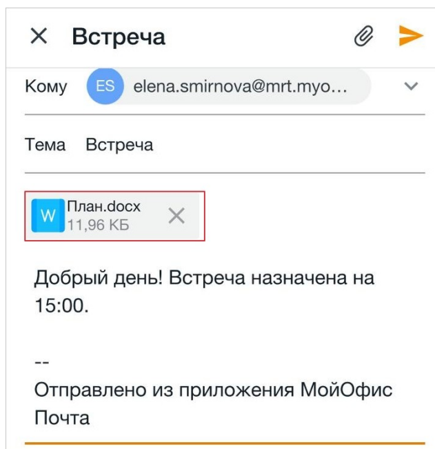
Рисунок 28 — Миниатюра вложения
