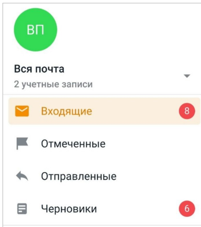
Рисунок 62 — Список смарт-папок
