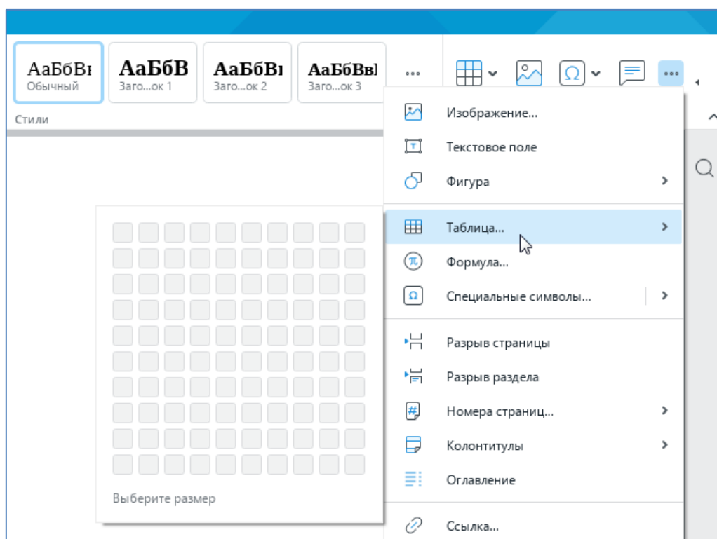
Рисунок 149 – Панель вставки
