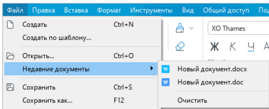
Рисунок 46 – Недавние документы
