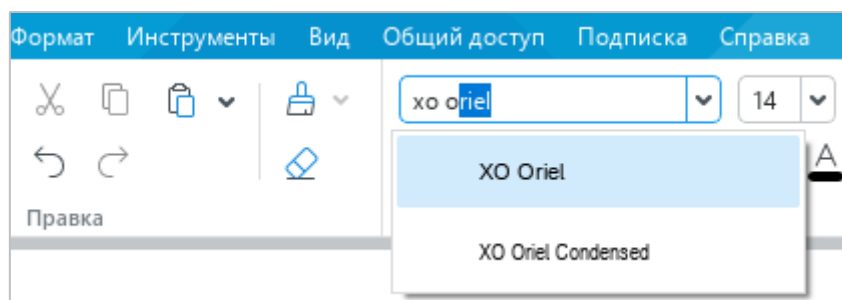
Рисунок 118 – Поиск шрифта
