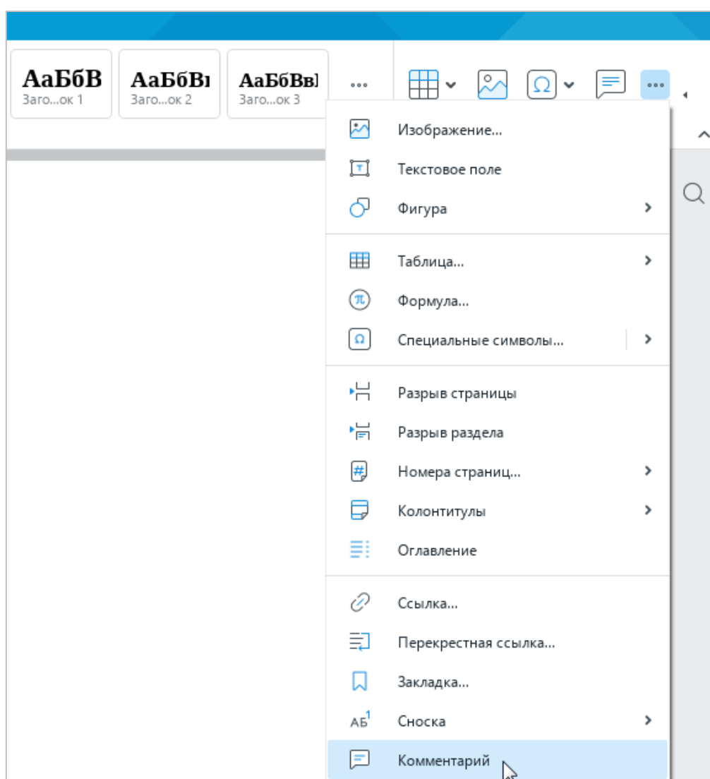
Рисунок 295 – Панель вставки
