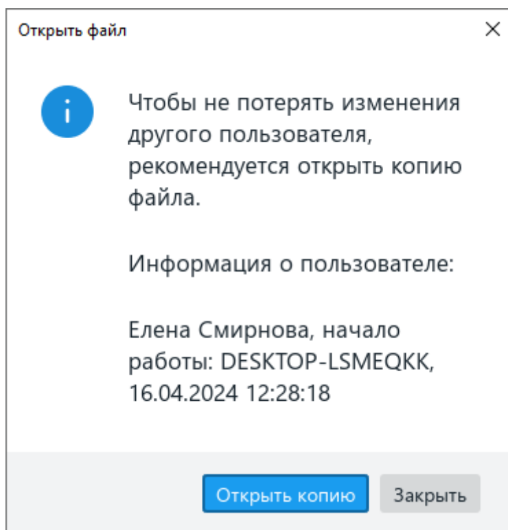
Рисунок 45 – Диалоговое окно
