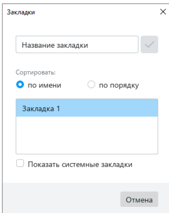
Рисунок 84 – Закладка добавлена
