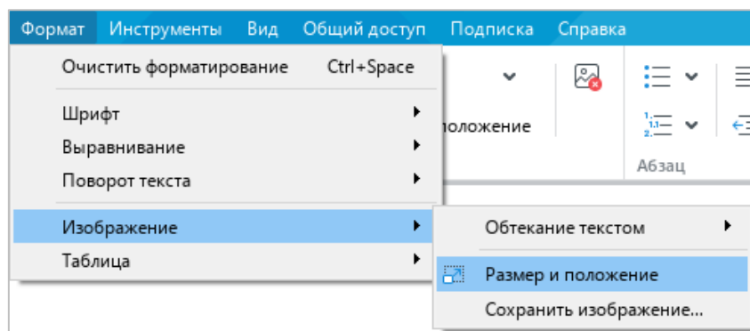
Рисунок 195 – Подменю Изображение
