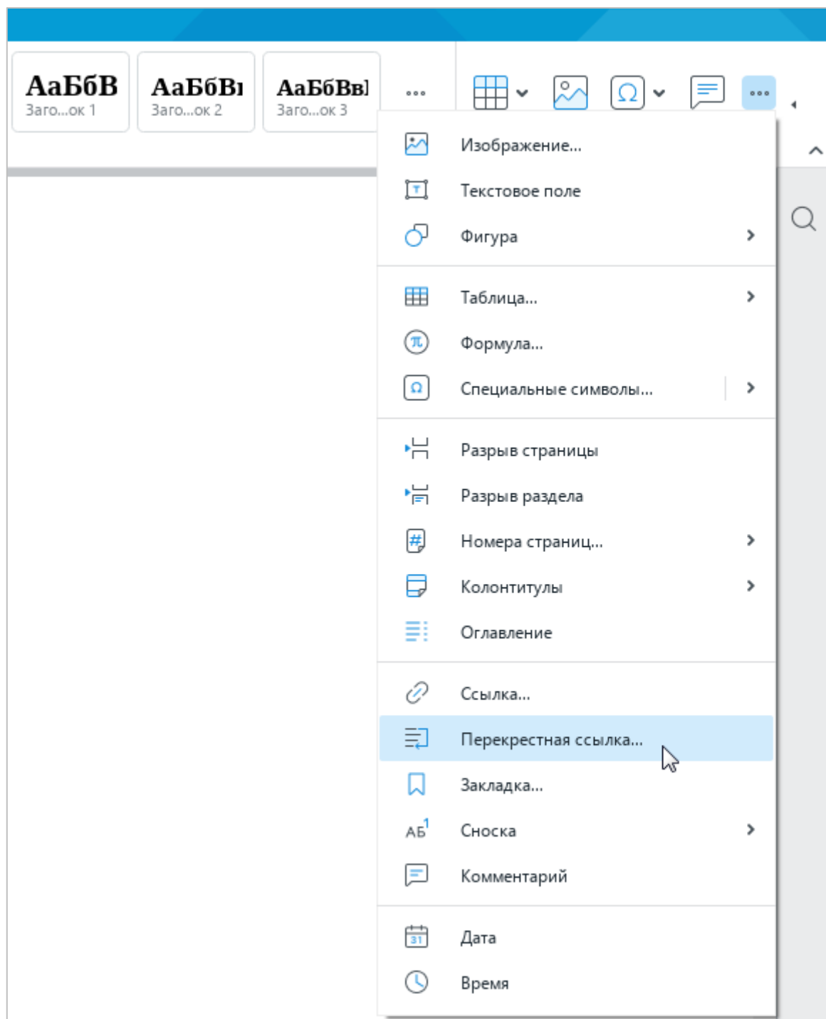
Рисунок 79 – Панель вставки
