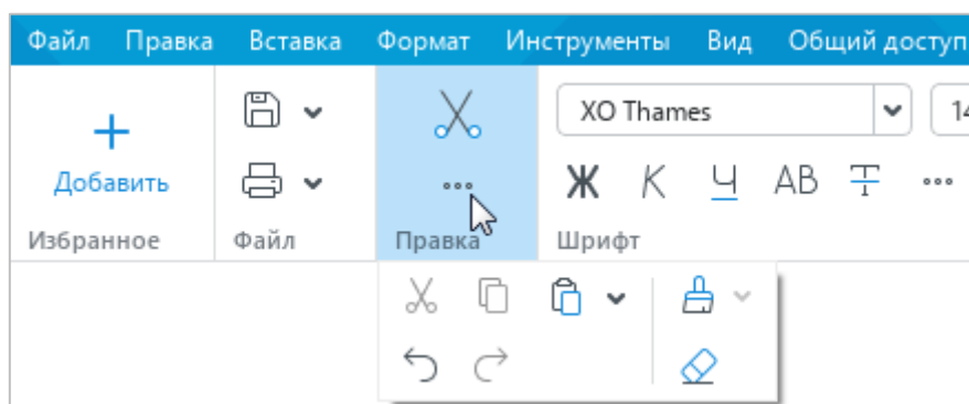
Рисунок 22 – Инструменты раздела
