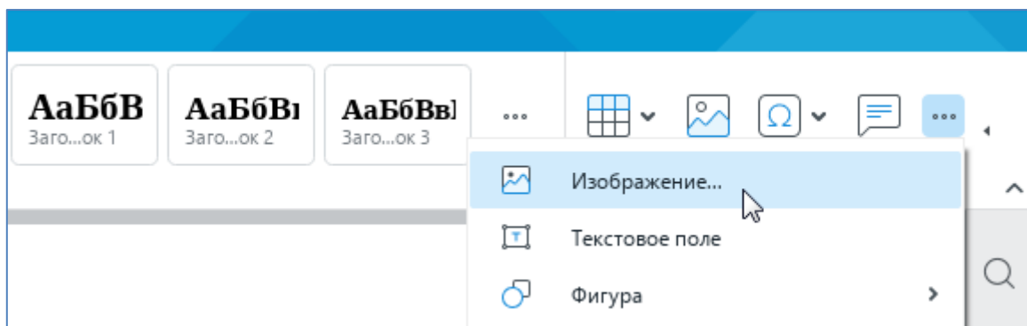
Рисунок 182 – Панель вставки
