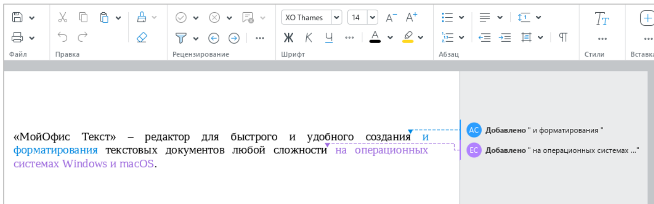
Рисунок 282 – Исправления
