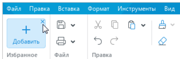
Рисунок 31 – Раздел Избранное
