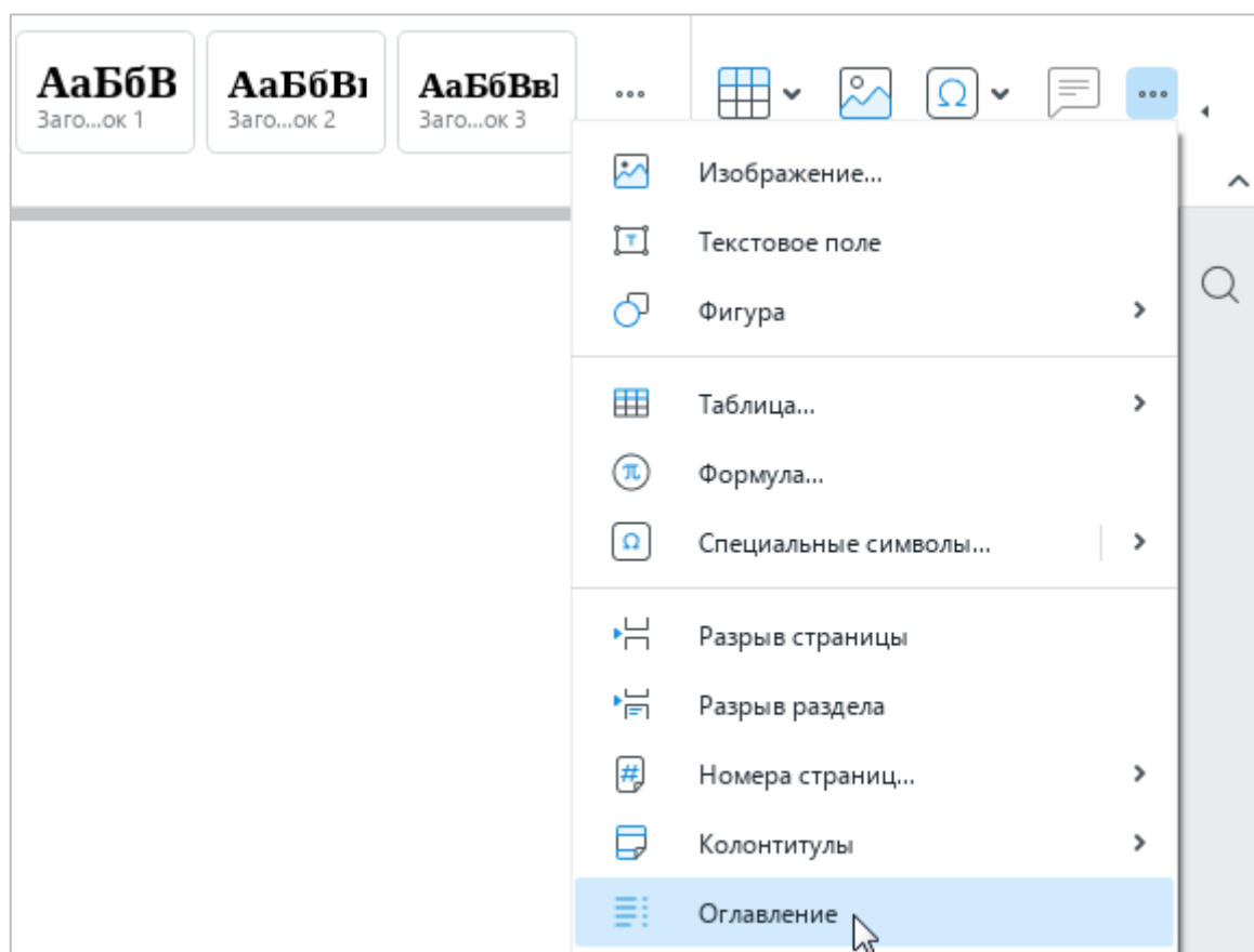
Рисунок 264 – Панель вставки
