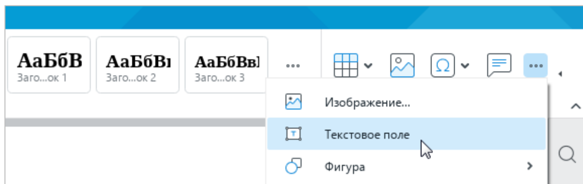
Рисунок 203 – Панель вставки
