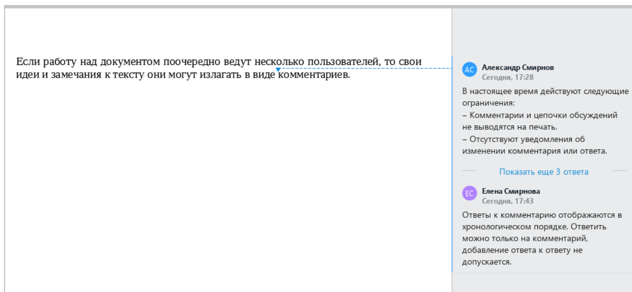
Рисунок 299 – Цепочка
