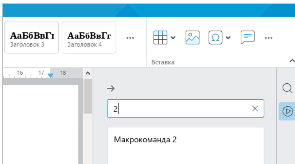
Рисунок 320 – Поиск макрокоманды
