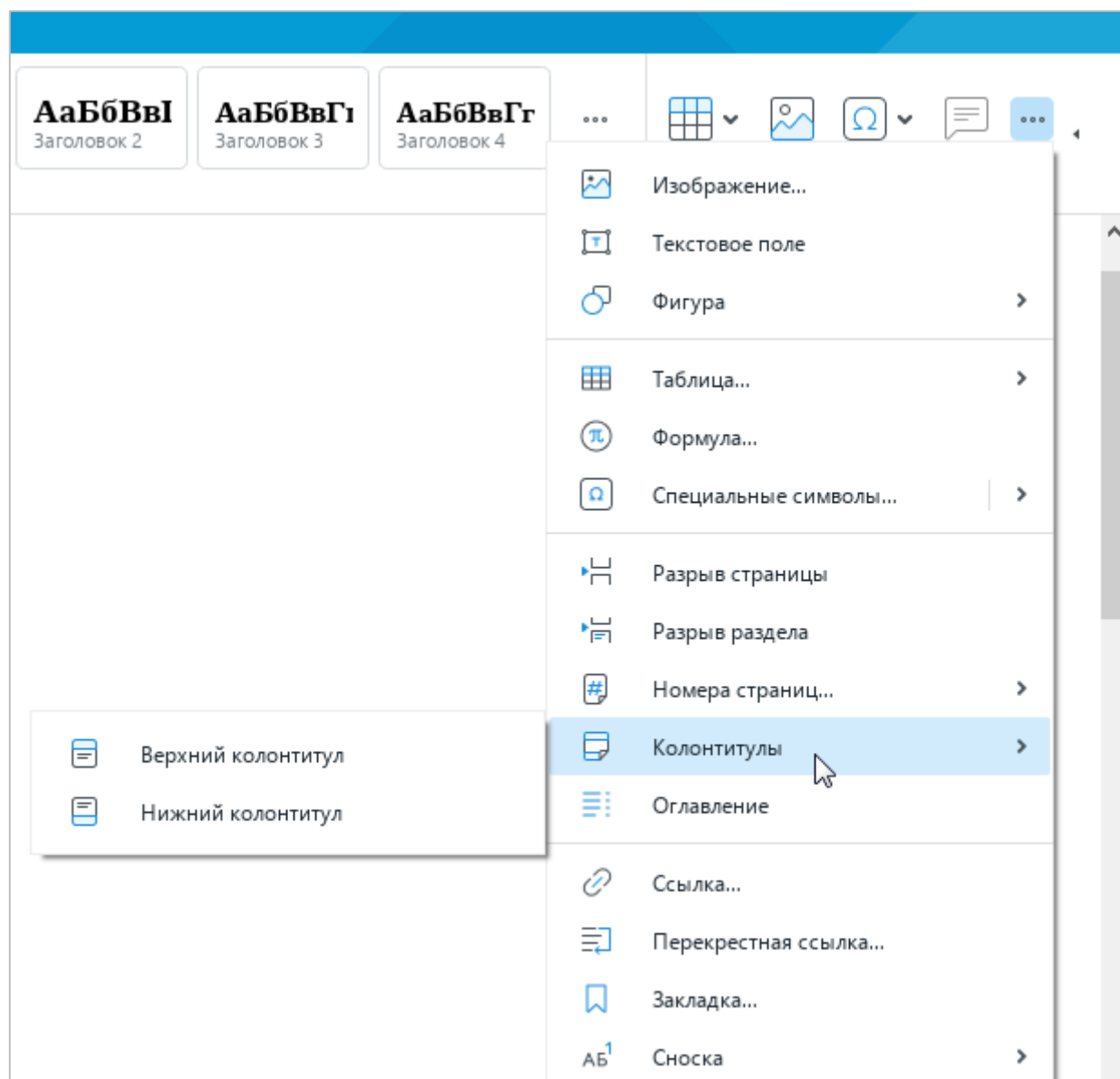
Рисунок 247 – Панель вставки
