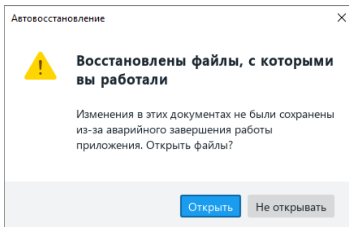
Рисунок 59 – Диалоговое окно
