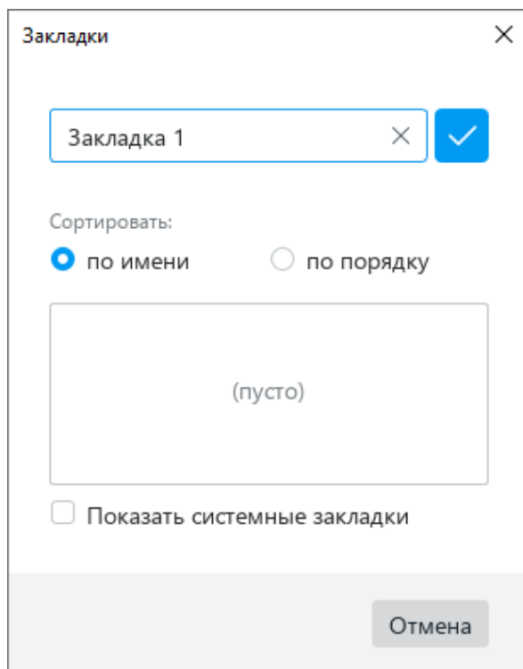
Рисунок 83 – Окно Закладки
