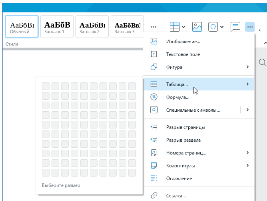
Рисунок 177 – Панель вставки
