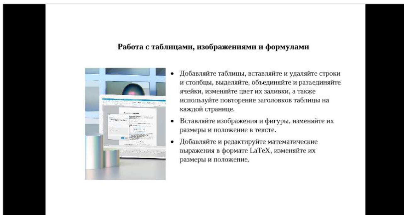
Рисунок 280 – Режим презентации
