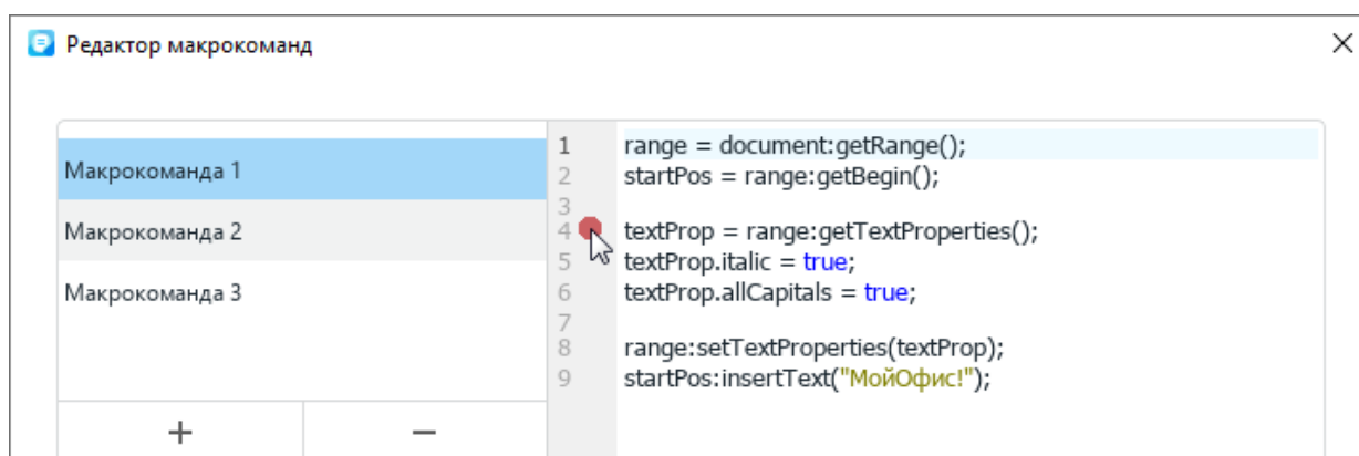
Рисунок 327 – Точка останова
