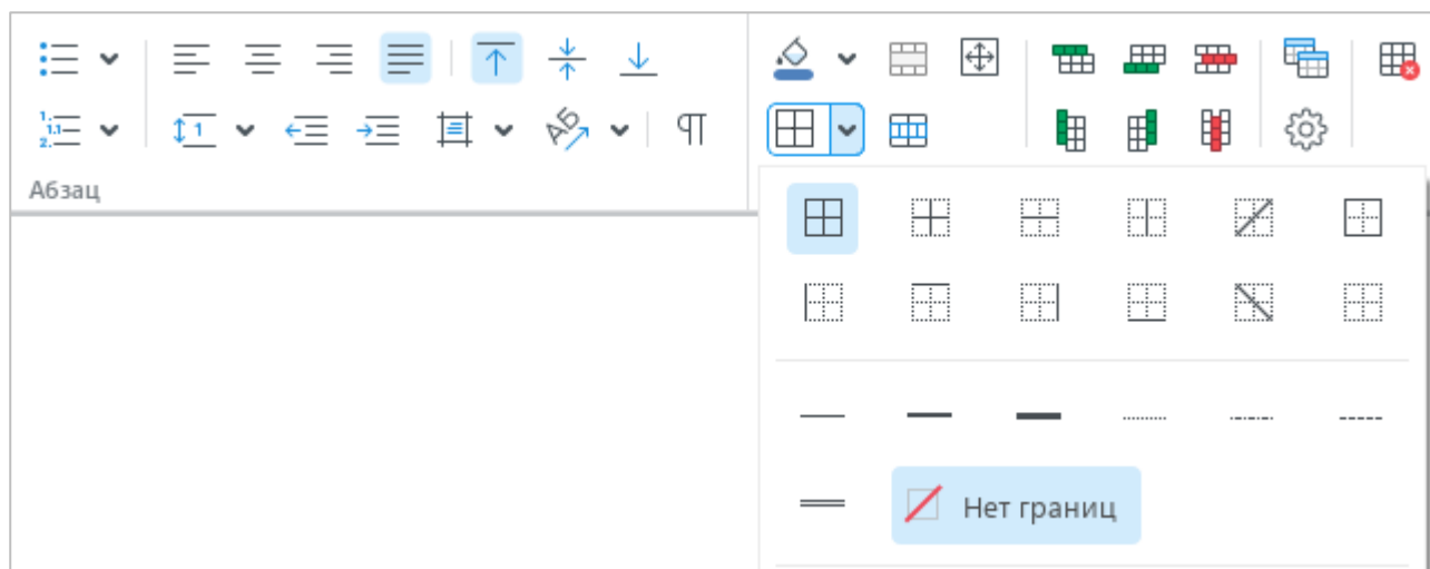
Рисунок 162 – Удаление границ
