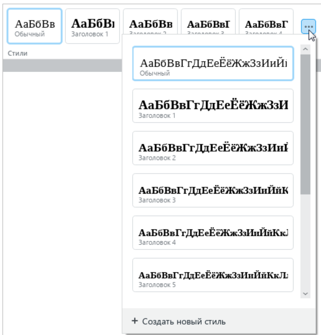
Рисунок 262 – Список стилей
