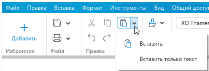
Рисунок 184 – Кнопка Вставить
