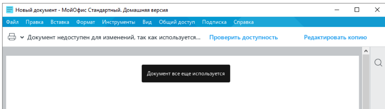
Рисунок 44 – Всплывающее сообщение
