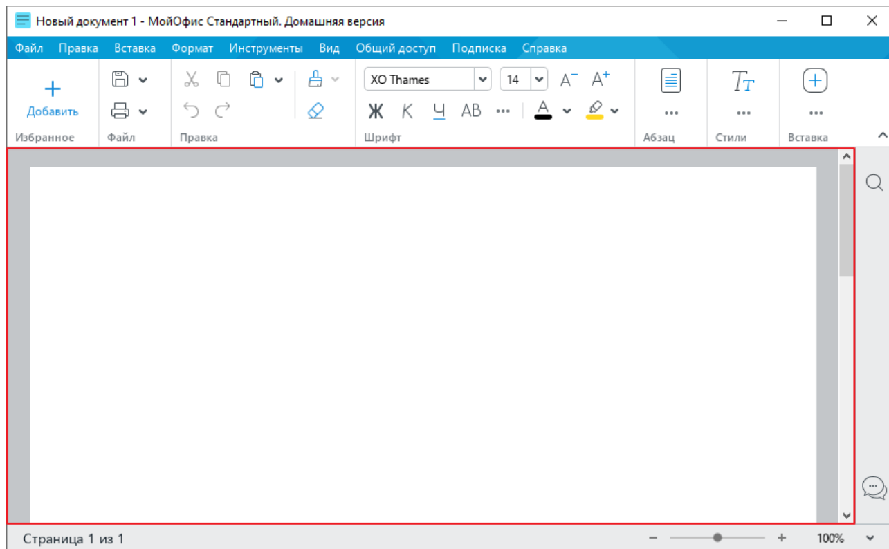
Рисунок 32 – Рабочая область
