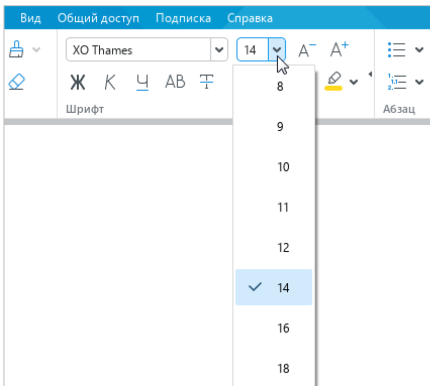
Рисунок 120 – Размер шрифта
