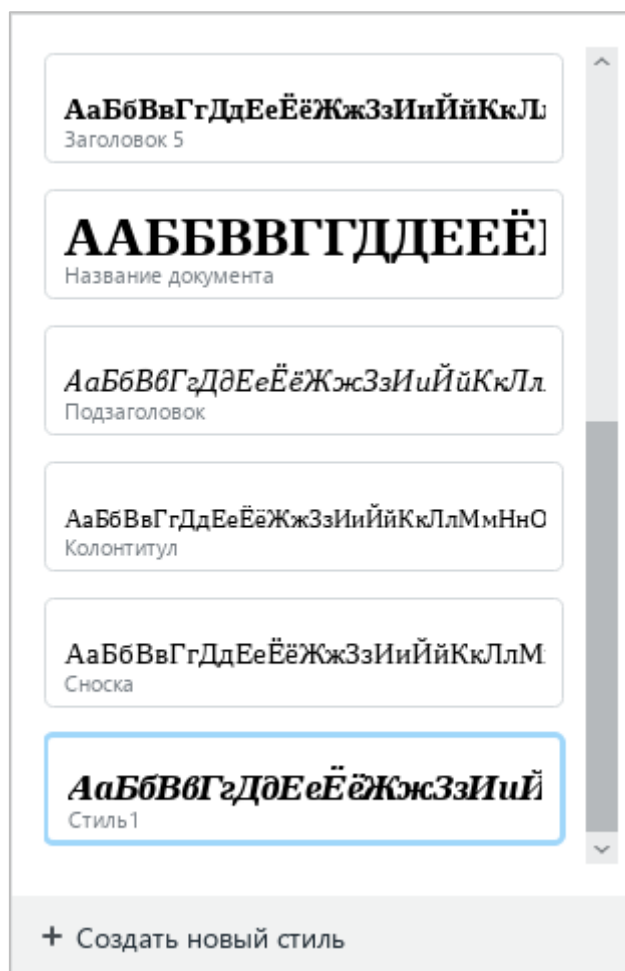
Рисунок 116 – Пользовательский стиль
