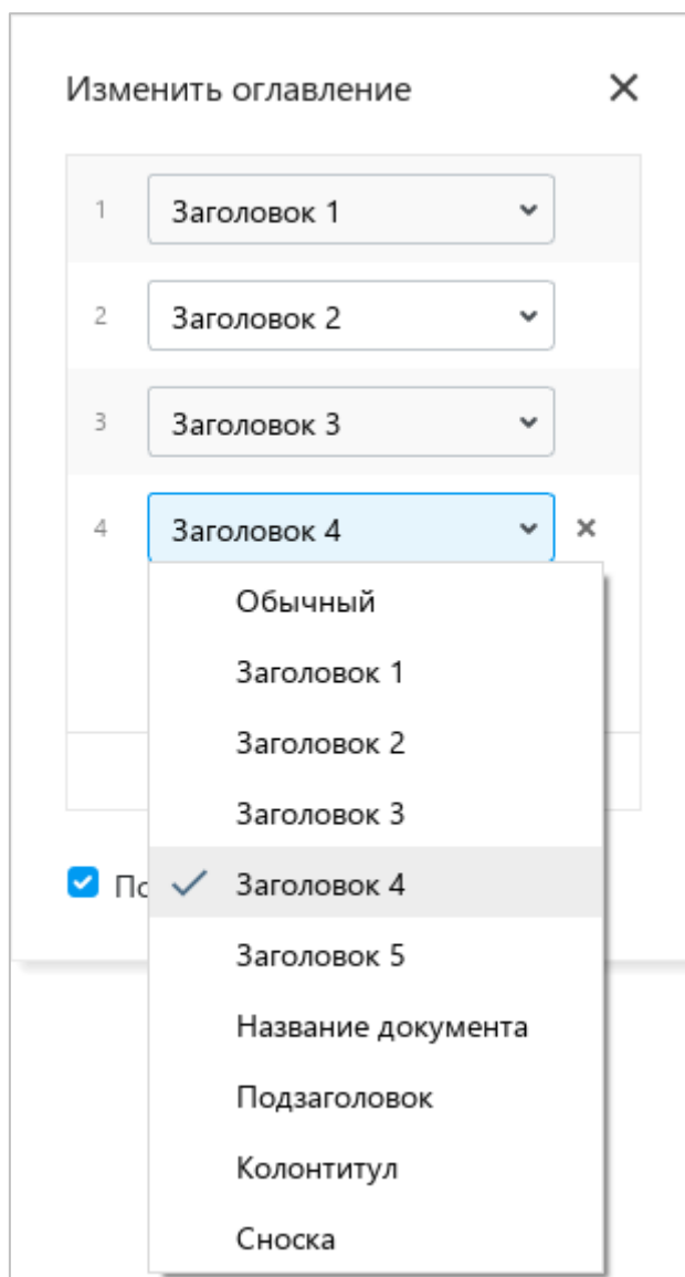
Рисунок 268 – Выбор стиля
