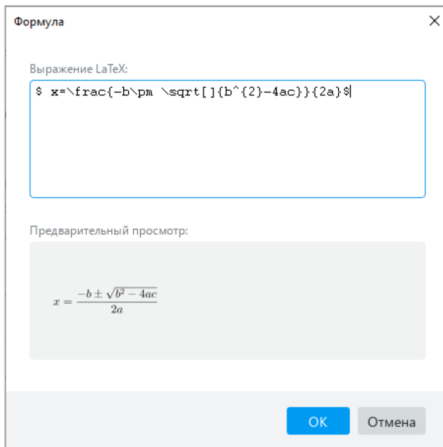
Рисунок 226 – Окно Формула
