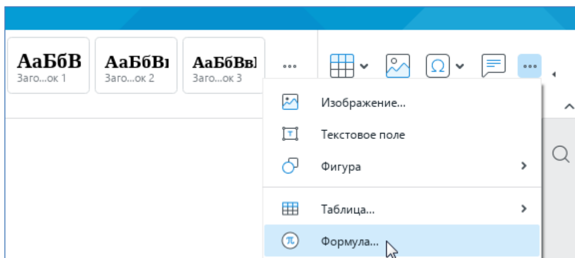
Рисунок 225 – Панель вставки
