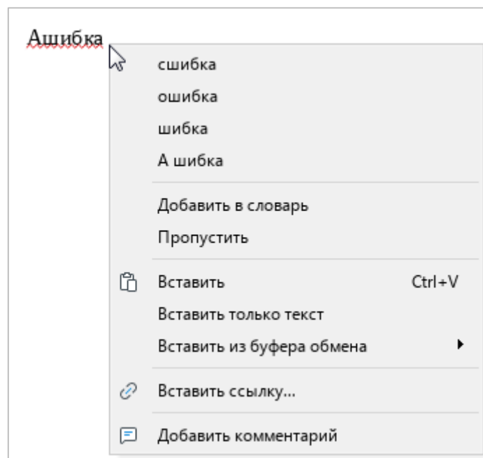
Рисунок 100 – Проверка правописания
