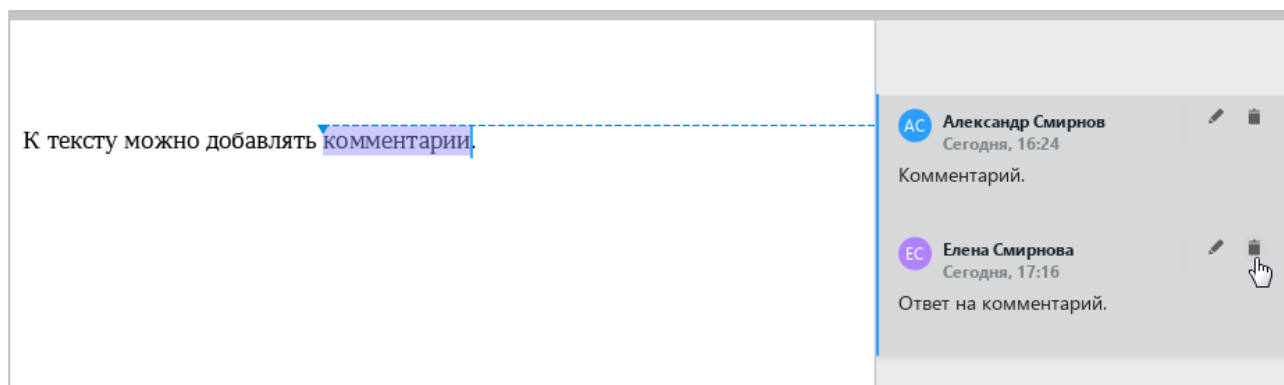
Рисунок 310 – Удаление ответа
