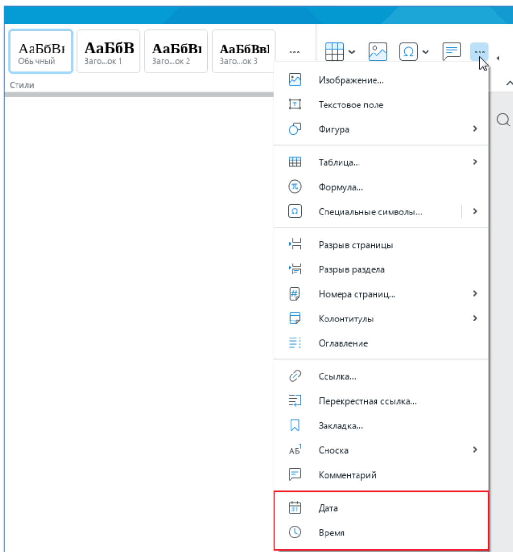
Рисунок 98 – Панель вставки
