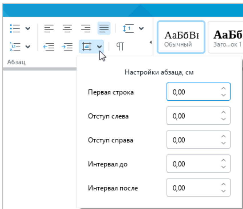
Рисунок 131 – Настройки абзаца
