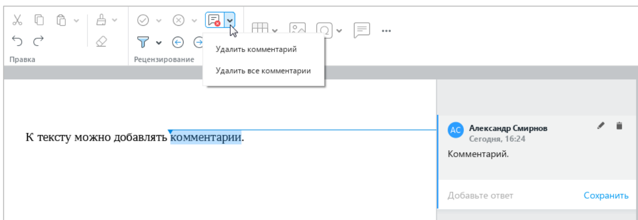
Рисунок 307 – Удаление комментария
