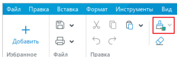
Рисунок 9 – Функция недоступна
