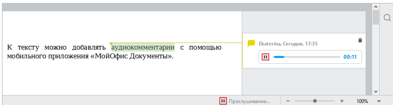
Рисунок 312 – Прослушивание аудиокomentarия
