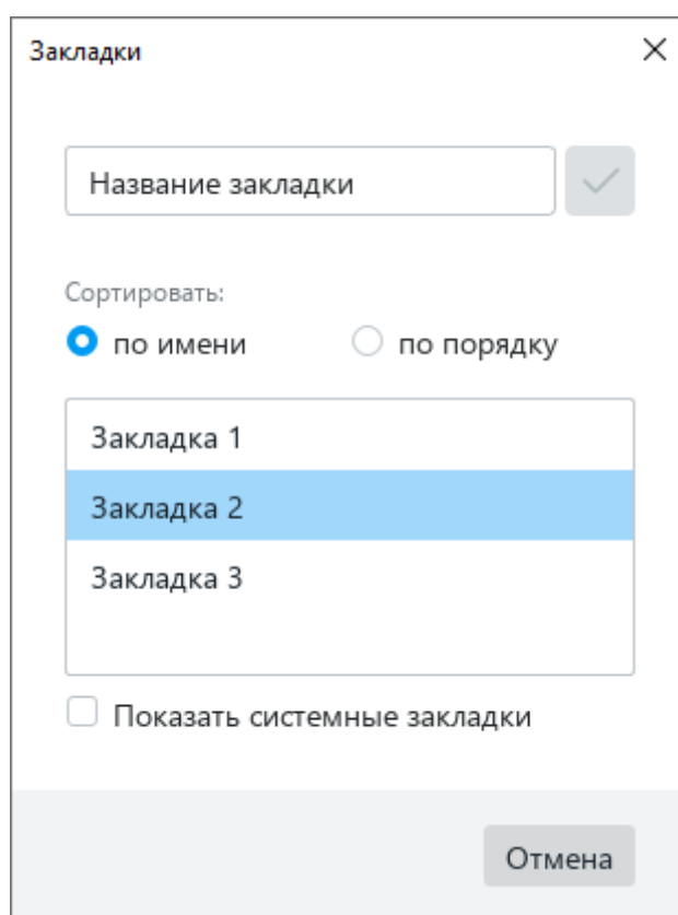
Рисунок 87 – Окно Закладки
