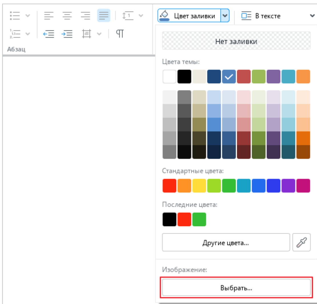
Рисунок 206 – Кнопка Выбрать
