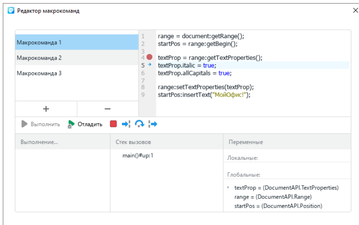
Рисунок 329 – Отладка макроккоманды
