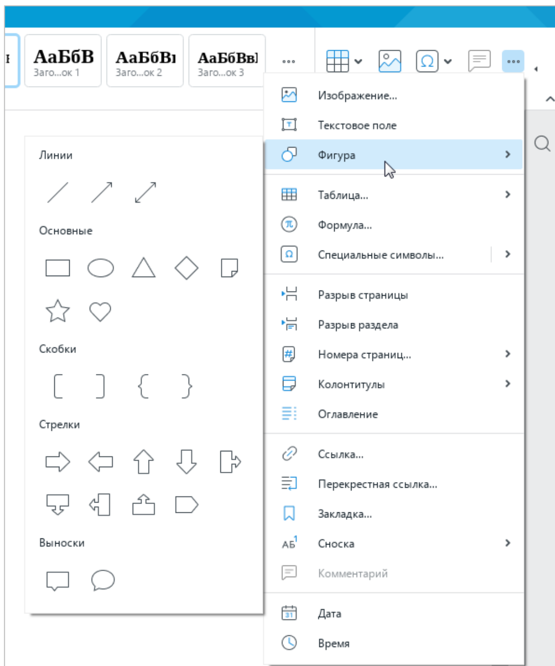
Рисунок 201 – Панель вставки
