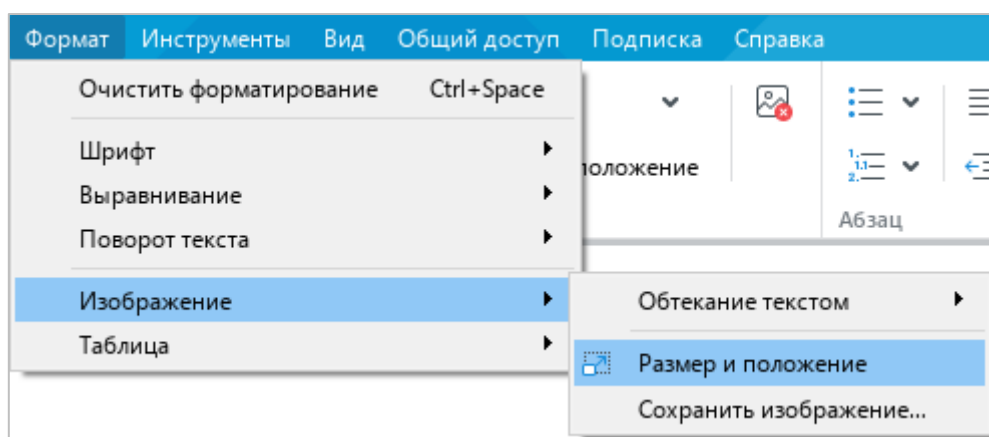
Рисунок 186 – Подменю Изображение
