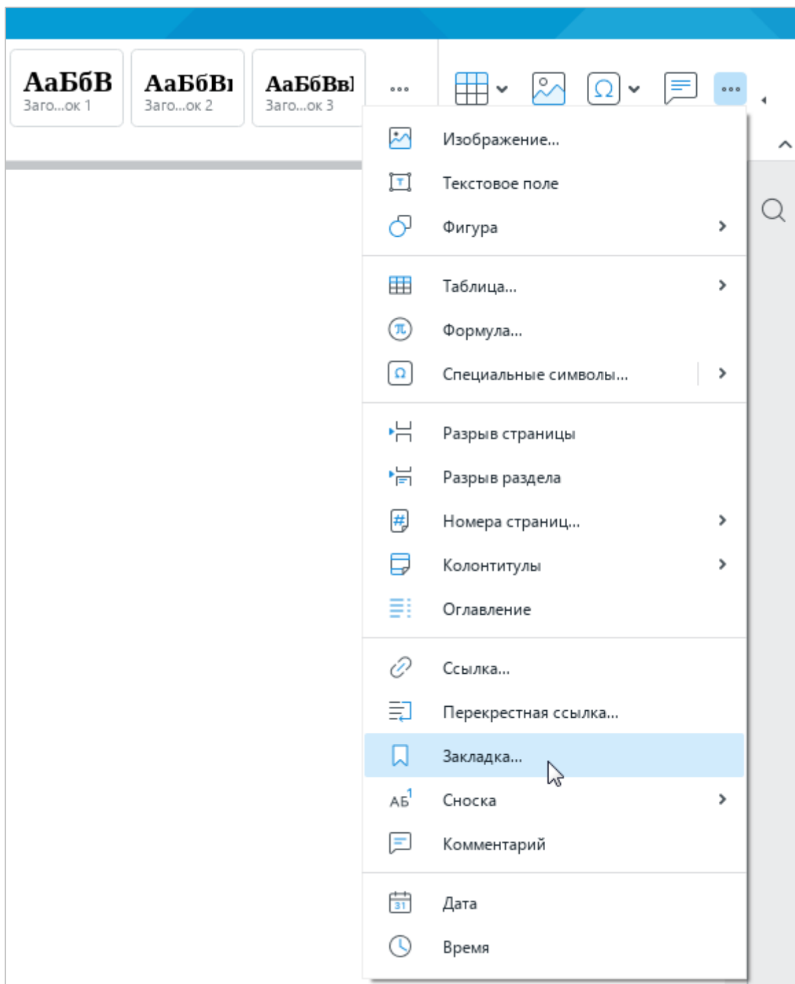
Рисунок 82 – Панель вставки
