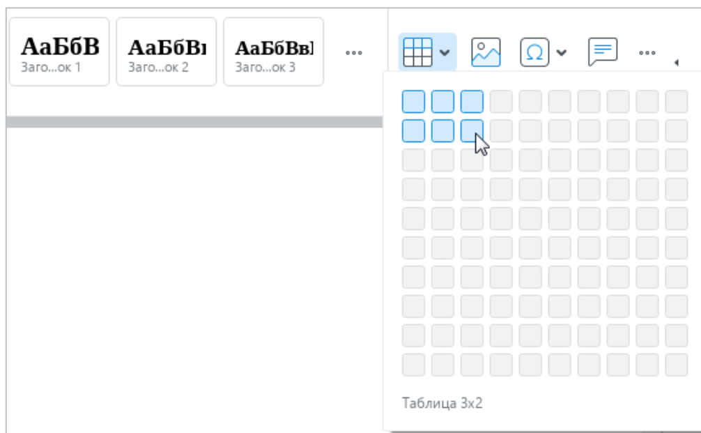
Рисунок 148 – Кнопка Таблица
