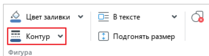
Рисунок 210 – Кнопка Контур
