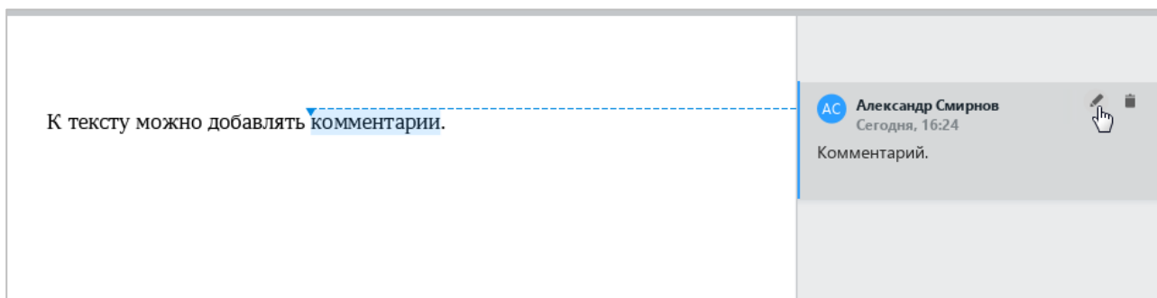
Рисунок 303 – Кнопка Редактировать
