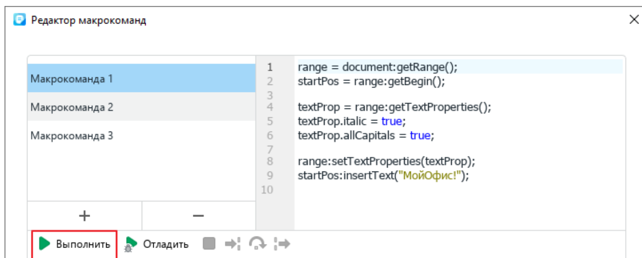
Рисунок 322 – Кнопка Выполнить
