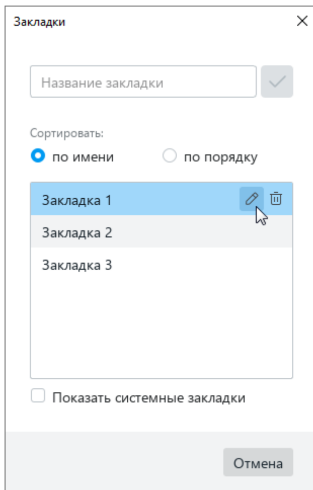
Рисунок 88 – Переименование закладки
