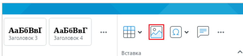
Рисунок 181 – Кнопка Изображение
