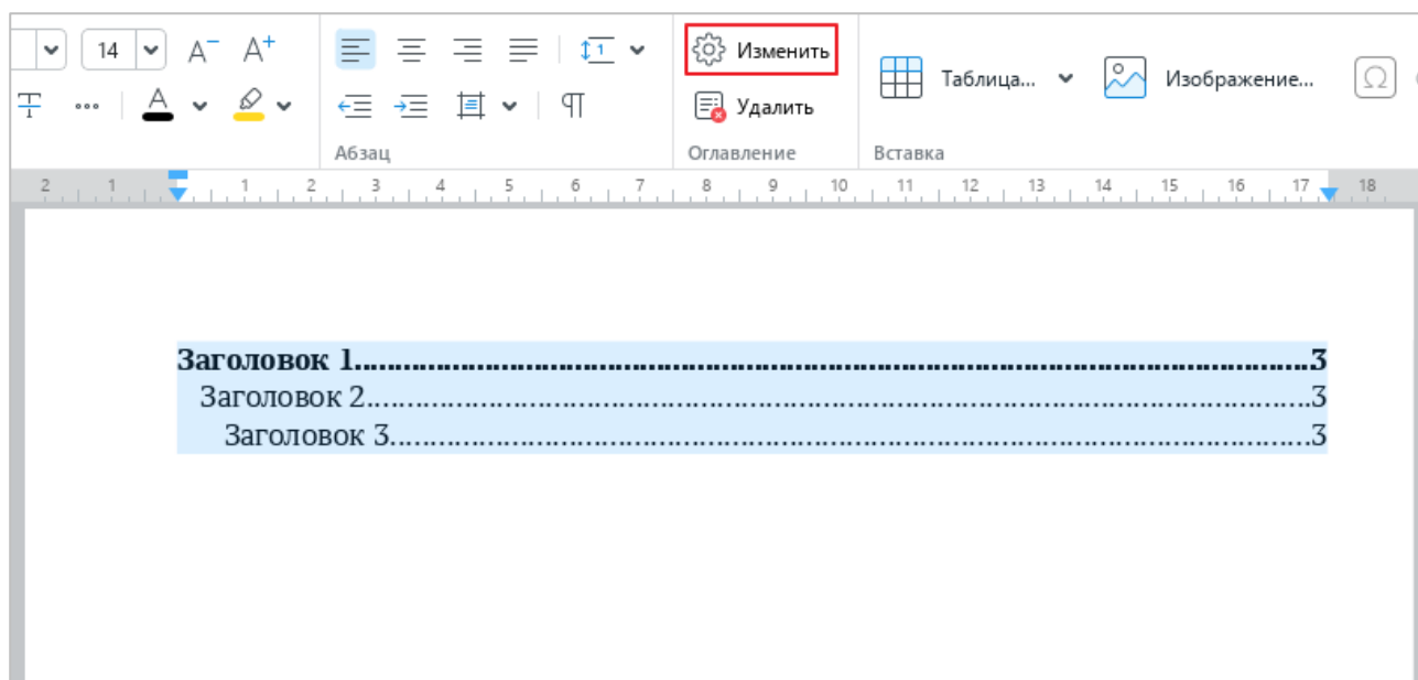
Рисунок 265 – Кнопка Изменить
