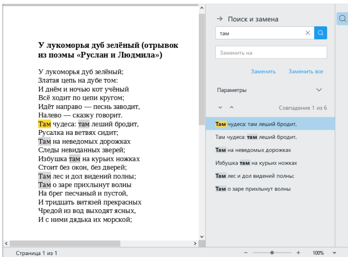
Рисунок 109 – Найденные совпадения
