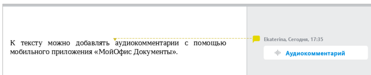
Рисунок 311 – Аудиокомментарий
