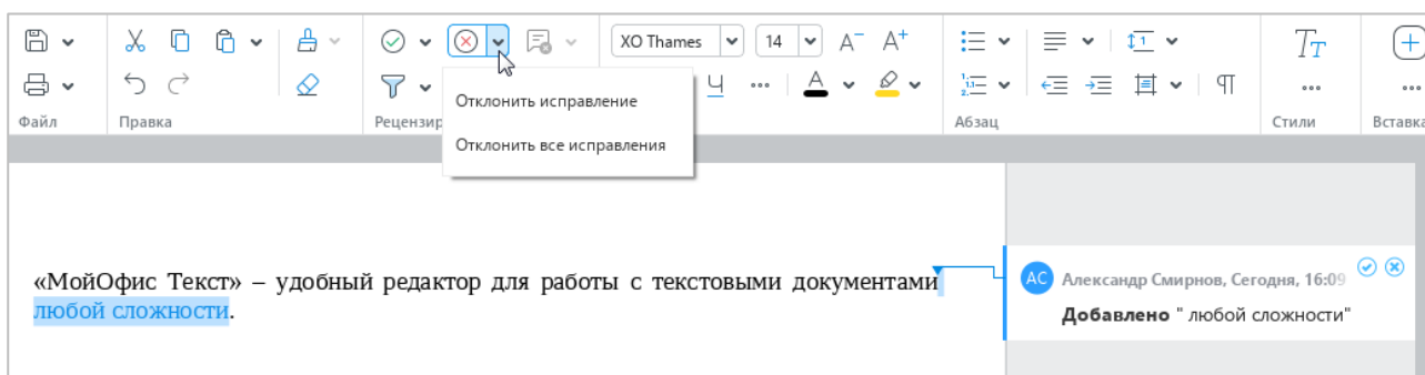
Рисунок 287 – Отклонение исправлений
