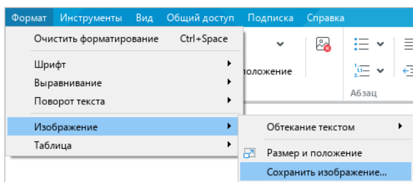
Рисунок 198 – Подменю Изображение
