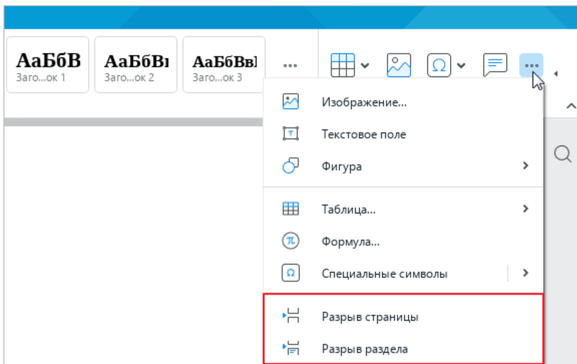
Рисунок 260 – Панель вставки
