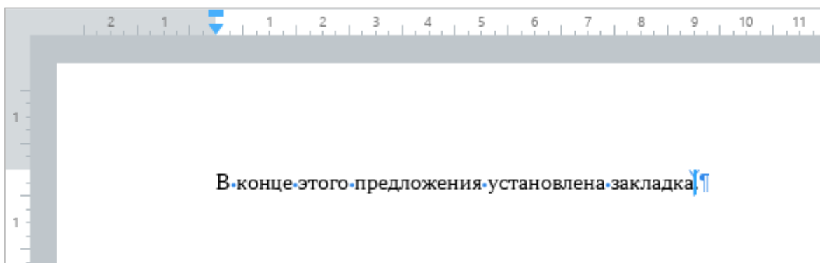
Рисунок 85 – Отображение закладки
