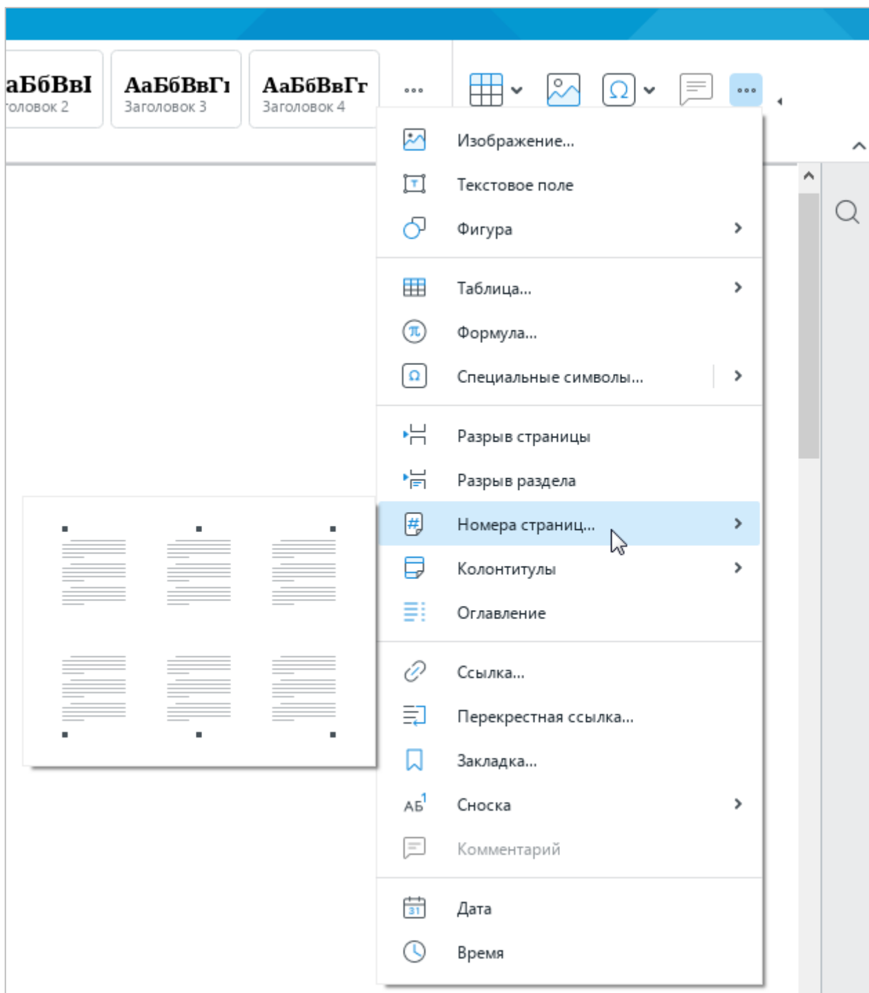
Рисунок 250 – Панель вставки
