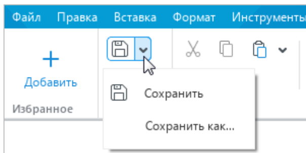
Рисунок 54 – Кнопка Сохранить
