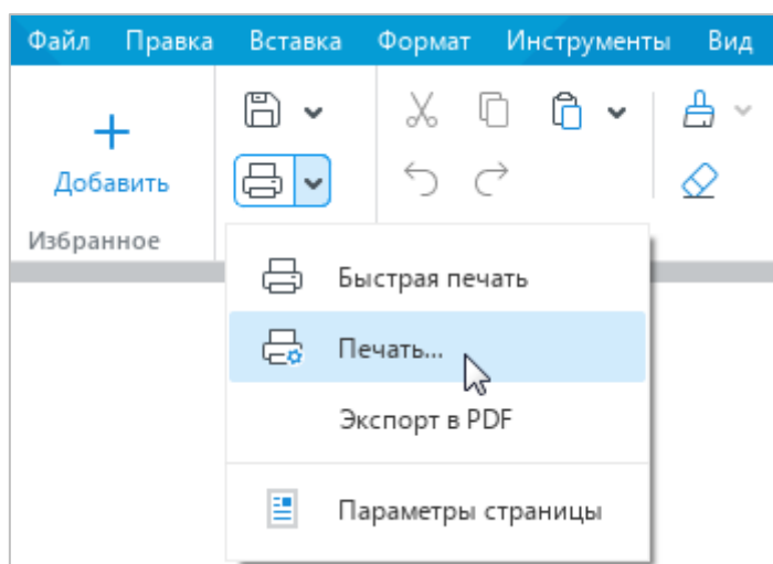
Рисунок 50 – Команда Печать
