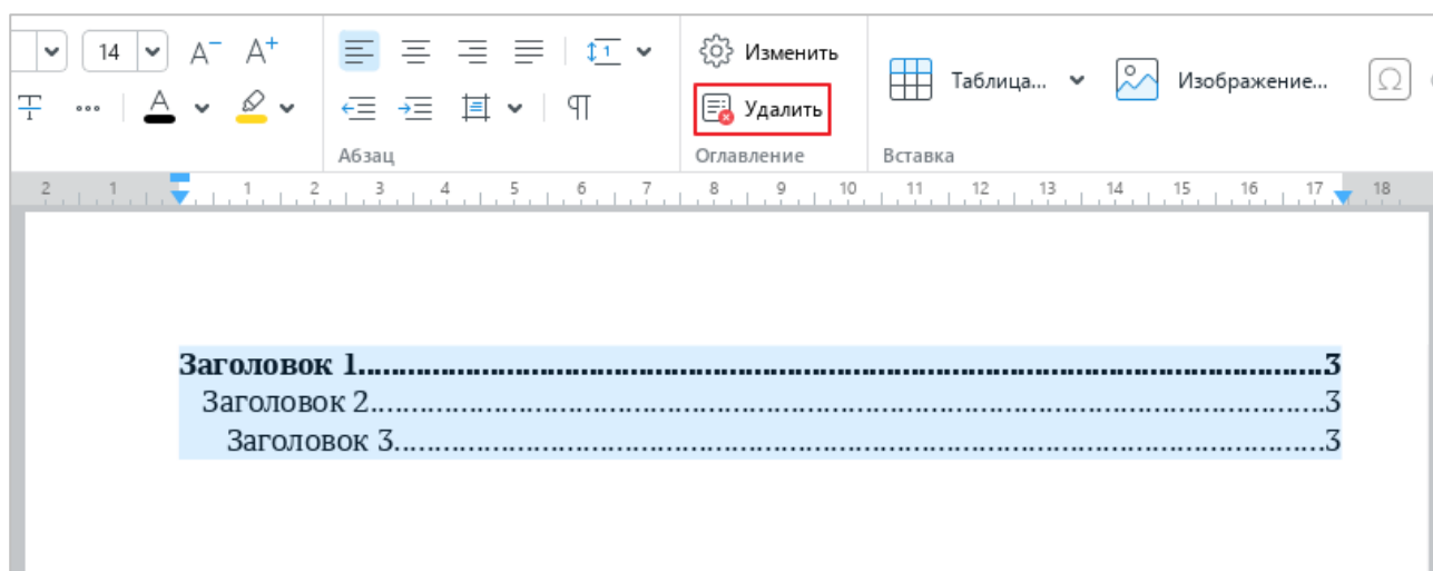
Рисунок 271 – Кнопка Удалить
