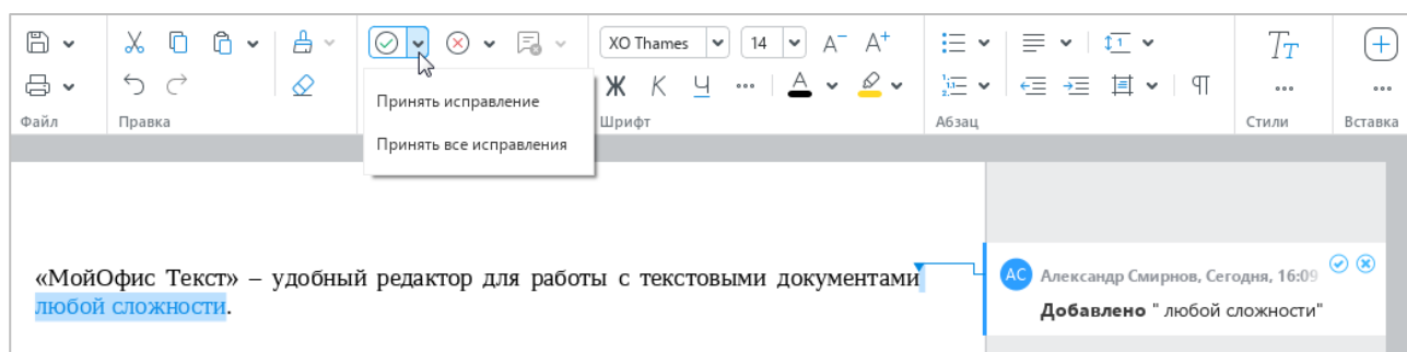
Рисунок 286 – Принятие исправлений
