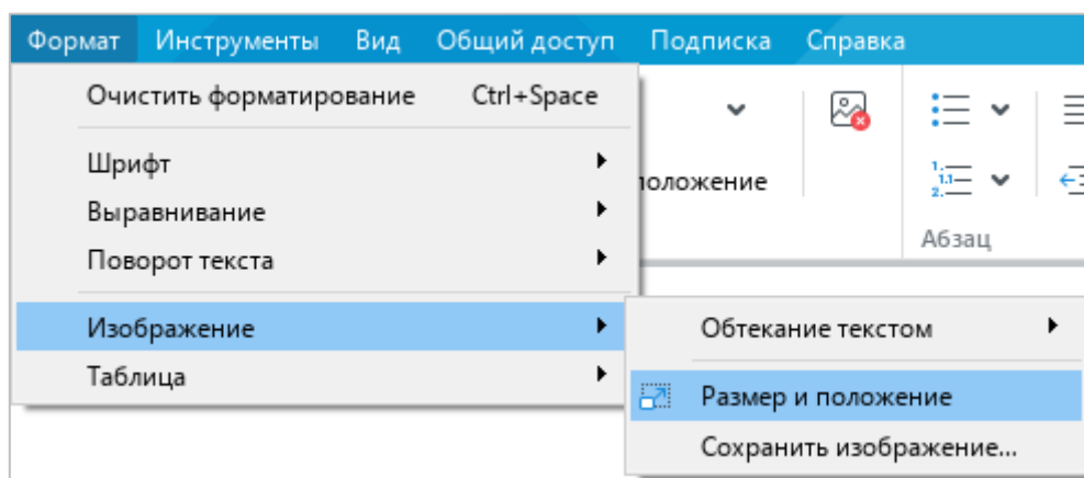
Рисунок 190 – Подменю Изображение
