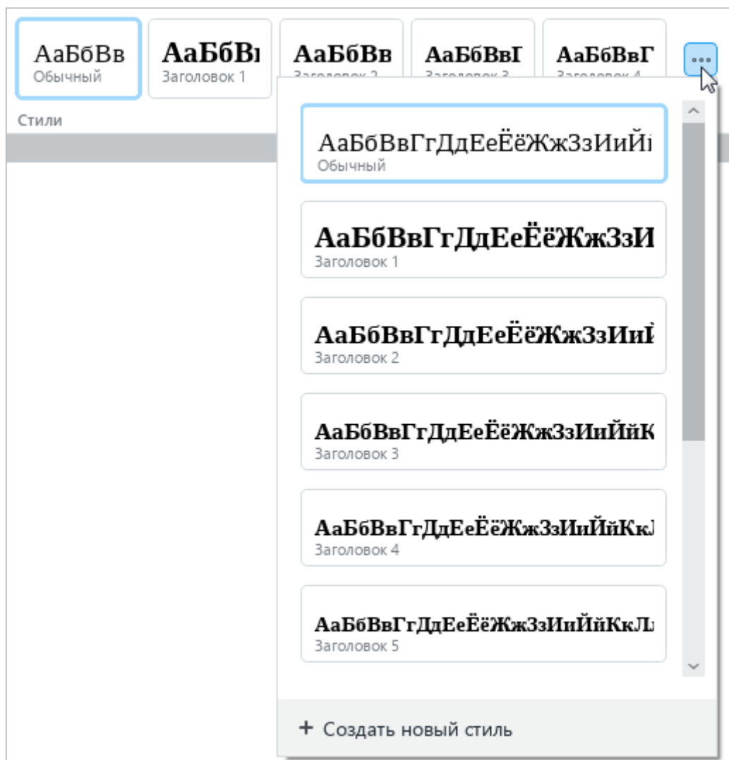
Рисунок 112 – Список стилей
