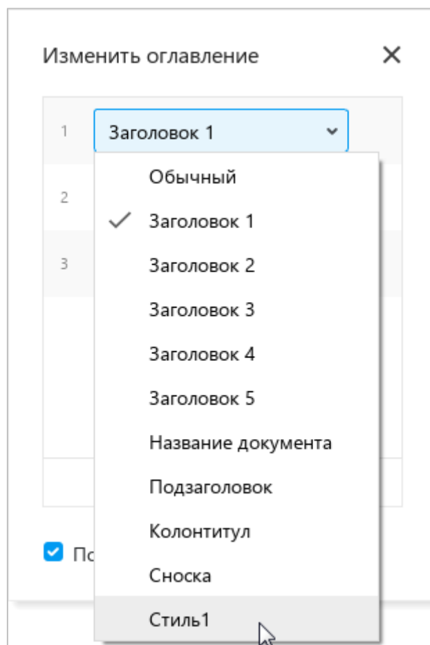
Рисунок 269 – Выбор стиля
