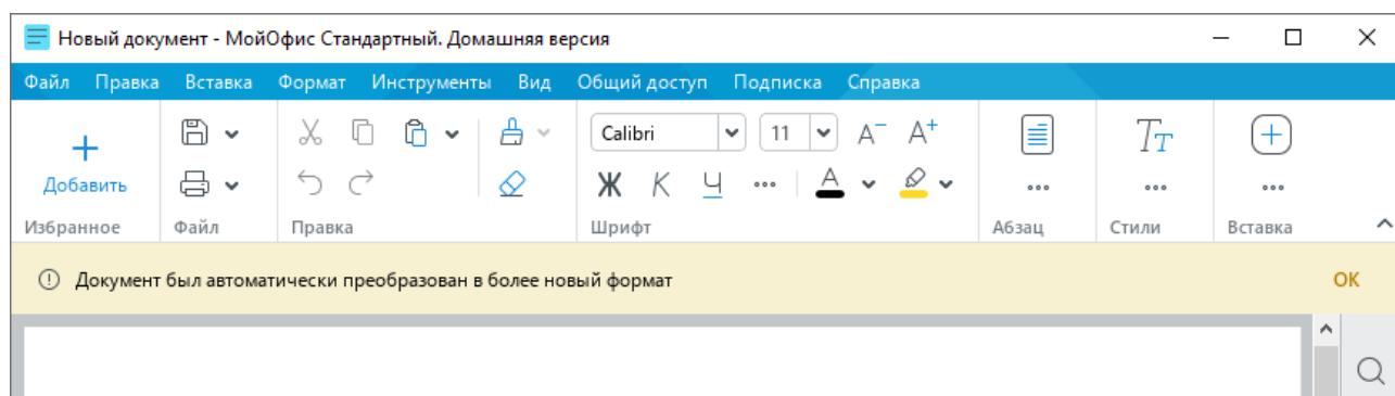
Рисунок 41 – Кнопка Заккрыть
