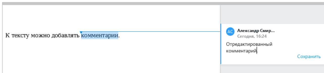
Рисунок 304 – Поле комментария
